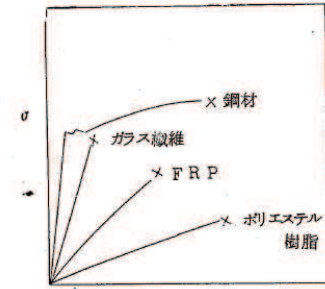
応力-ひずみ関係 (「FRP成形入門講座(日本プラスチック加工技術協会)」)
