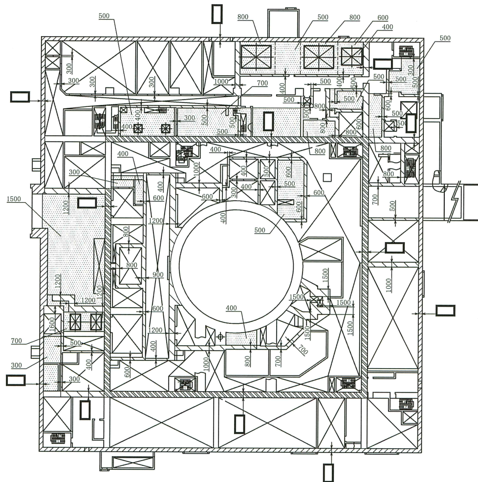
原子炉建屋 O.P. 18.30m
