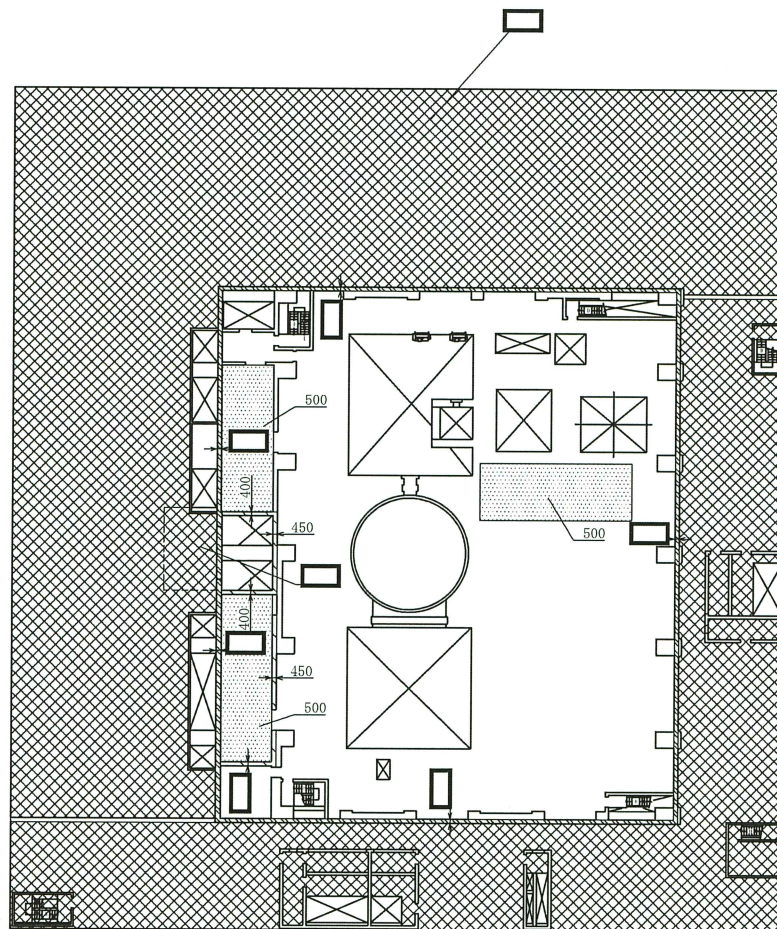
原子炉建屋 O.P. 33. 20m
