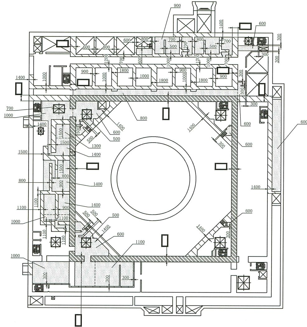
原子炉建屋 0.P.-0.80m
