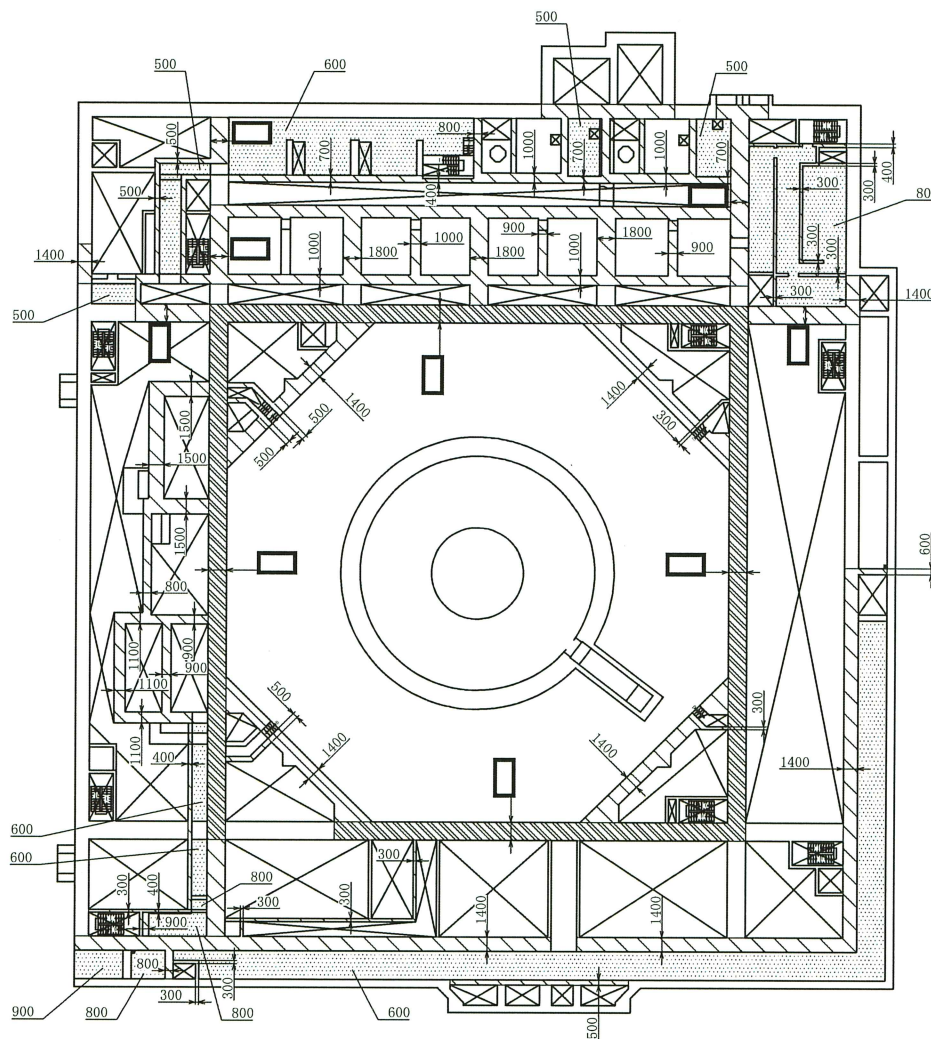
原子炉建屋 O.P. 1.10m
