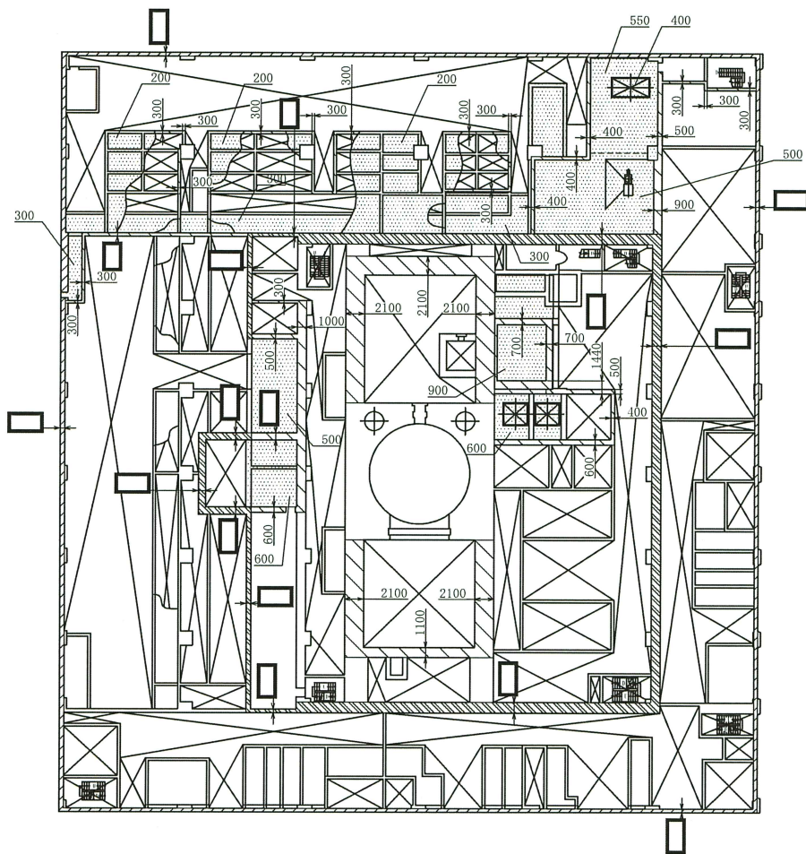
原子炉建屋 0.P. 28.50m
