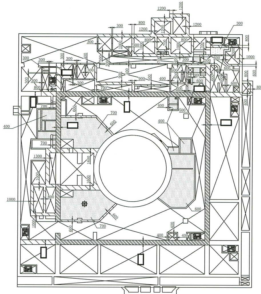
原子炉建屋 O.P. 11.50m
