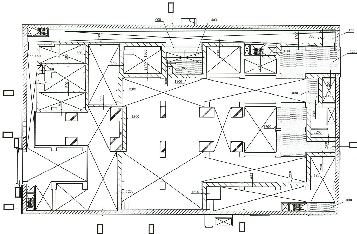
タービン建屋 0. P. 17. 00m
