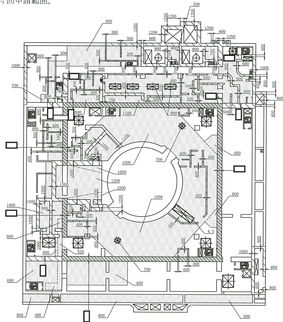
原子炉建屋 O.P. 6.00m
