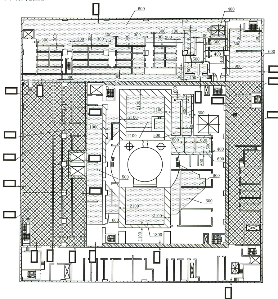
原子炉建屋 0.P. 22. 50m
