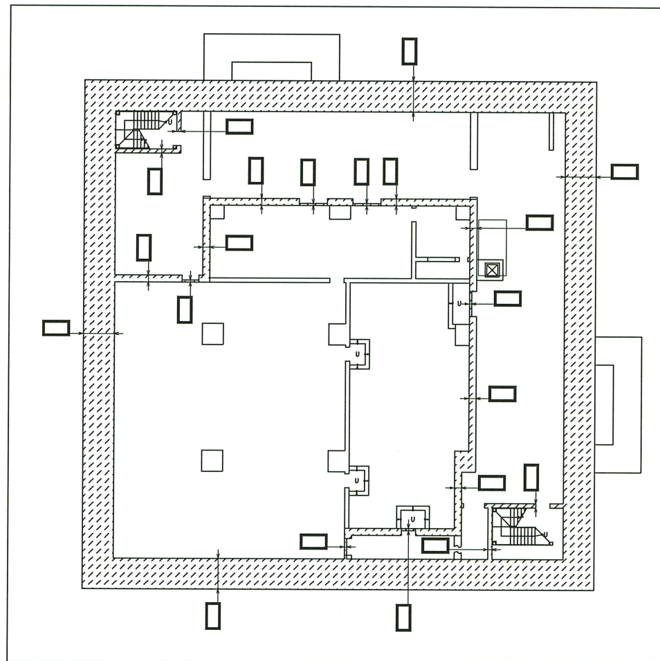
緊急時対策建屋 0.P. 51. 50m
