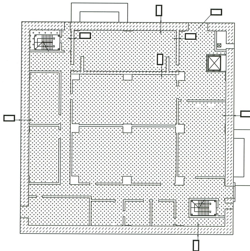
緊急時対策建屋 O.P. 62. 20m
