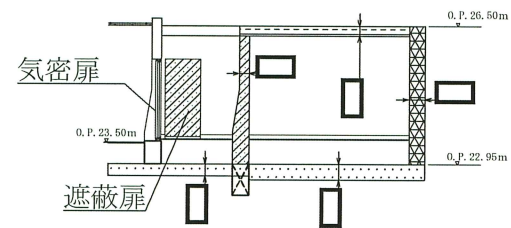
A～A断面図
