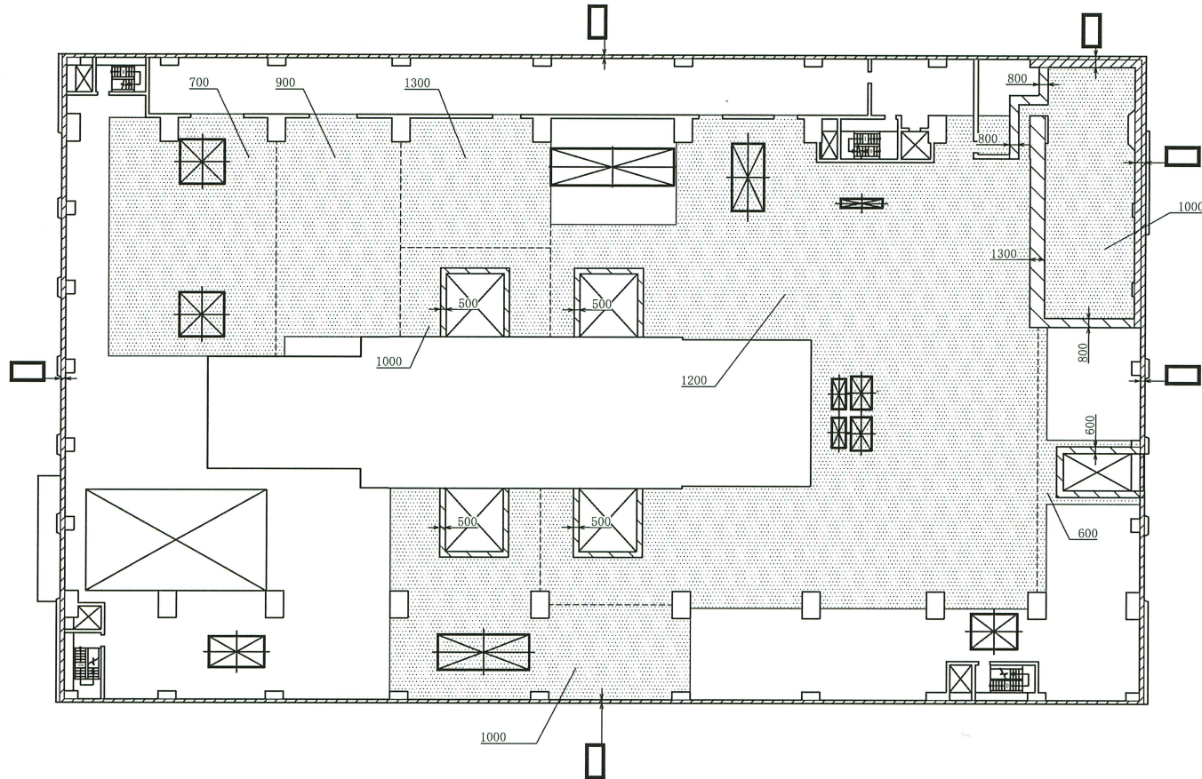
タービン建屋 O.P. 24.80m
