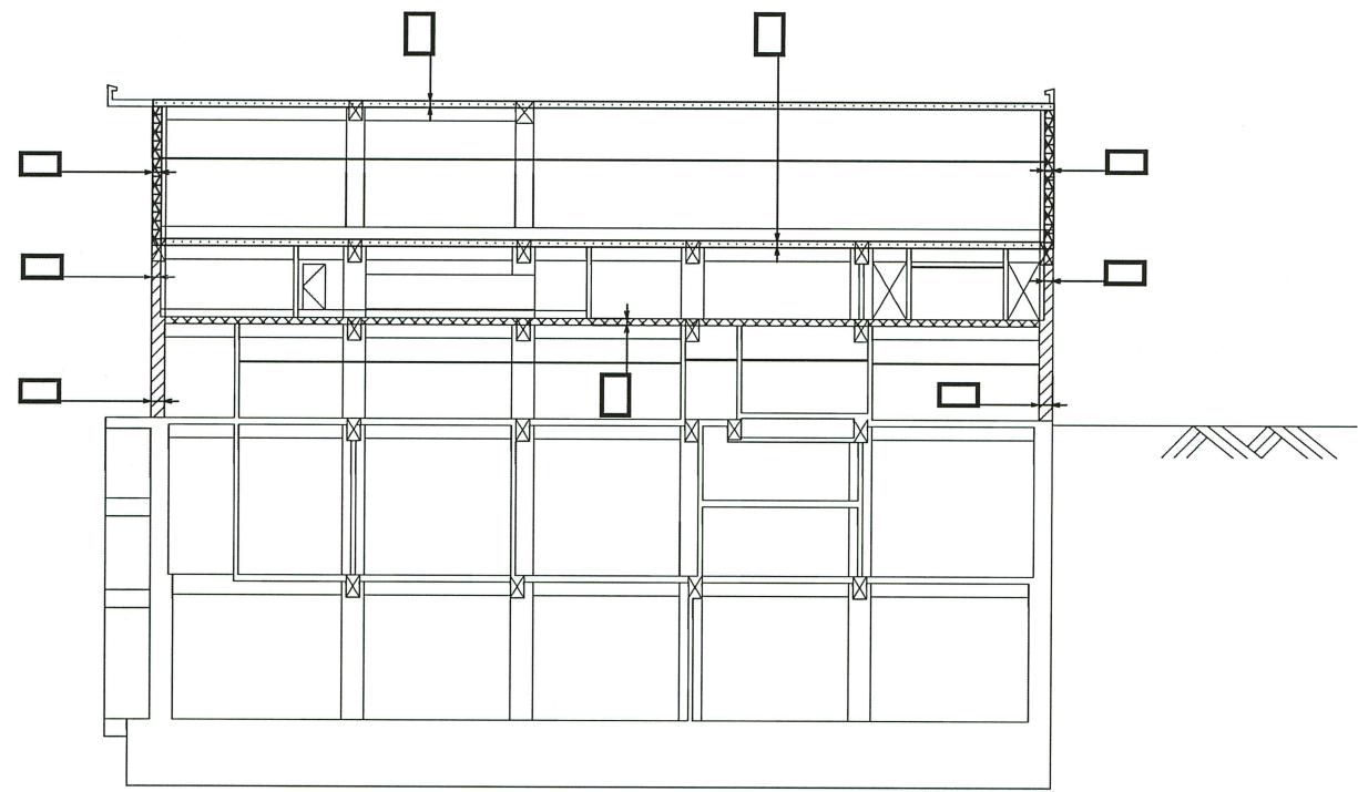
制御建屋 A-A断面
