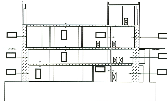
B-B断面図
