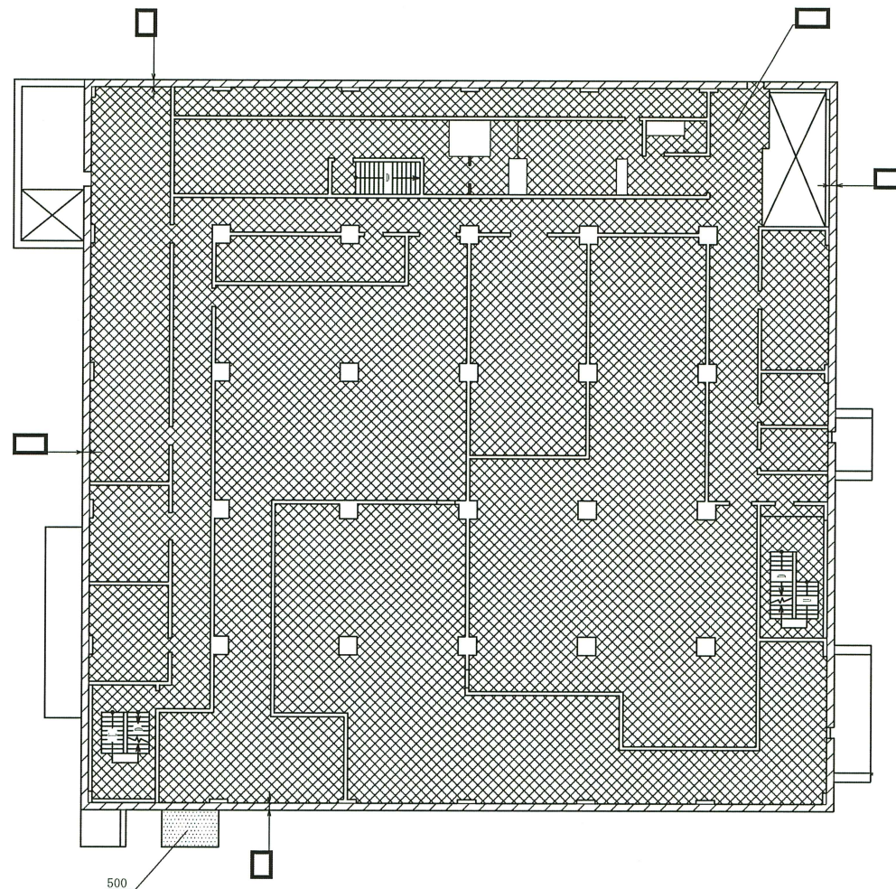
制御建屋 O.P. 19.50m
