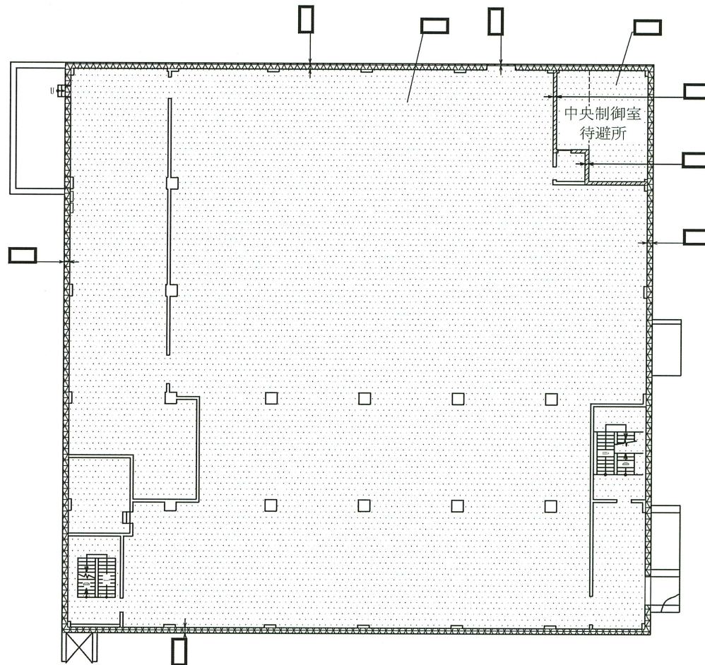
制御建屋 0.P. 23.50m
