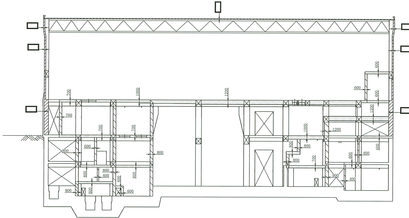
タービン建屋 A-A断面
