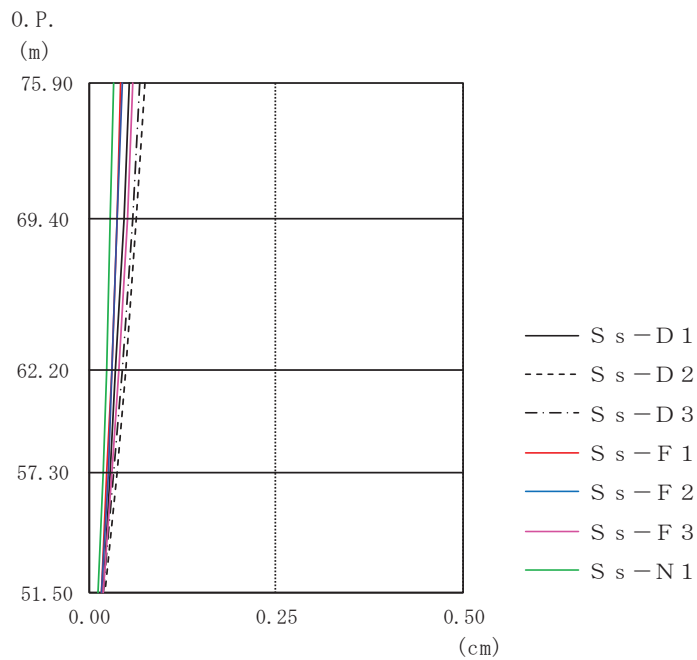
图 4-11 最大応答変位 (基準地震動 S_s , UD 方向)
