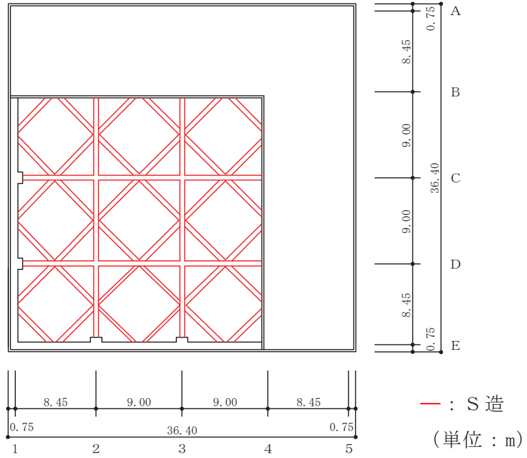
図 2-2(5) 緊急時対策建屋の概略平面図 (O.P. 75.9m)
