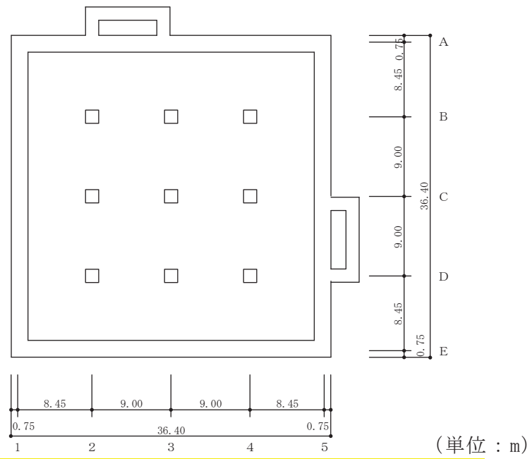
図 2-2(2) 緊急時対策建屋の概略平面図 (O.P. 57.3m)
