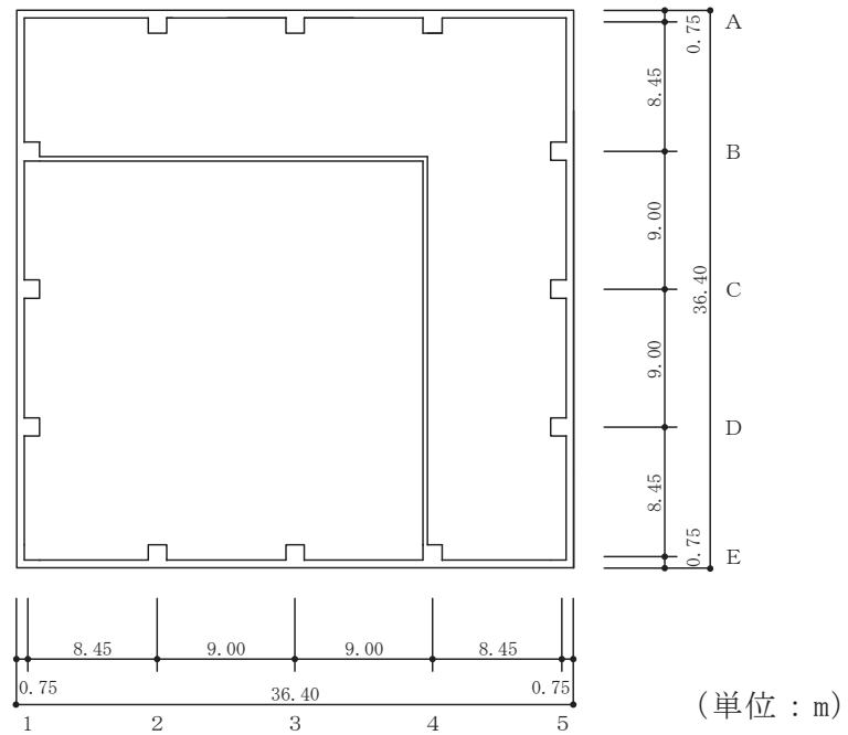
図 2-2(4) 緊急時対策建屋の概略平面図 (O.P. 69.4m)
