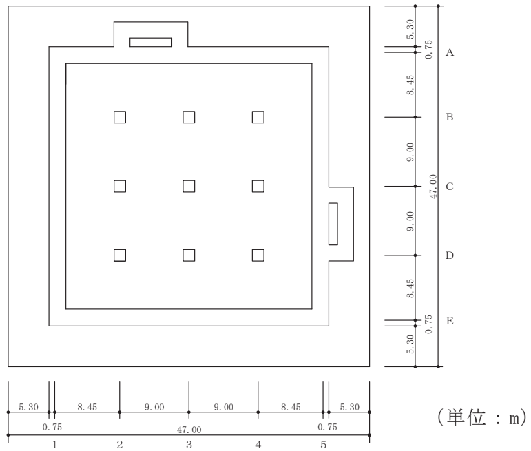
図 2-2(1) 緊急時対策建屋の概略平面図 (O.P. 51.5m)
