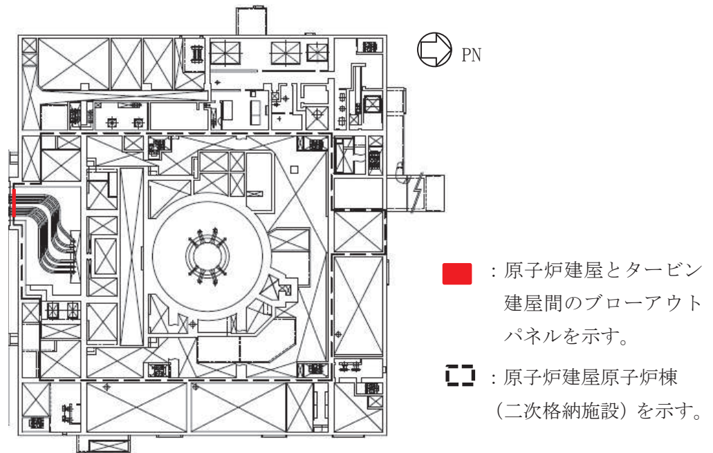
図 1-1 原子炉建屋内側ブローアウトパネル配置図 (3/3)
