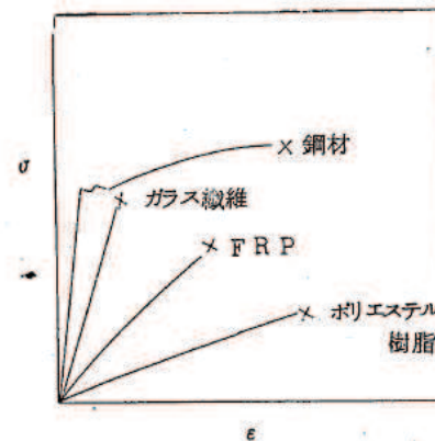
応力-ひずみ曲線
