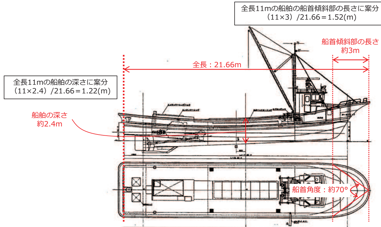
図-1 一般配置図(FRP漁船)
