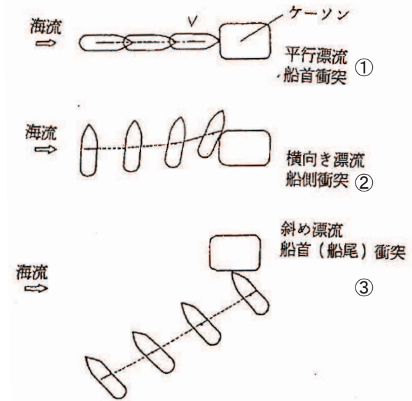
図 漂流による衝突形態(「土木学会(1994)」に一部加筆)
