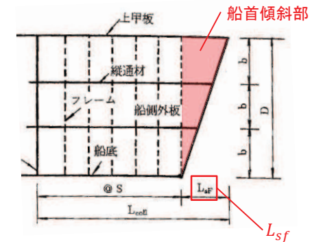
船首部の標準型 (「土木学会(1994)」に一部加筆)
