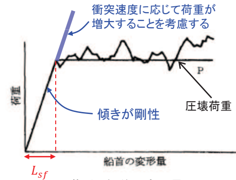
荷重と船首の変形量 (「土木学会(1994)」に一部加筆)
