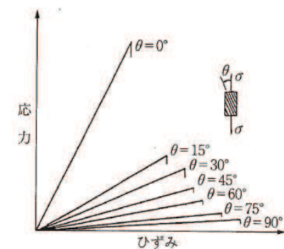
応力-ひずみ曲線
