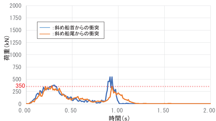
衝突荷重の時刻歴(斜め船首, 斜め船尾)
