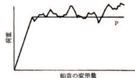
荷重と船首の変形量(「土木学会(1994)」)
