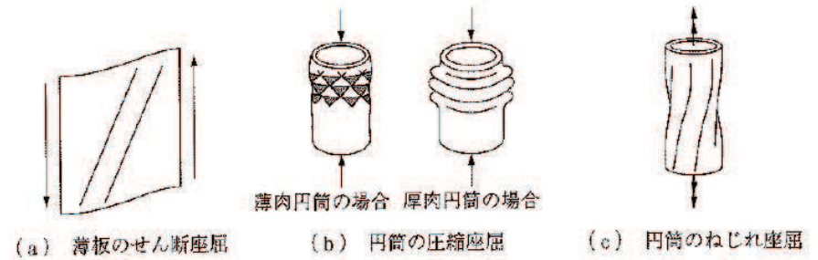
座屈変形の例
