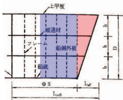
図 3.3 船首部の標準型
