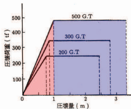
図 3.6 圧壊荷重と圧縮量
