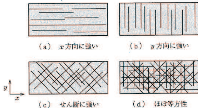
FRPの材料異方性
