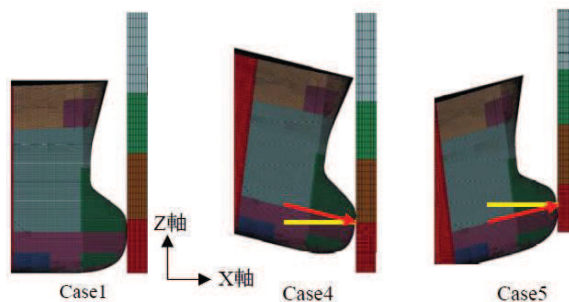
図3 解析ケース(被衝突体は鋼製主塔)
