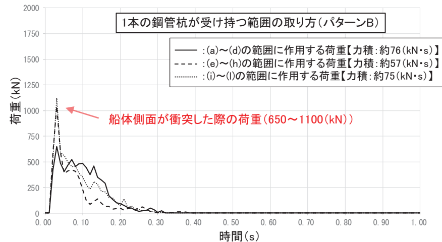
1本の鋼管杭が受け持つ範囲の取り方(パターンB)
