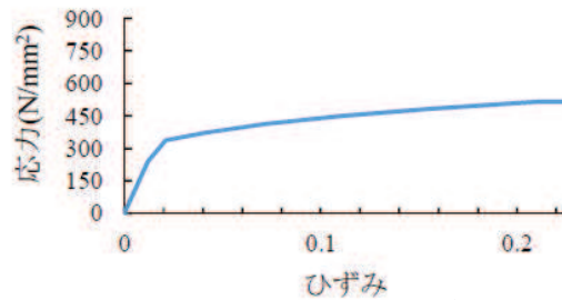
図2 船舶の鋼材の応力-ひずみ関係
