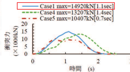
図4 衝突力の時刻歴
