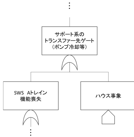
図 1 ハウス事象の設置のイメージ (SWS A トレインの例)
