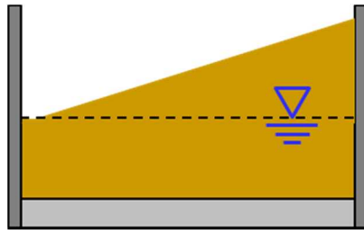
図-2 液状化試験の模型断面のイメージ（傾斜あり地盤）
