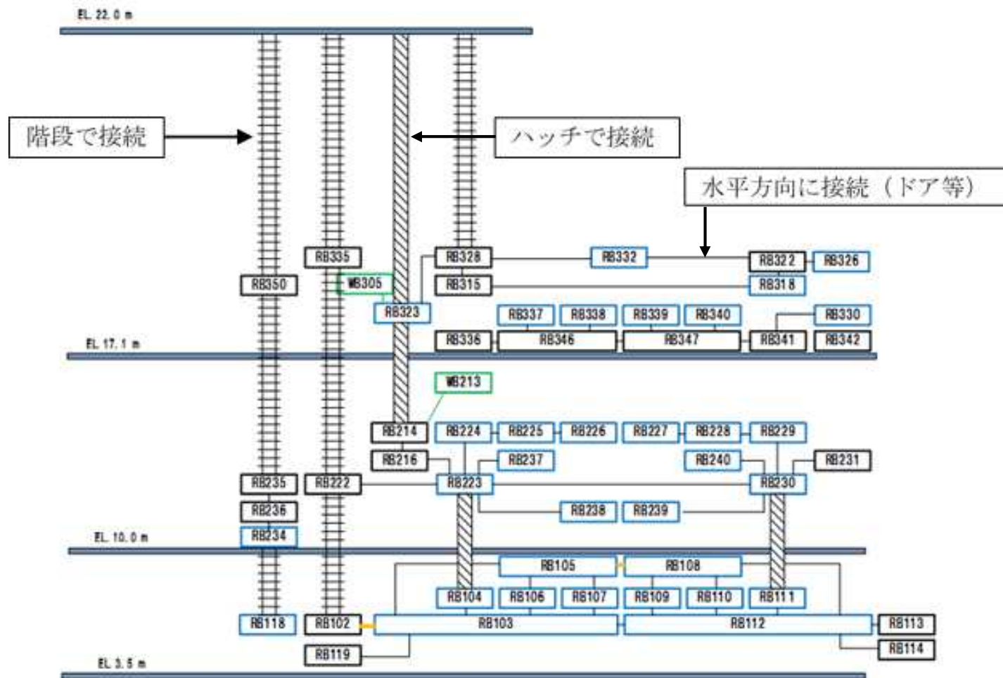
図2 浸水解析ツールのモデルの階層概念図
