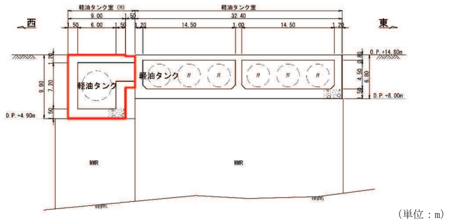
図 2-5(2) 軽油タンク室 (H) 断面図 (B-B 断面, 東西)
