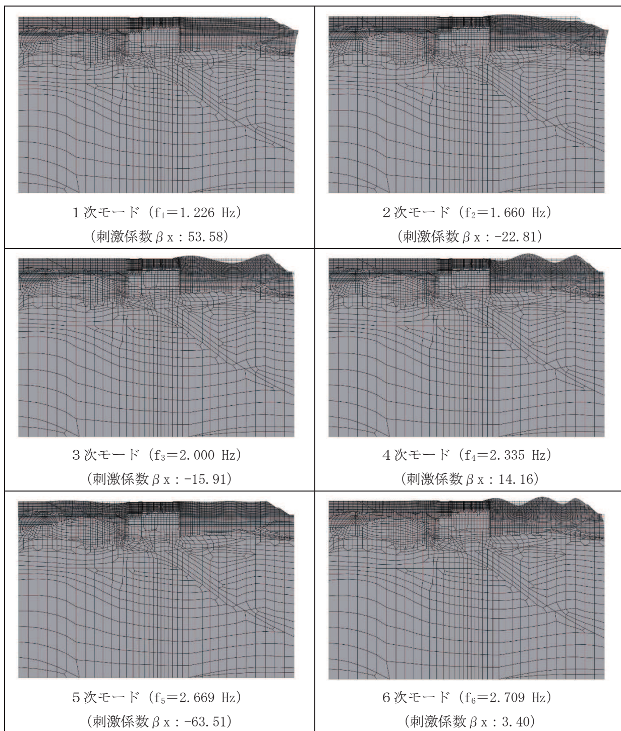
図 3-21(1) 固有値解析結果 (モード図) (C-C 断面, 東西(ポンプ室)) (1/2)
