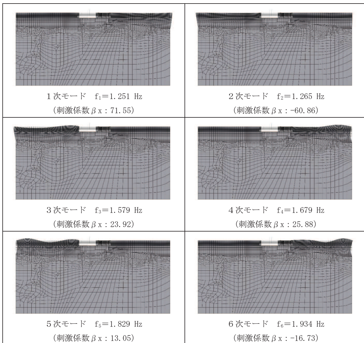
図 3-19(1) 固有値解析結果 (モード図) (A-A 断面, 南北) (1/2)
