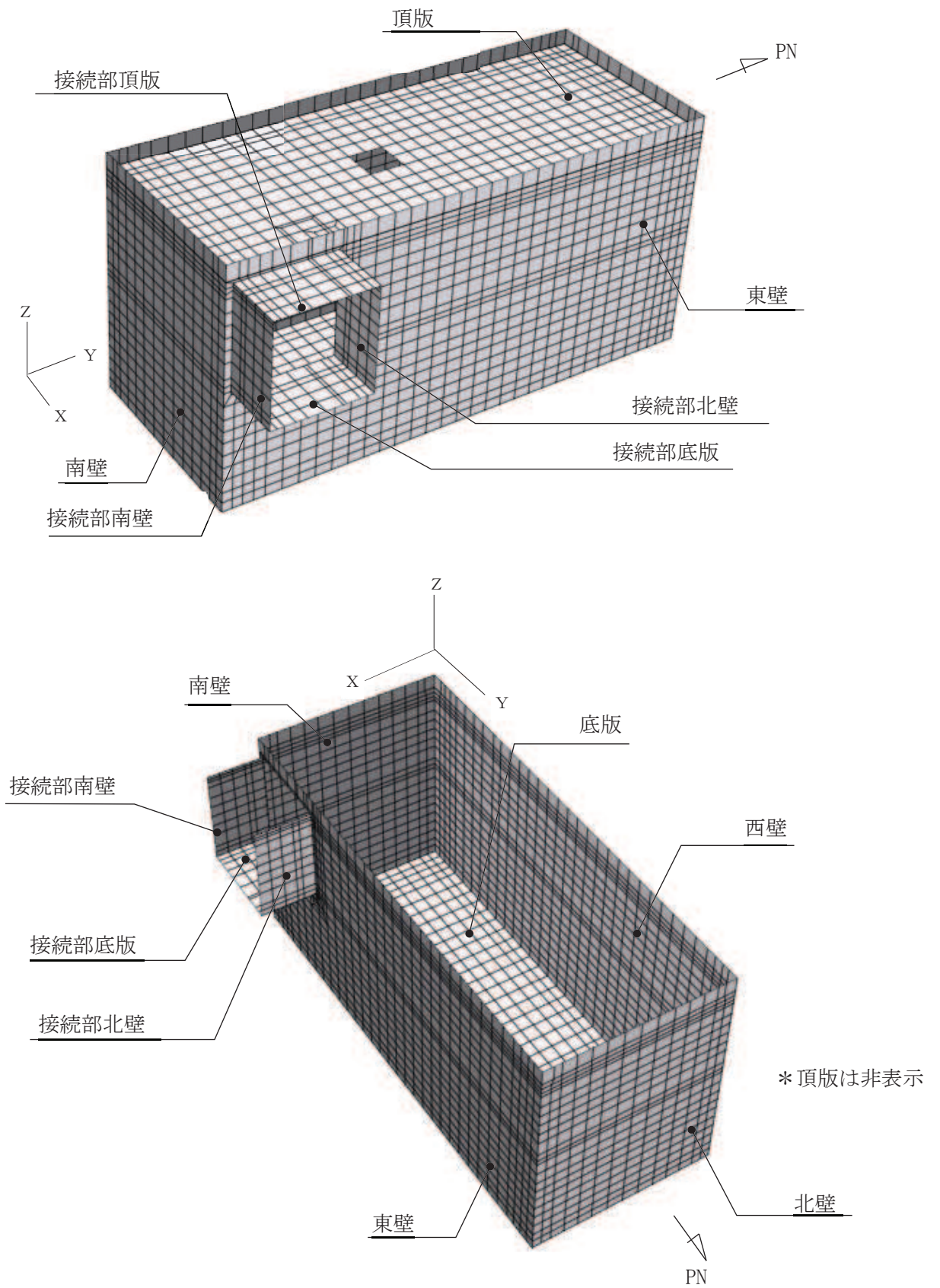
図 4-1 三次元構造解析モデルの概念図
