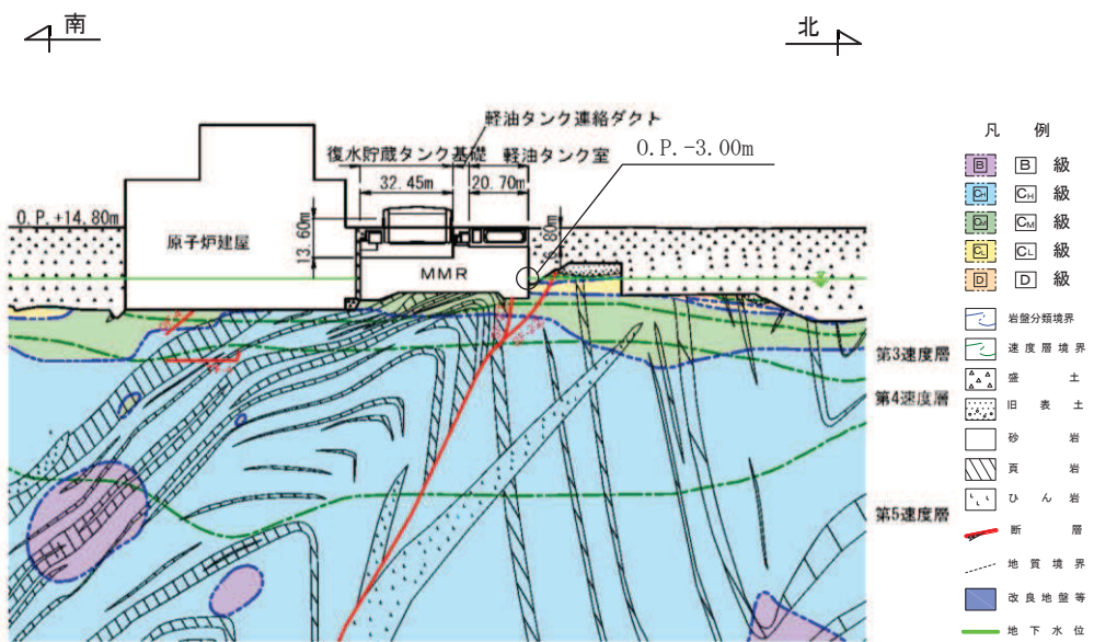
図 2-7(1) 軽油タンク室 地震時荷重算出用地質断面図 (A-A 断面, 南北)
