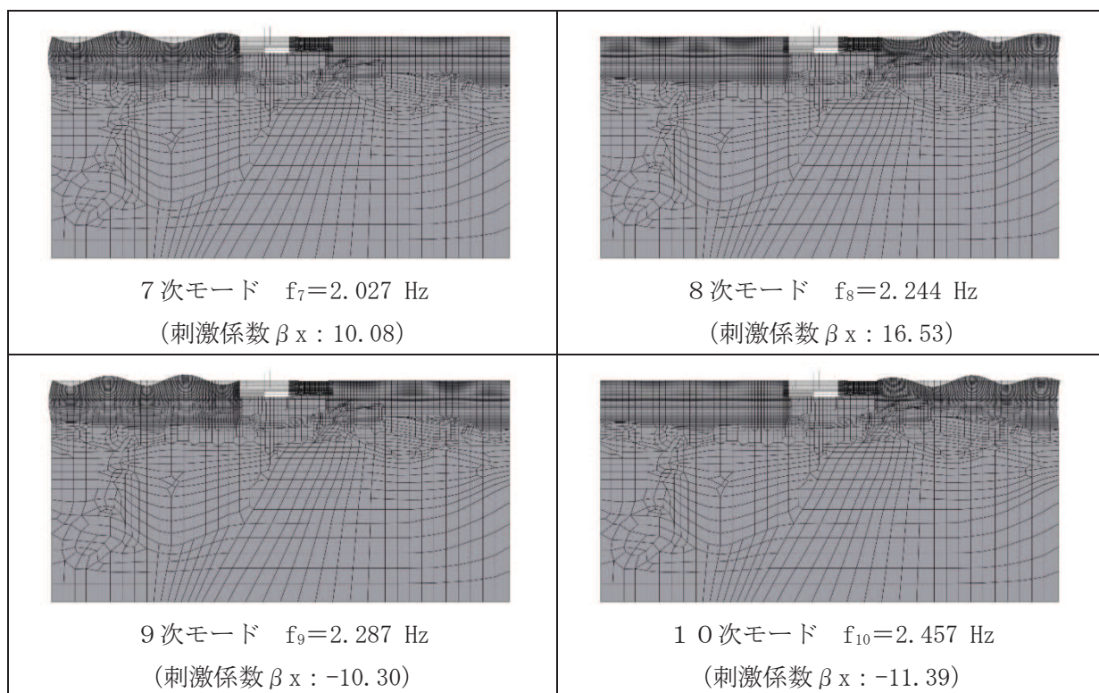
図 3-19(2) 固有値解析結果 (モード図) (A-A 断面, 南北) (2/2)
