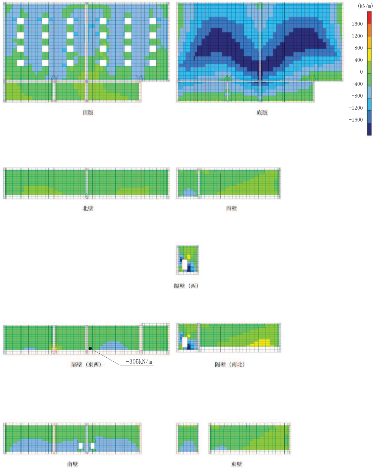
図 6-10(4) せん断破壊に対する照査値最大時の断面力分布図 (軸力 (kN/m) : N_y ) (隔壁 (東西), 解析ケース③, S_s - D 2 (++) , t = 25.09\text{s} )
