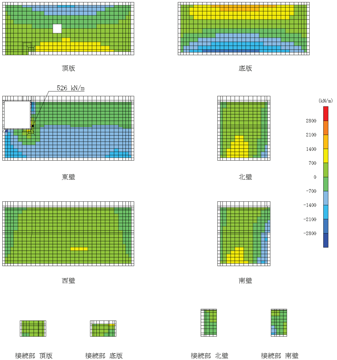
図 6-10 曲げ・軸力系の破壊に対する照査値最大時の断面力分布図 (軸力 (kN/m) : N_y ) (東壁, 解析ケース③, S_s - D 2 (++) , t = 8.58 s)
