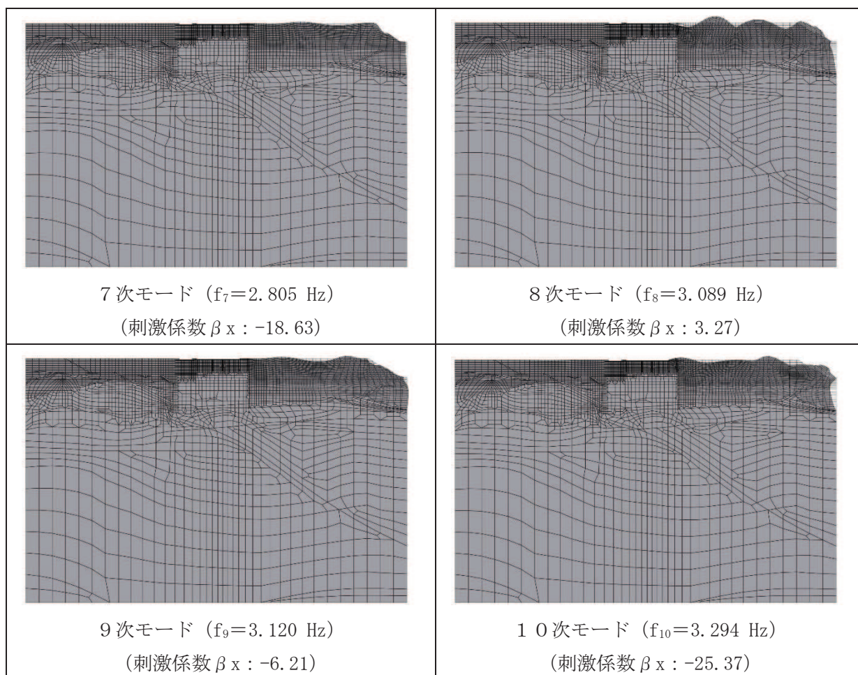
図 3-21(2) 固有値解析結果 (モード図) (C-C 断面, 東西(ポンプ室)) (2/2)
