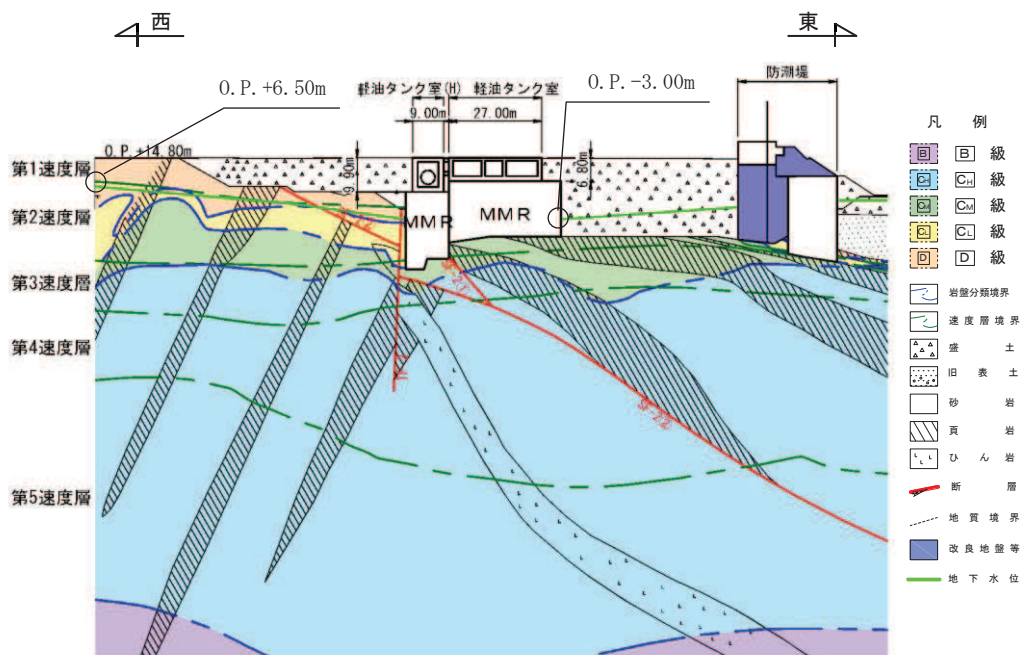
図 2-9(3) 設計用地下水位 (C-C 断面, 東西 (ポンプ室))
