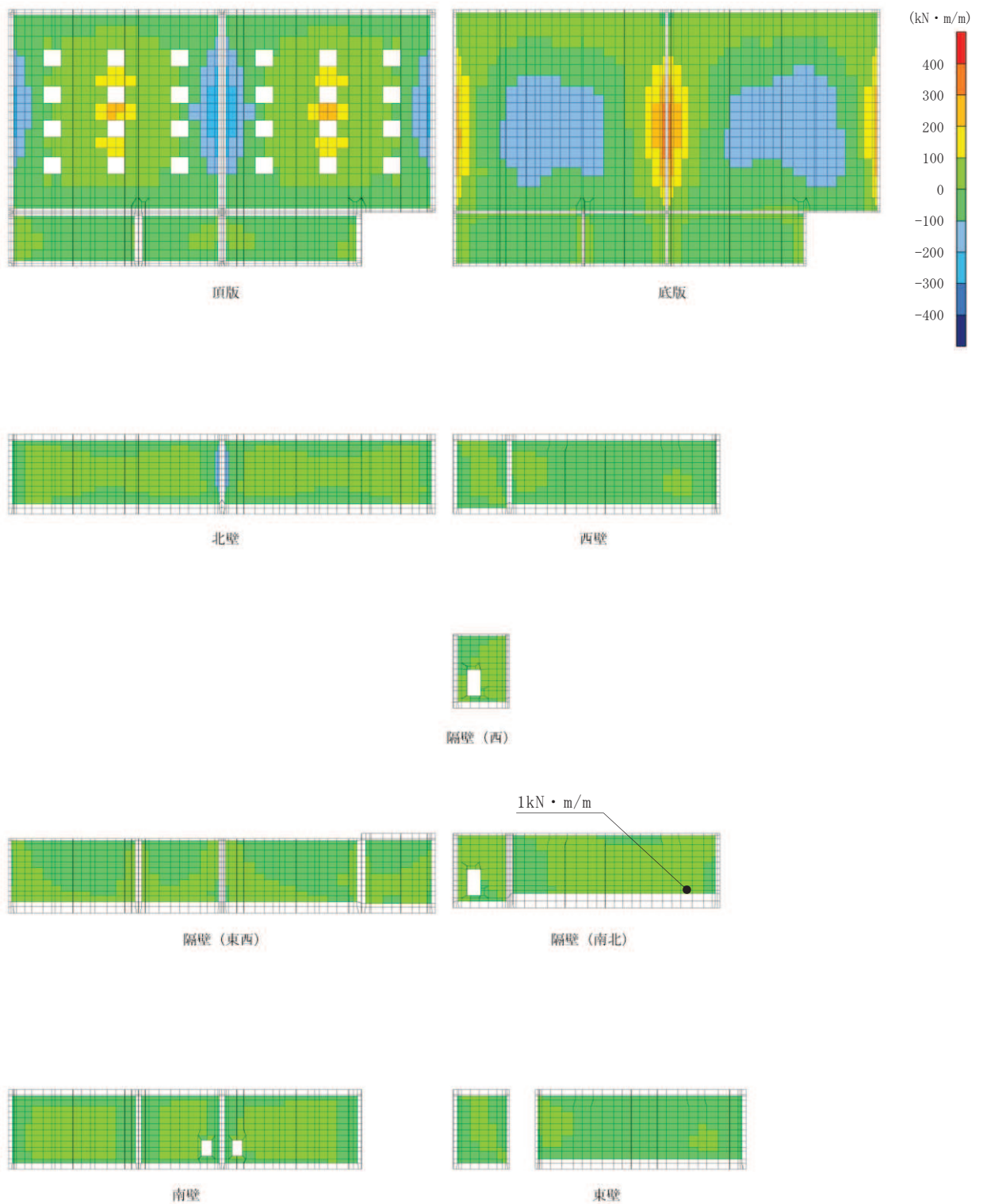
図 10-1 静的地震力載荷時の断面力分布図 (曲げモーメント ( \text{kN} \cdot \text{m}/\text{m} ) : M_x )
