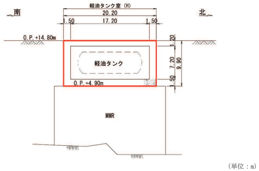
図 2-5(1) 軽油タンク室 (H) 断面図 (A-A 断面, 南北)
