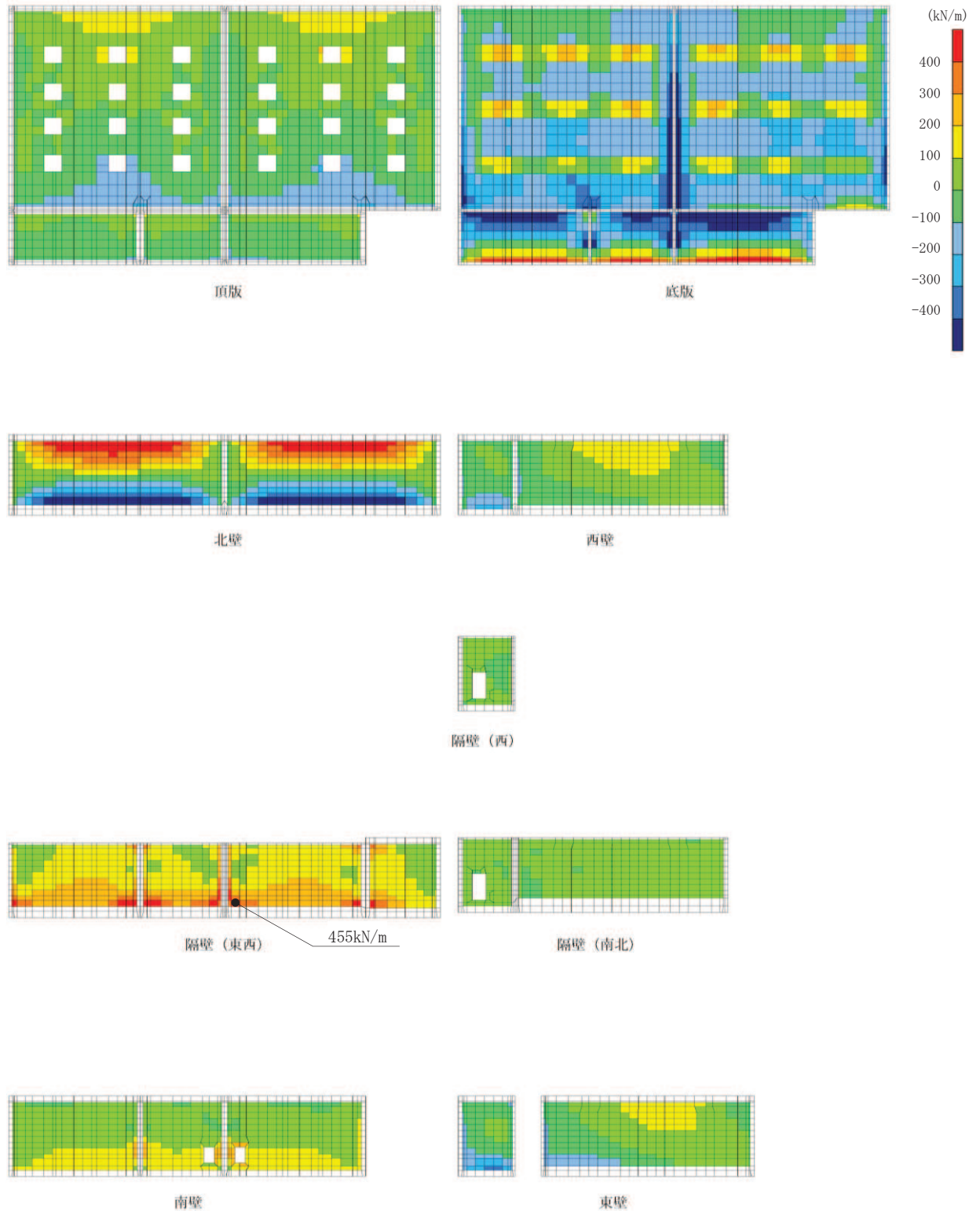
図 6-10(6) せん断破壊に対する照査値最大時の断面力分布図 (せん断力 (kN/m) : Q_y ) (隔壁 (東西), 解析ケース③, S_s - D_2 (++) , t = 25.09s )
