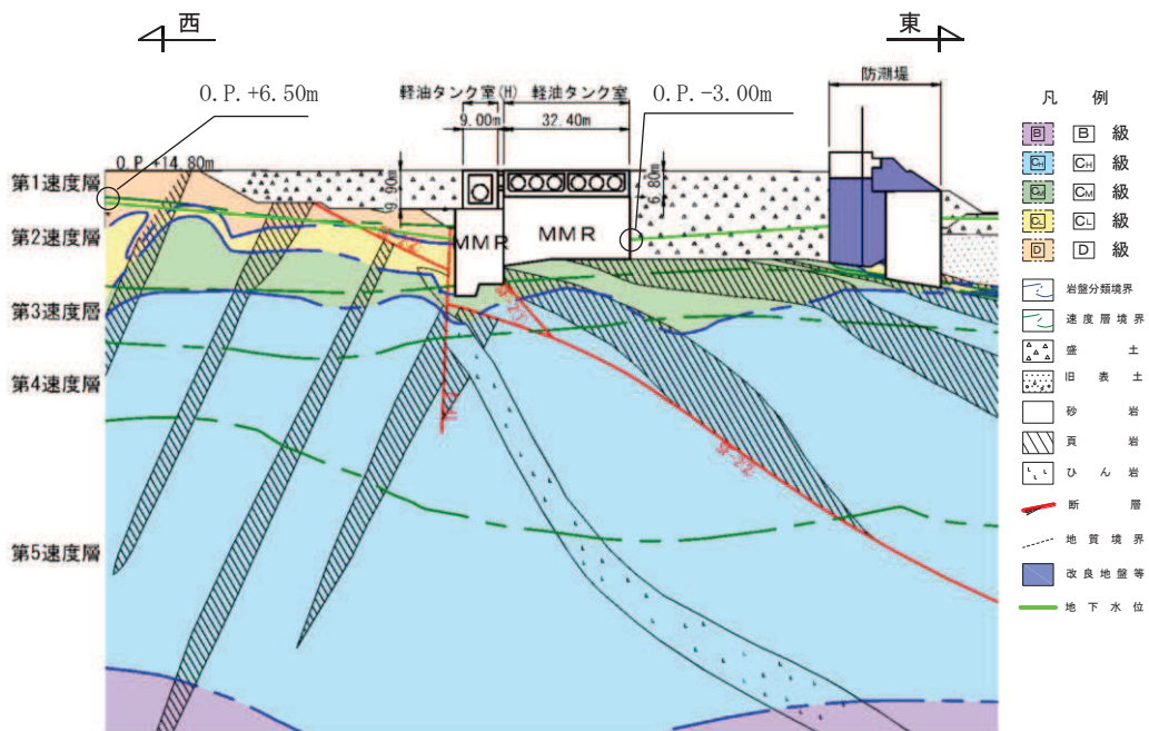
図 2-7(2) 軽油タンク室 地震時荷重算出用地質断面図 (B-B 断面, 東西 (タンク室))
