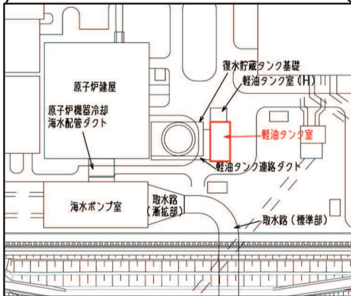
図 2-3 軽油タンク室の位置図
