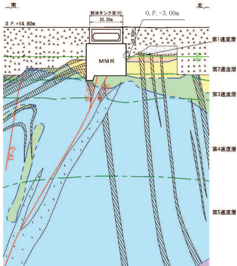
図 2-7(1) 軽油タンク室 (H) 地震時荷重算出用地質断面図 (A-A 断面, 南北)
