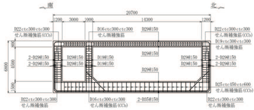
図 2-6(1) 軽油タンク室概略配筋図 (A-A 断面, 南北)
