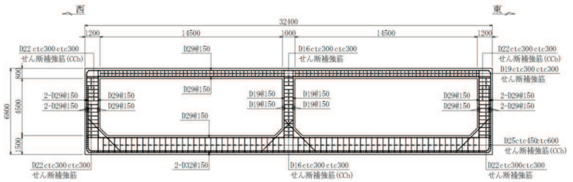
図 2-6(2) 軽油タンク室概略配筋図 (B-B 断面, 東西 (タンク室))
