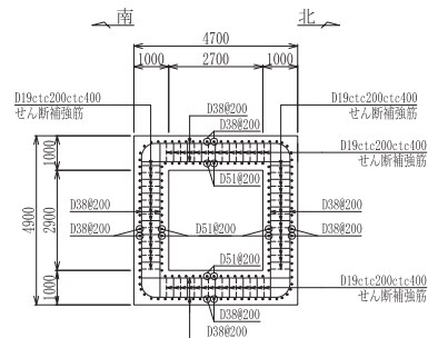
図 2-6(3) 軽油タンク室 (H) 概略配筋図 (接続部)
