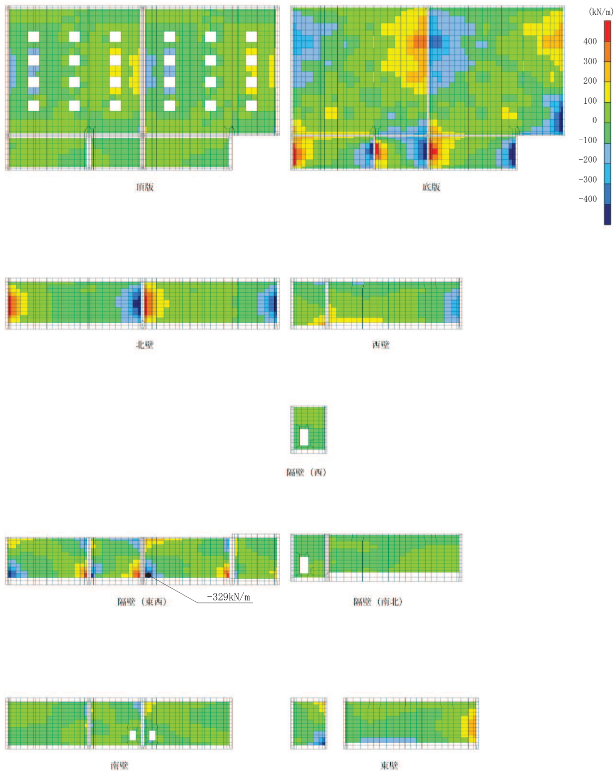
図 6-10(5) せん断破壊に対する照査値最大時の断面力分布図 (せん断力 (kN/m) : Q_x ) (隔壁 (東西), 解析ケース③, S_s - D 2 (+ +) , t = 25.09s )
