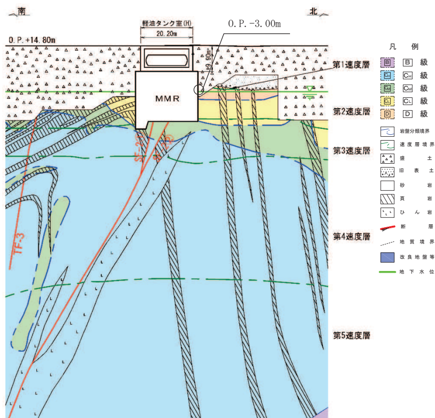
図 2-9(1) 設計用地下水位 (A-A 断面, 南北)
