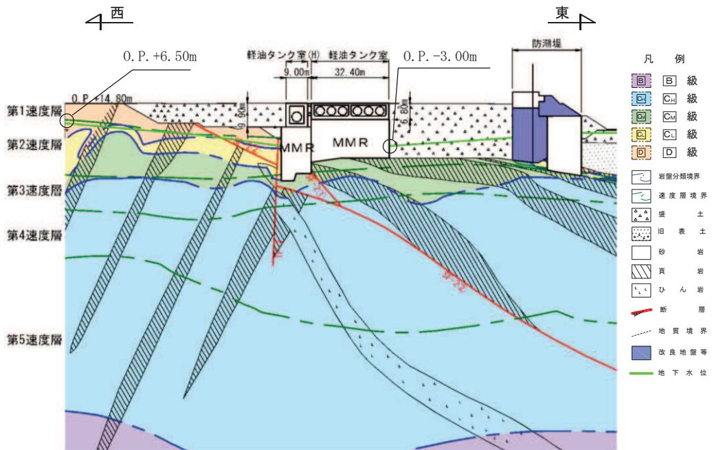
図 2-7(2) 軽油タンク室 (H) 地震時荷重算出用地質断面図 (B-B 断面, 東西)
