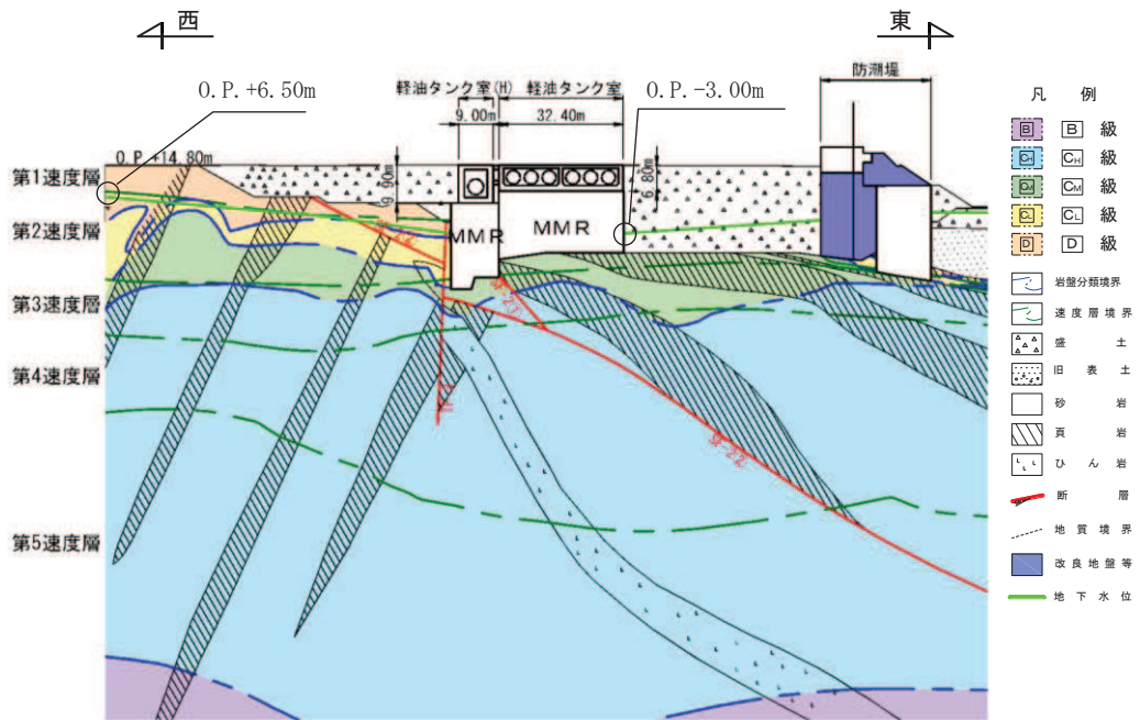
図 2-9(2) 設計用地下水位 (B-B 断面, 東西 (タンク室))
