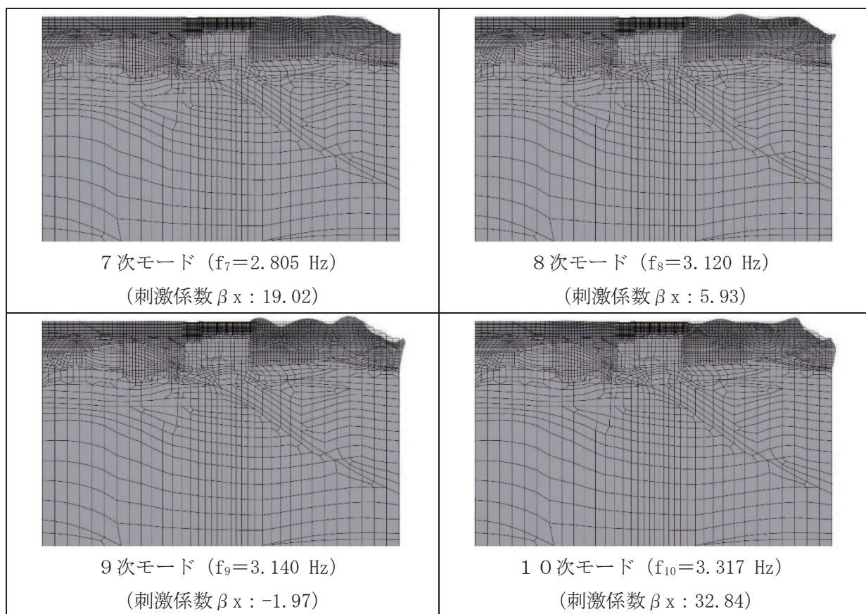
図 3-20(2) 固有値解析結果 (モード図) (B-B 断面, 東西(タンク室)) (2/2)
