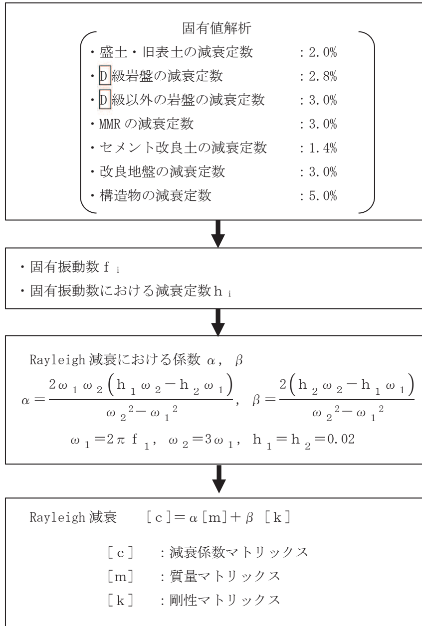
図 3-18 Rayleigh 減衰の設定フロー
