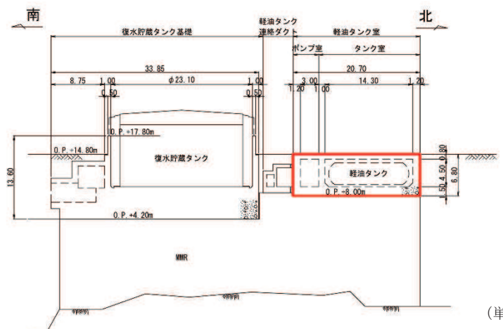
図 2-5(1) 軽油タンク室断面図 (A-A 断面, 南北)
