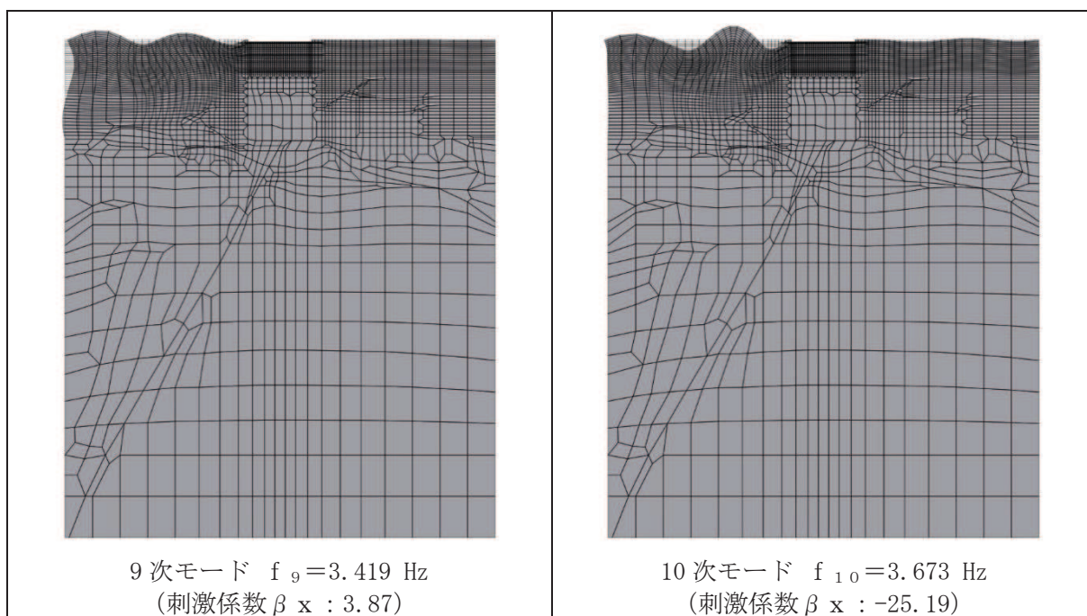
図 3-19(3) 固有値解析結果 (モード図) (A-A 断面, 南北) (3/3)
