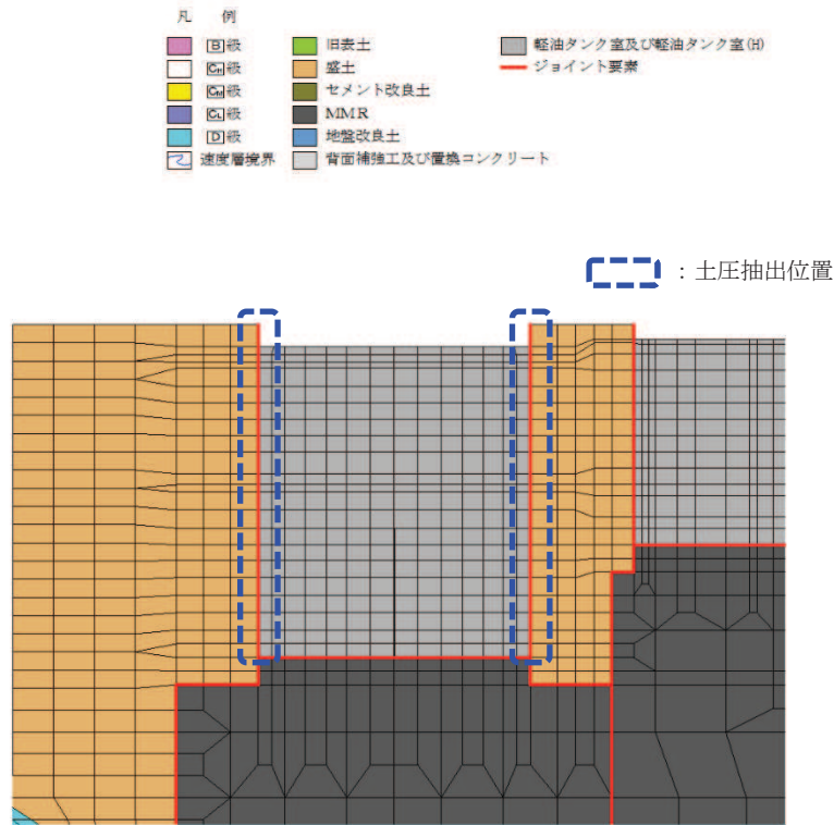
図4-10 地震時土圧及び周面せん断力抽出位置
