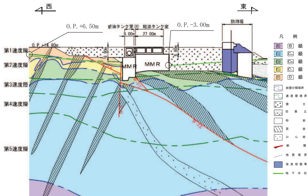
図 2-7(3) 軽油タンク室 地震時荷重算出用地質断面図 (C-C 断面, 東西 (ポンプ室))
