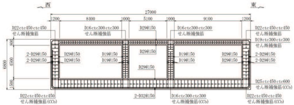
図 2-6(3) 軽油タンク室概略配筋図 (C-C 断面, 東西 (ポンプ室))
