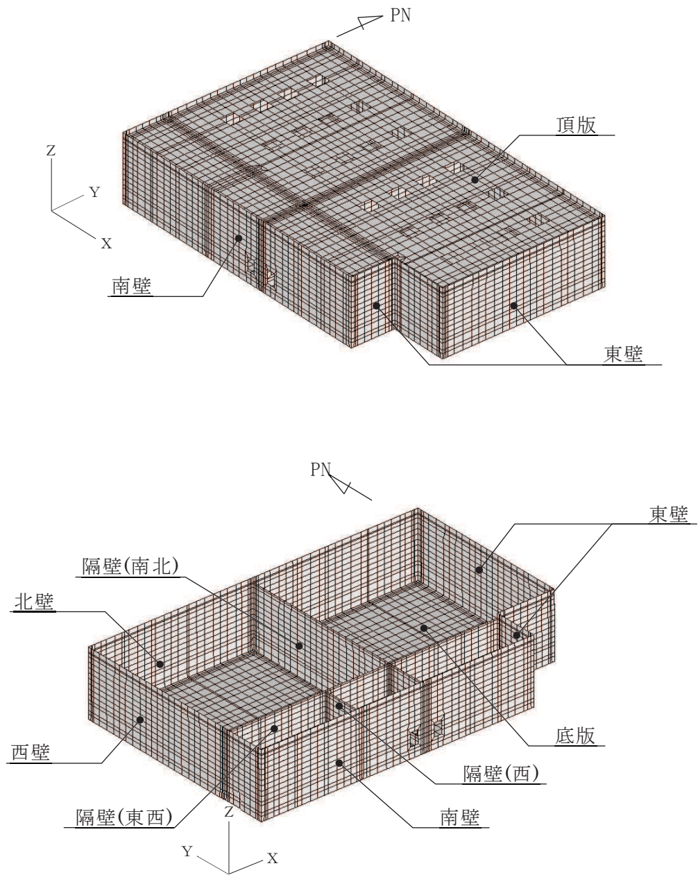
図 8-1 三次元構造解析モデル図
