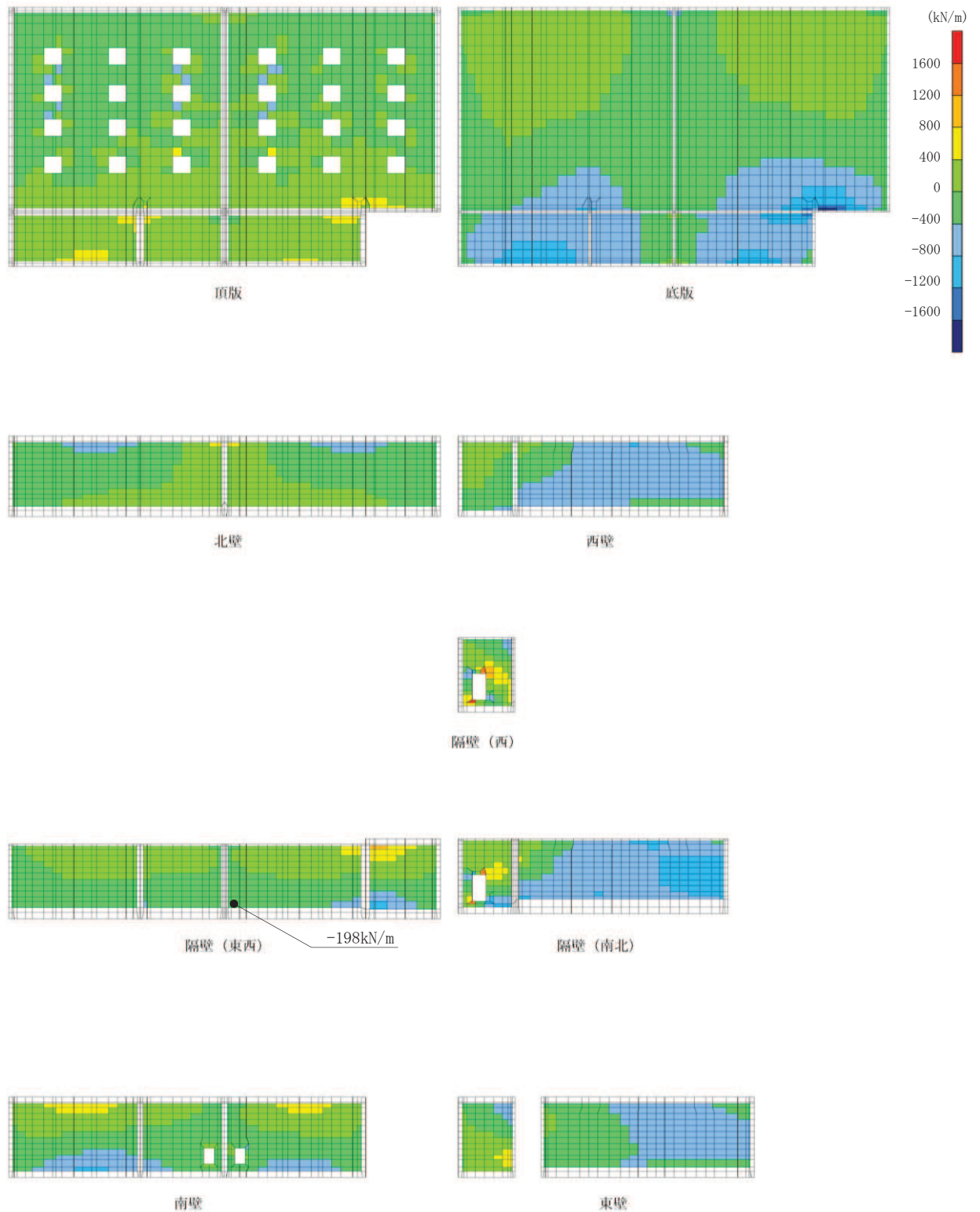
図 6-10(3) せん断破壊に対する照査値最大時の断面力分布図 (軸力 (kN/m) : N_x ) (隔壁 (東西), 解析ケース③, S_s - D_2 (++) , t = 25.09\text{s} )
