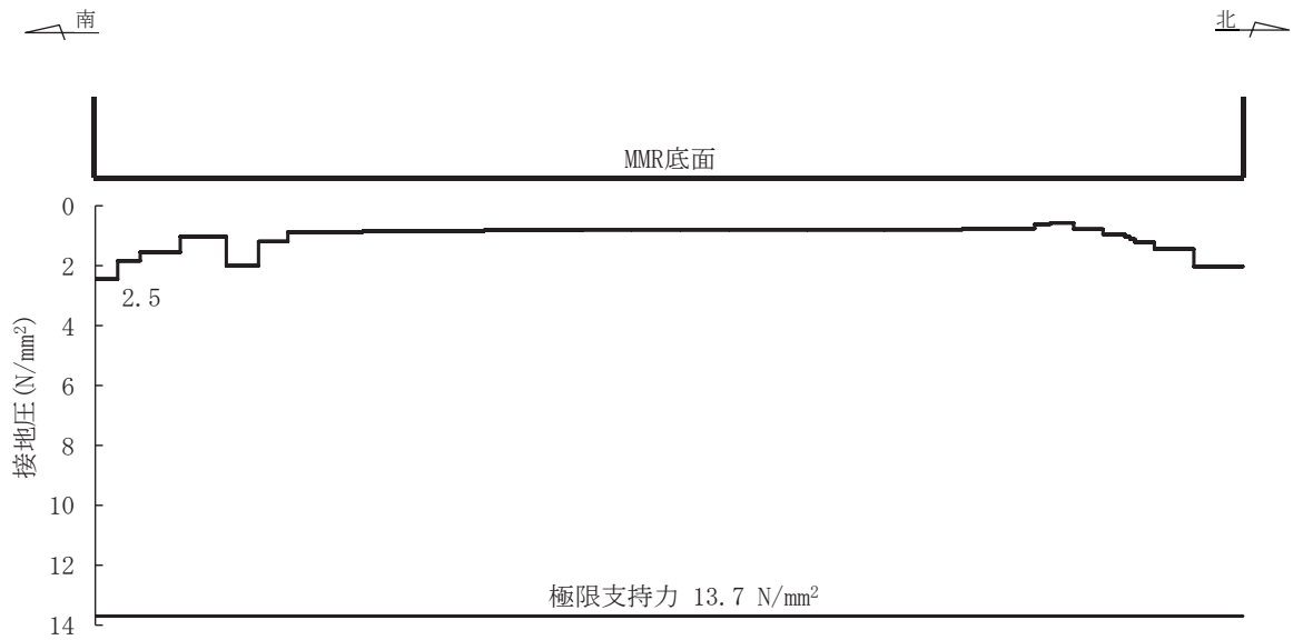
図 6-12 基礎地盤の最大接地圧分布図 (解析ケース②, S s -D2 (++))
