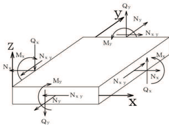
図 6-7 シェル要素における断面力の方向
