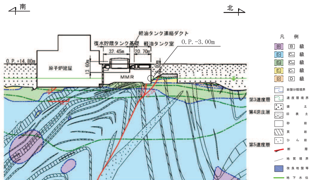
図 2-9(1) 設計用地下水位 (A-A 断面, 南北)
