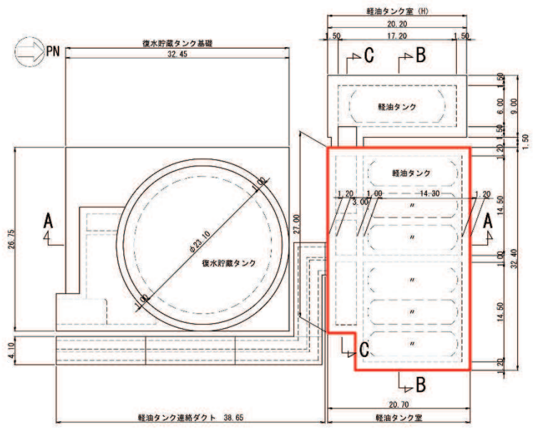
図 2-4 軽油タンク室平面図
