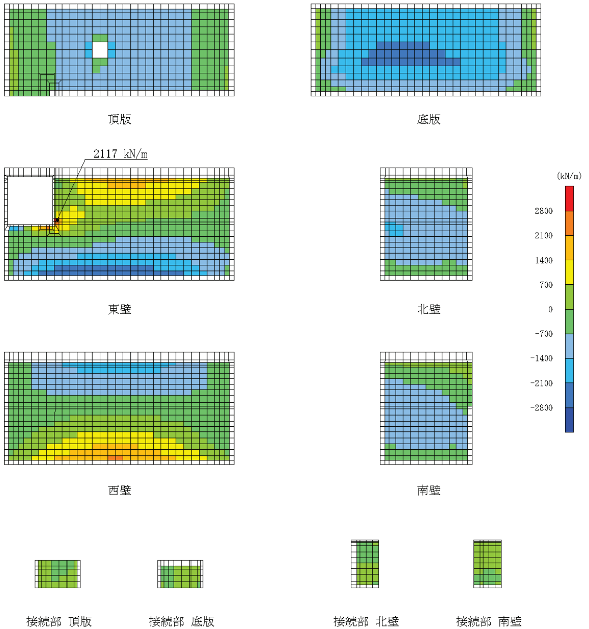
図 6-9 曲げ・軸力系の破壊に対する照査値最大時の断面力分布図 (軸力 (kN/m) : N_x ) (東壁, 解析ケース③, S_s - D 2 (++) , t = 8.58 s)
