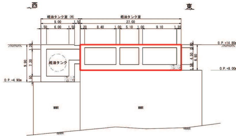
図 2-5(3) 軽油タンク室断面図 (C-C 断面, 東西 (ポンプ室))
