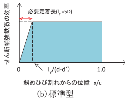
図 5-31 セラミックキャップバー (CCb) の有効率算定の概念図
