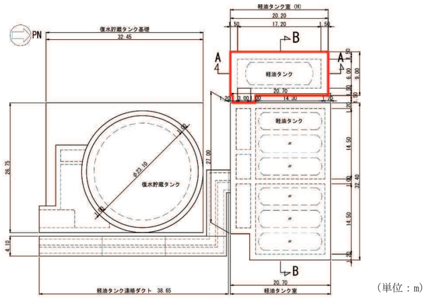
図 2-4 軽油タンク室 (H) 平面図
