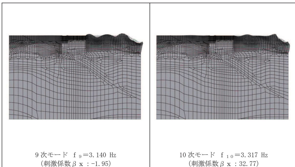
図 3-20(3) 固有値解析結果 (モード図) (B-B 断面, 東西) (3/3)
