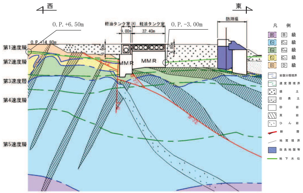
図 2-9(2) 設計用地下水位 (B-B 断面, 東西)
