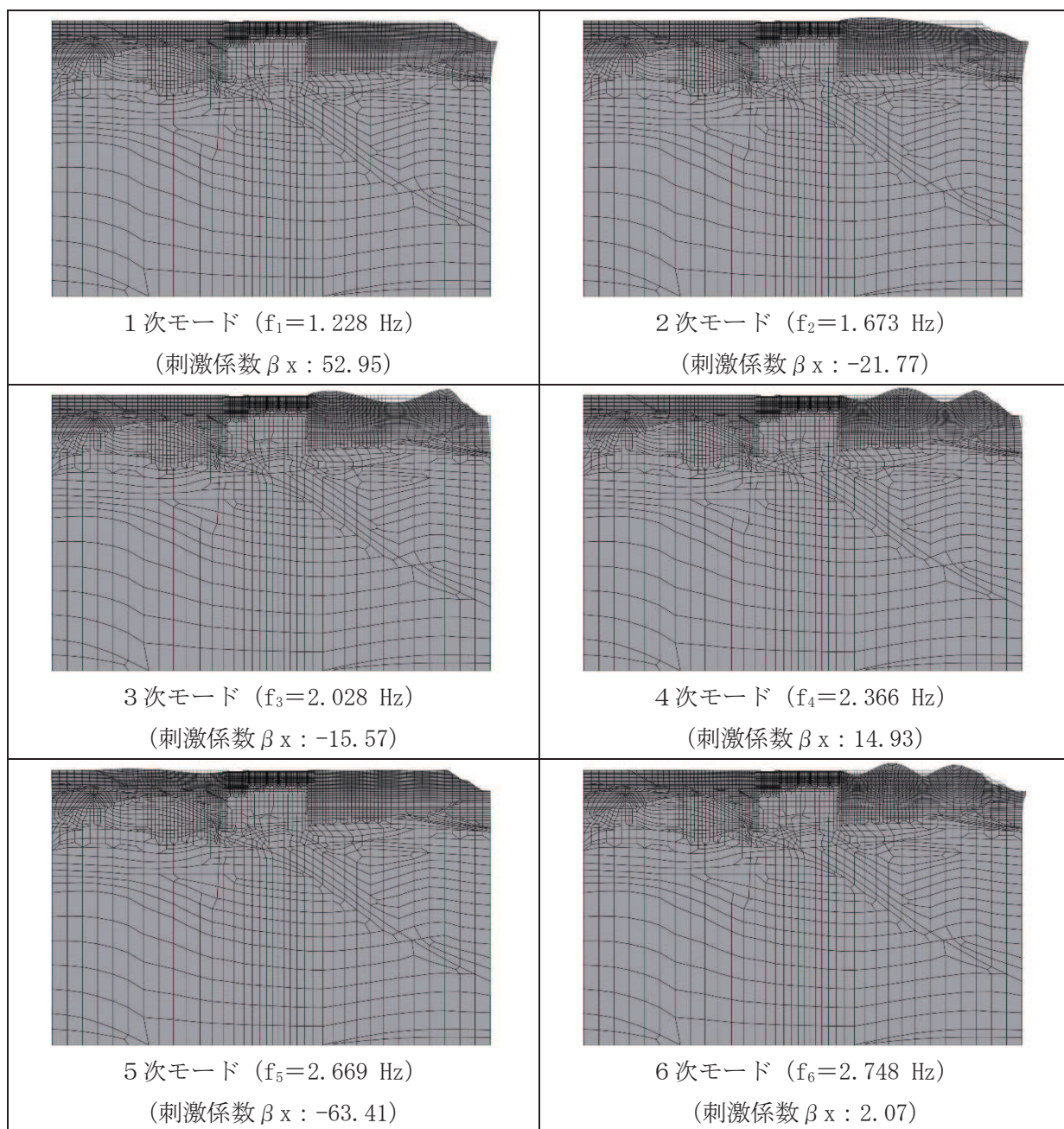
図 3-20(1) 固有値解析結果 (モード図) (B-B 断面, 東西(タンク室)) (1/2)
