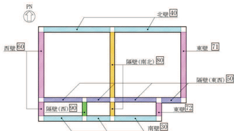
図 6-11 評価部材位置 (面内せん断ひずみ)
