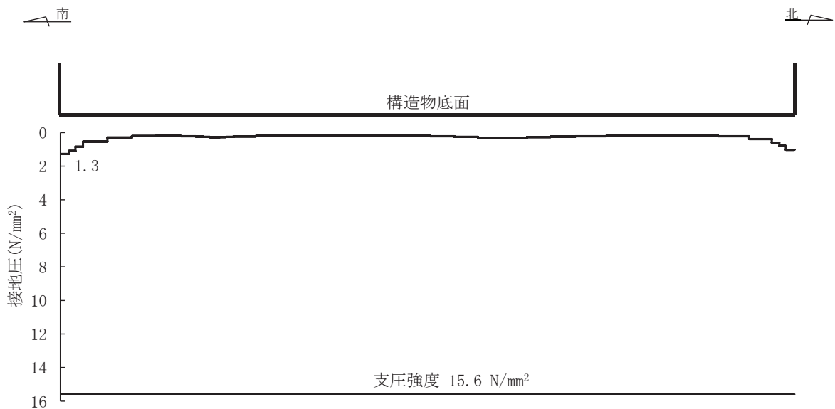
図 6-13 MMR (既設) の最大接地圧分布図 (解析ケース③, S s - D 2 (++) )
