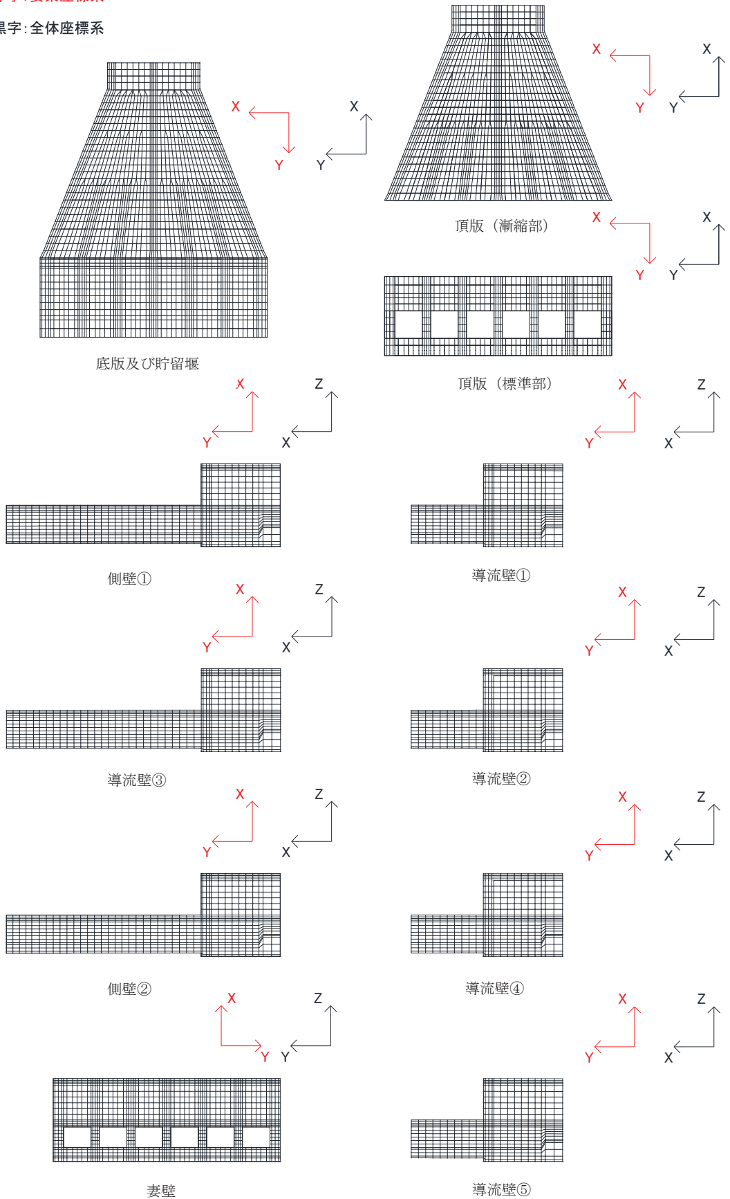
図 4-2 要素座標系
