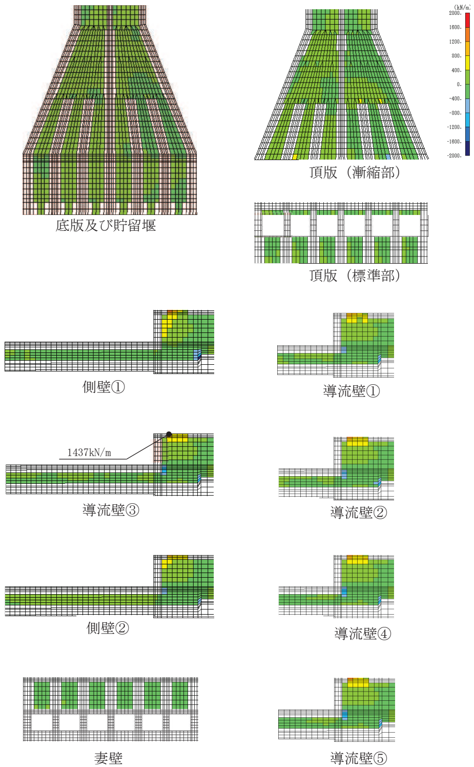
図 4-14 せん断破壊に対する照査における照査値最大時の断面力分布図 (せん断力 (kN/m) : Q_y ) (導流壁, 解析ケース①, S_s - D_2 (一+))
