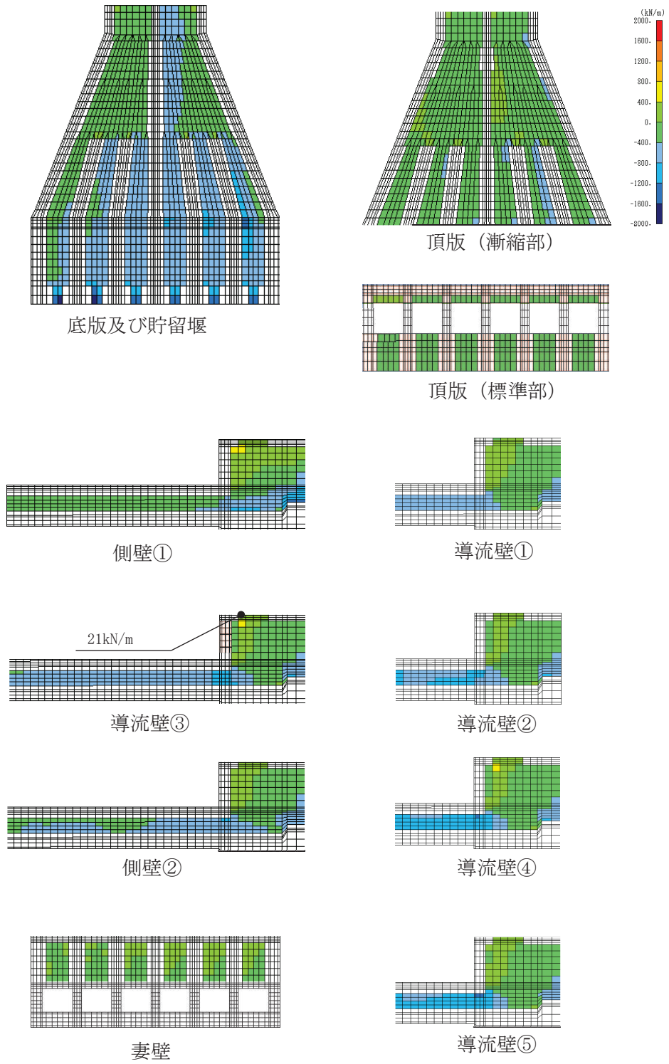
図 4-13 セン断破壊に対する照査における照査値最大時の断面力分布図 (せん断力 (kN/m) : Q_x ) (導流壁, 解析ケース①, S_s - D 2 (-+) )
