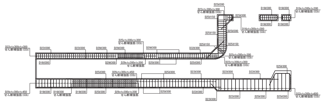
图 2-10 取水口概略配筋图 (纵断)
