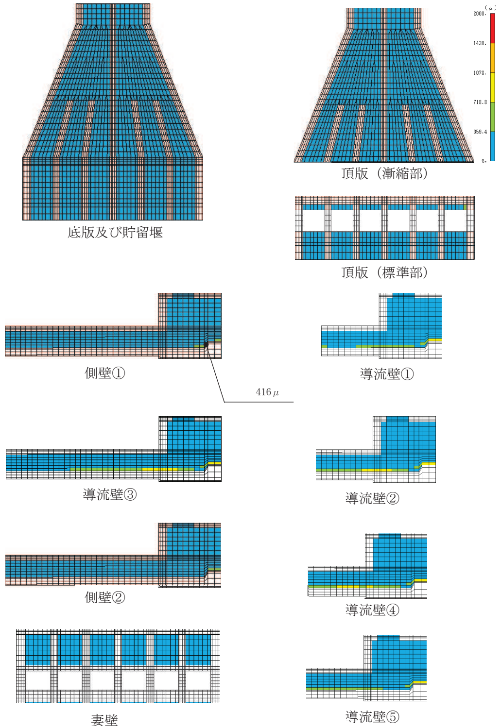
図 4-8 曲げ・軸力系の破壊に対する照査における照査値最大時のひずみ分布図（鉄筋） （側壁，解析ケース③，S s -D2（-+））
