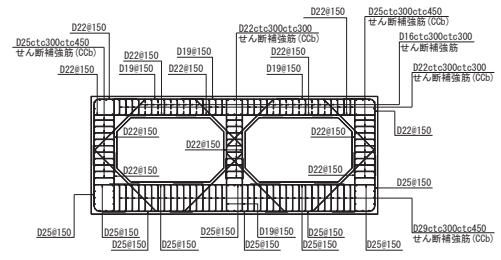
图 2-9 取水口概略配筋图 (C-C 断面, 渐缩部)
