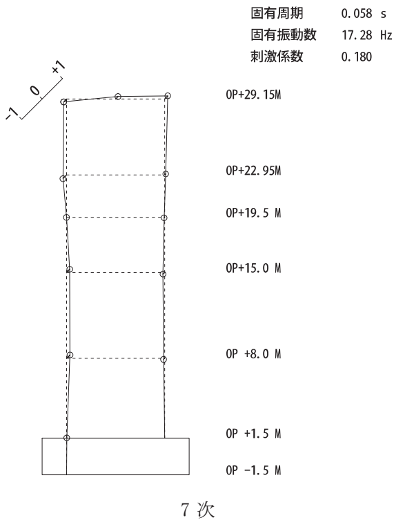
図 4-3(2) 刺激関数図 (ケース 4) (EW 方向 5 次~8 次)
