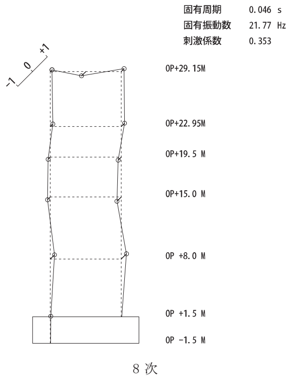
図 4-3(2) 刺激関数図 (ケース 4) (EW 方向 5 次~8 次)
