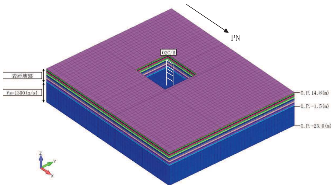
(b) 鳥観図：建屋部分拡大図
