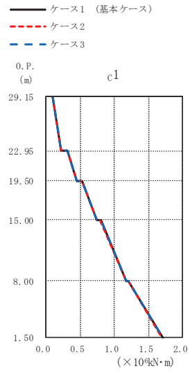
図 2-47 (1) 最大応答曲げモーメント (弾性設計用地震動 S d, EW 方向) (1/2)
