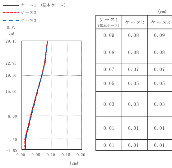
図 2-28 (2) 最大応答変位 (基準地震動 S_s , UD 方向) (2/2)
