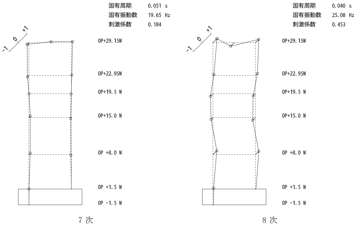
図 4-8(2) 刺激関数図 (ケース 3) (EW 方向 5 次~8 次)
