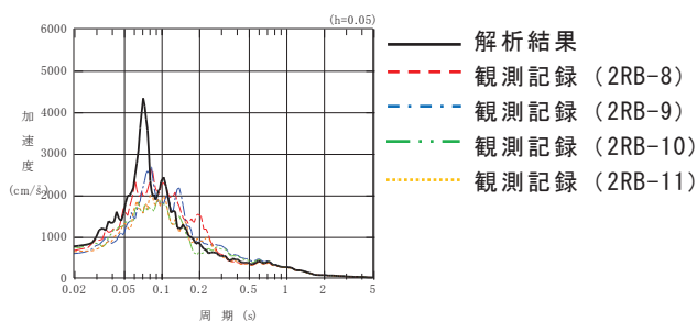
地上3階
