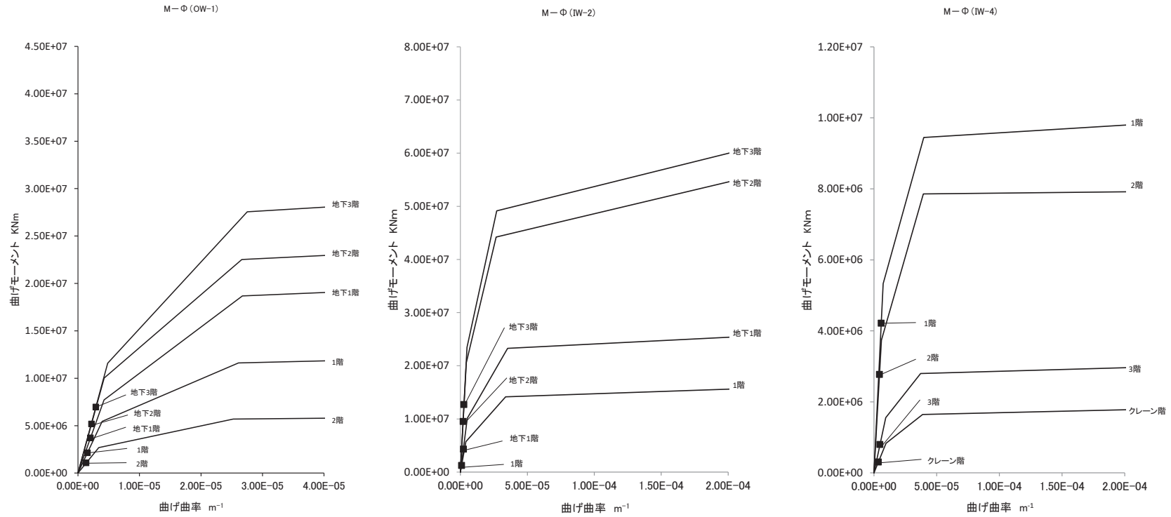
図 2-51 原子炉建屋 曲げスケルトン曲線上の最大応答値(EW 方向) 3.11 地震 (1/2)
