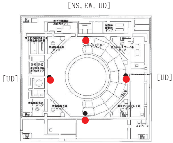
基礎版上 (O. P. -8. 1m)
