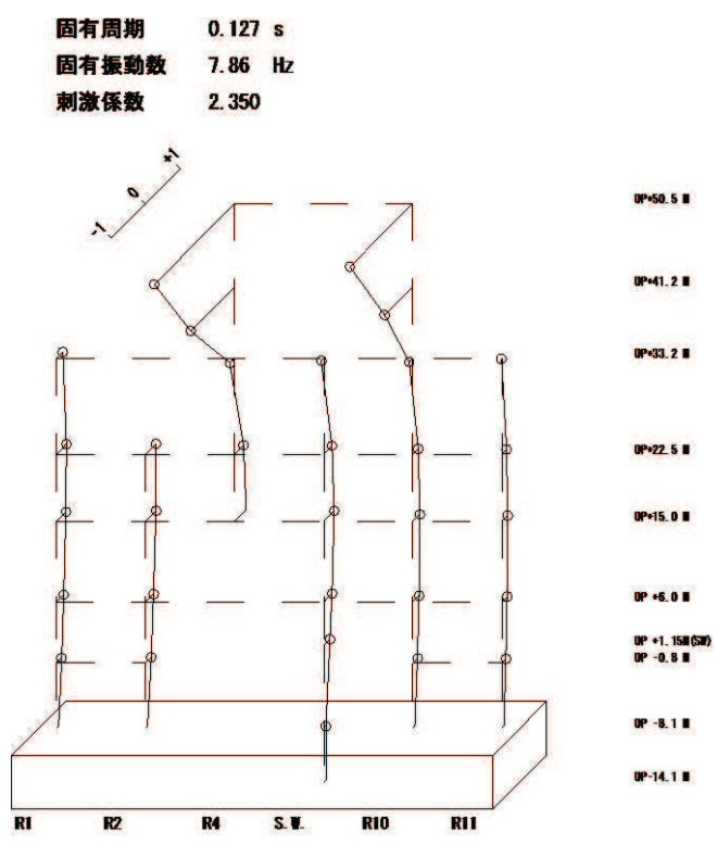
2 次モード
