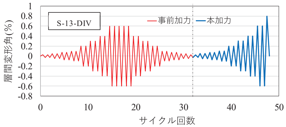
図 3.2-2 加力概念図
