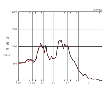
基礎版上 (0. P. -8.1m)
