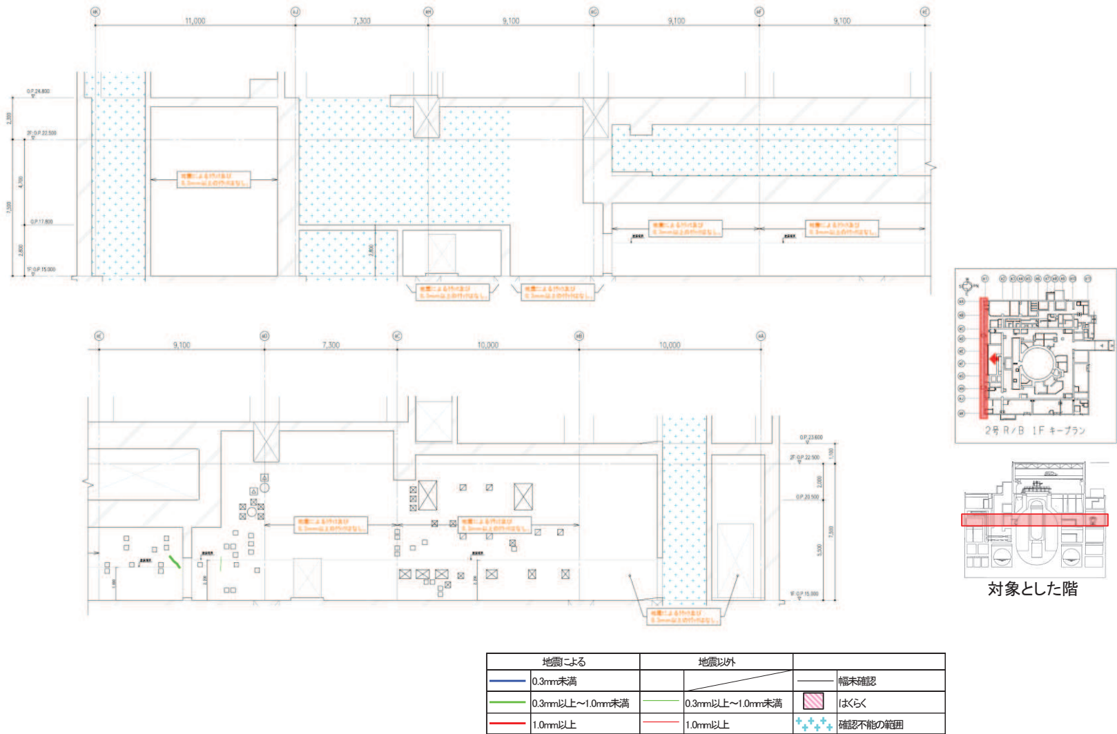
図 29 原子炉建屋のひび割れ分布 耐震壁 (29) 地上 1 階 R1 通り
