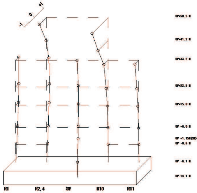
3次モード
