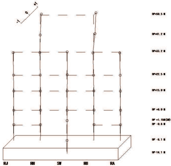
6次モード
