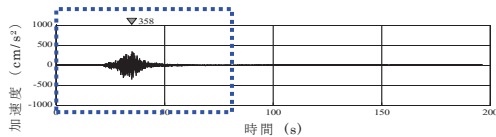
4.7 地震 加速度波形
