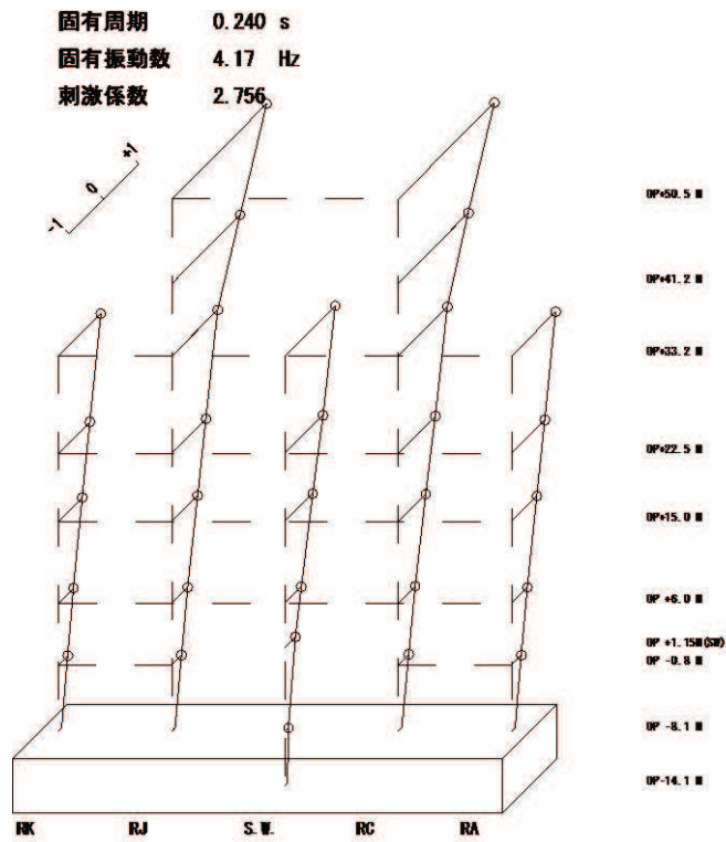
1次モード
