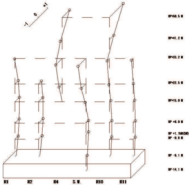
6次モード
