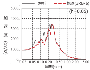
(地上3階)
