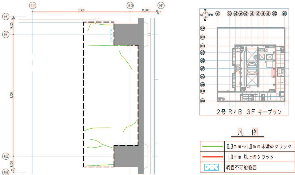
図 2.3-16 (1) 原子炉建屋地上 3 階床ひび割れ調査結果 (発生応力の大きい部位を選定)
