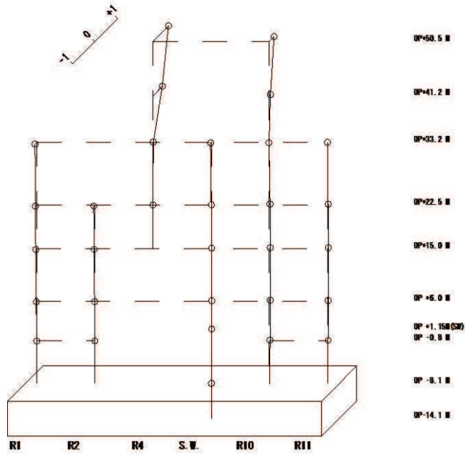
5次モード
