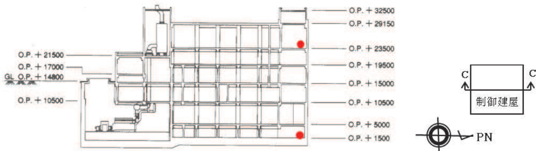
図 3-2 女川第1号機制御建屋の地震計位置
