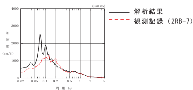
地上1階
