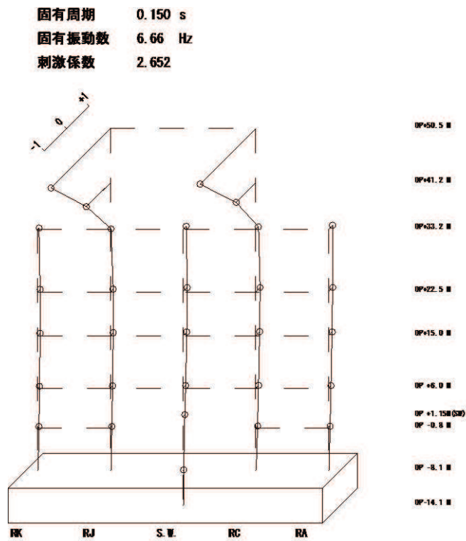
2次モード
