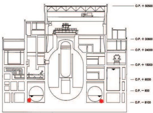
AA 断面
