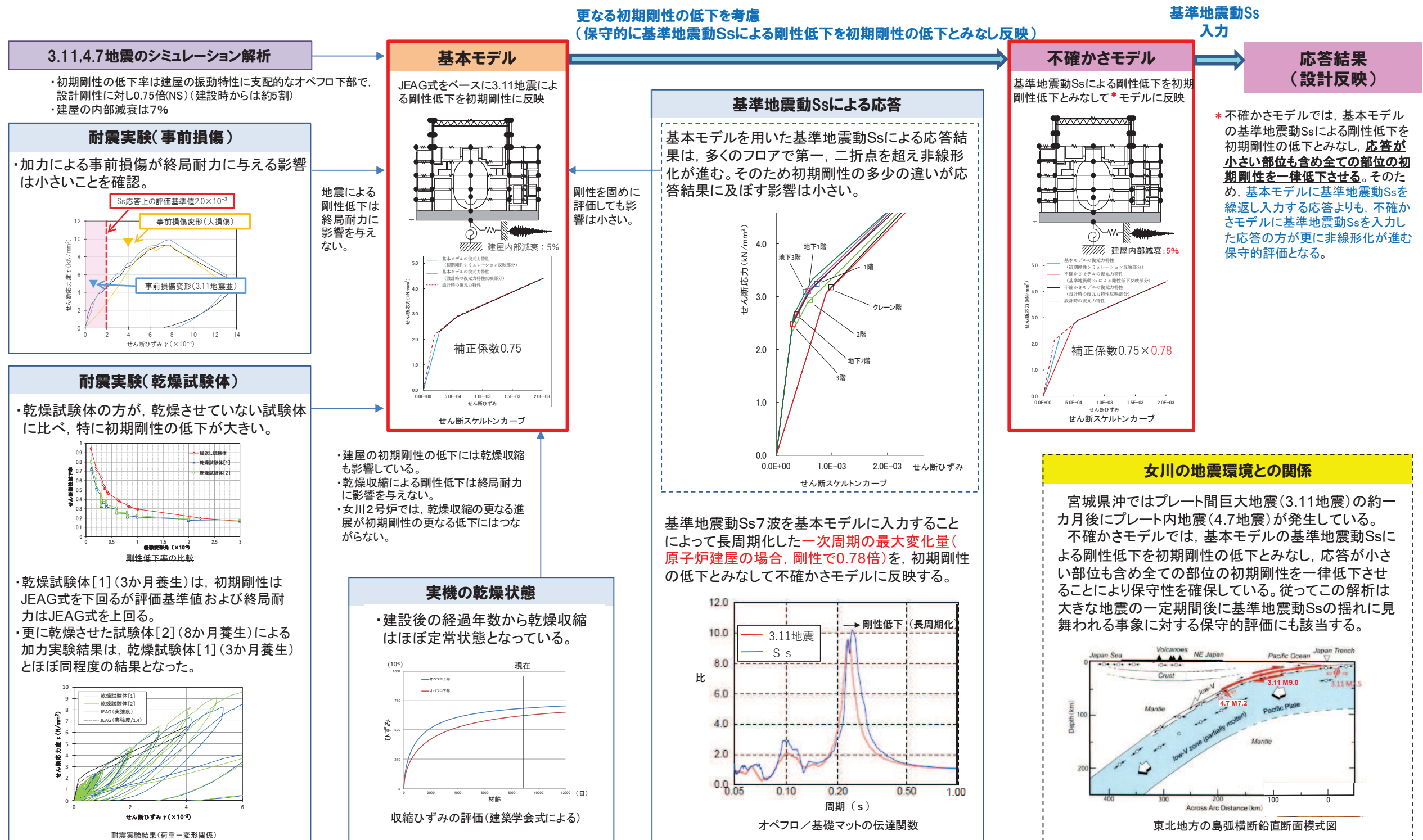
図1-4 原子炉建屋の地震による初期剛性低下を反映した基準地震動Ssに対する地震応答解析モデル
