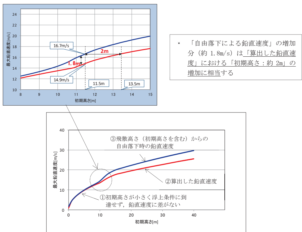
図 11 鉛直速度と初期高さの関係（鋼製材，流入層高さ：17.5m）
