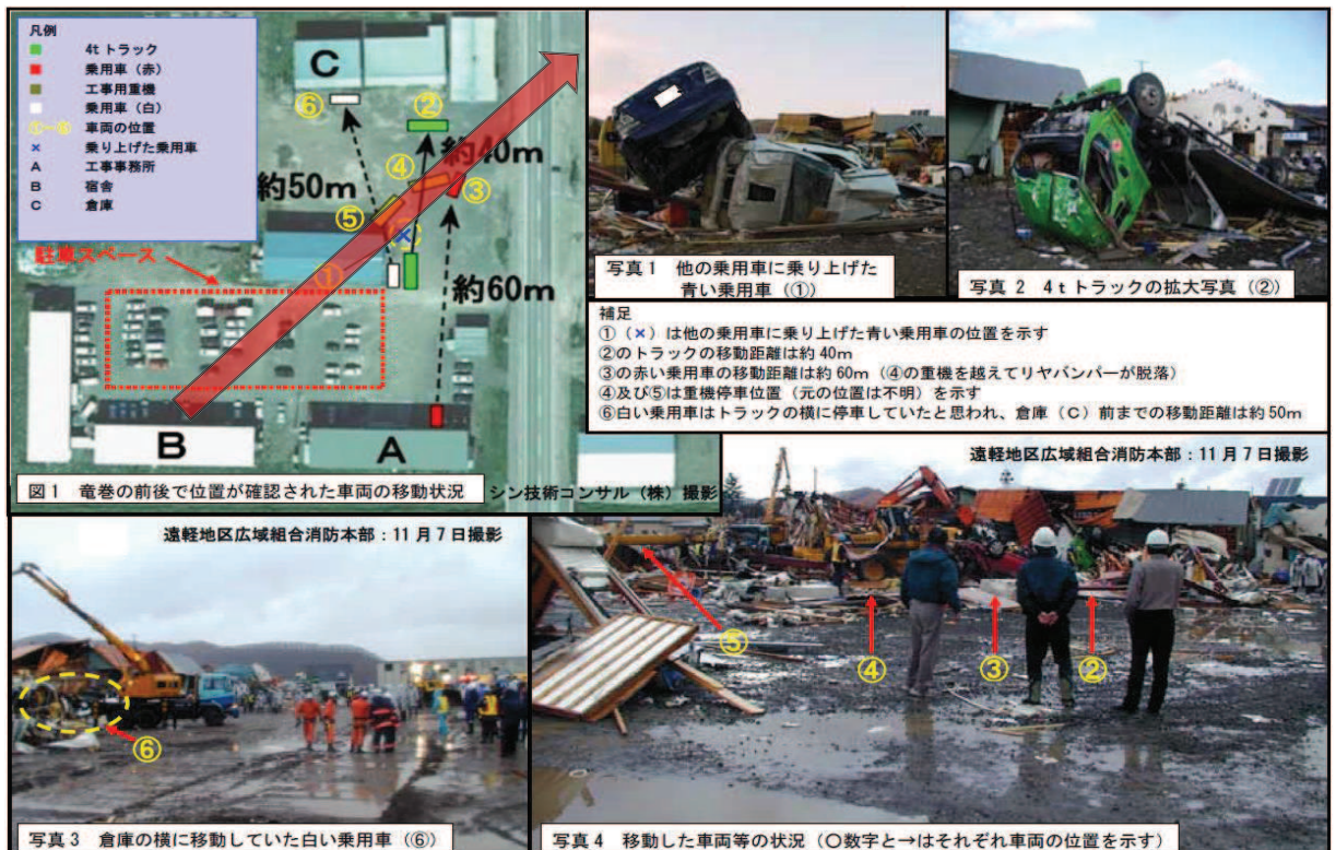
図34 佐呂間竜巻 (2006.11.7) による被災状況 (工事事務所敷地内の車両被災) (25)
