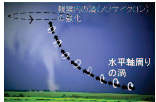
水平渦度の親雲への輸送に関する模式図
