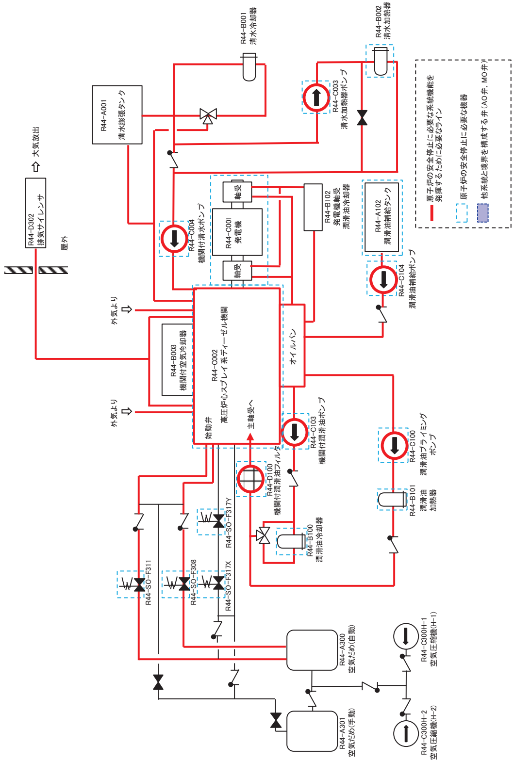
図 13 高圧炉心スプレイ系ディーゼル発電設備
