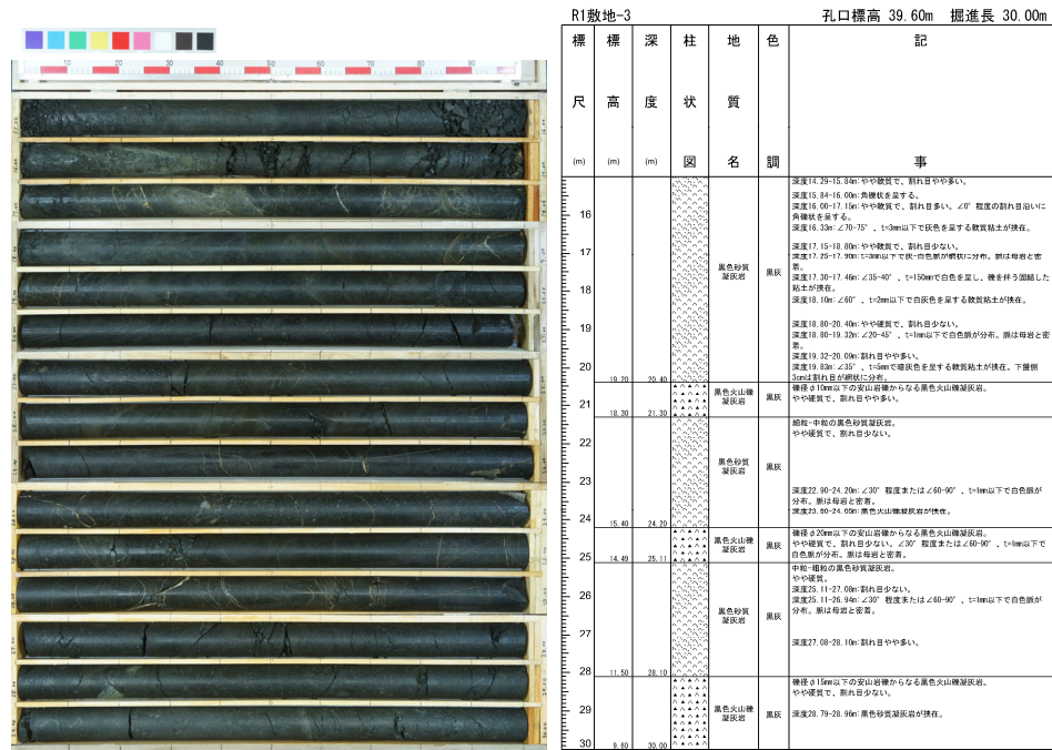
コア写真 (R1敷地-3: 深度15~30m)
