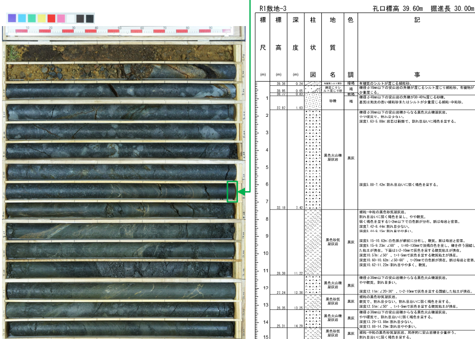
コア写真 (R1敷地-3: 深度0~15m)
