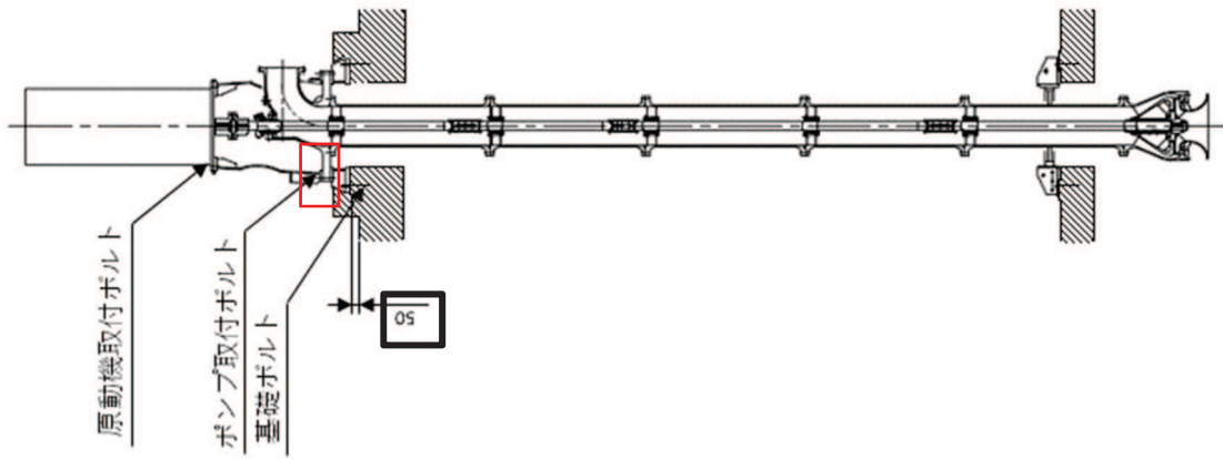
構造概要図
