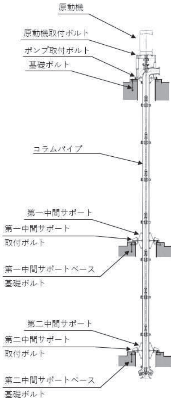
図5 高圧炉心スプレイ補機冷却海水ポンプ概要図 (1/2)
