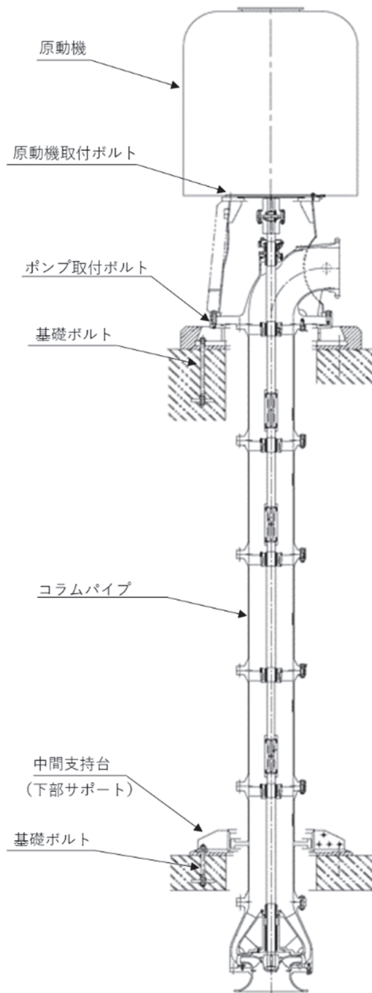
図4 原子炉補機冷却海水ポンプ概要図 (1/2)
