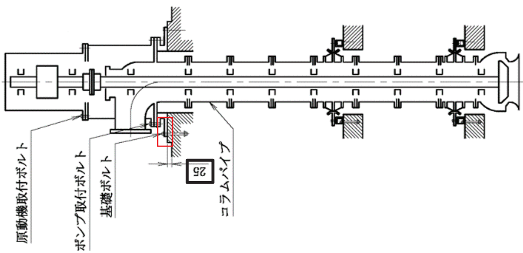
構造概要図
