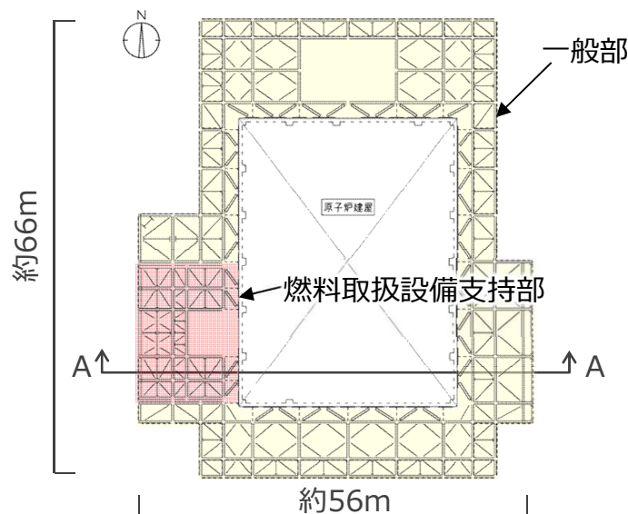
大型カバー平面図 (G.L. +28,300mm)
