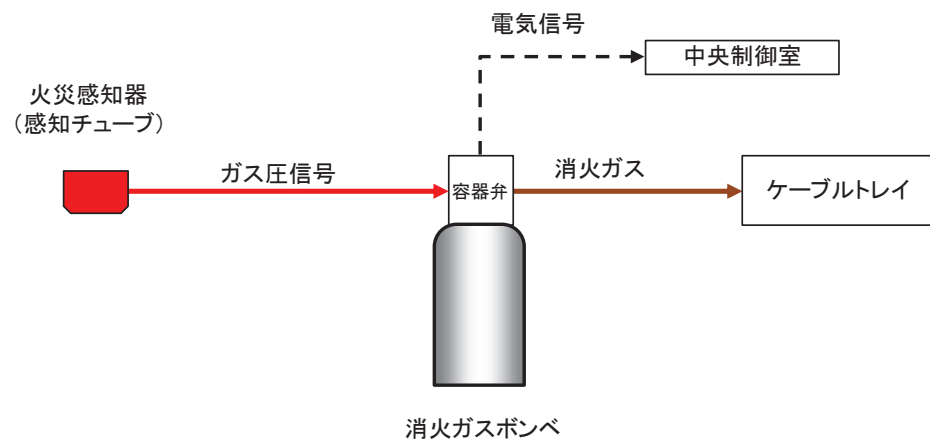
図 18 ケーブルトレイ消火設備の系統構成
