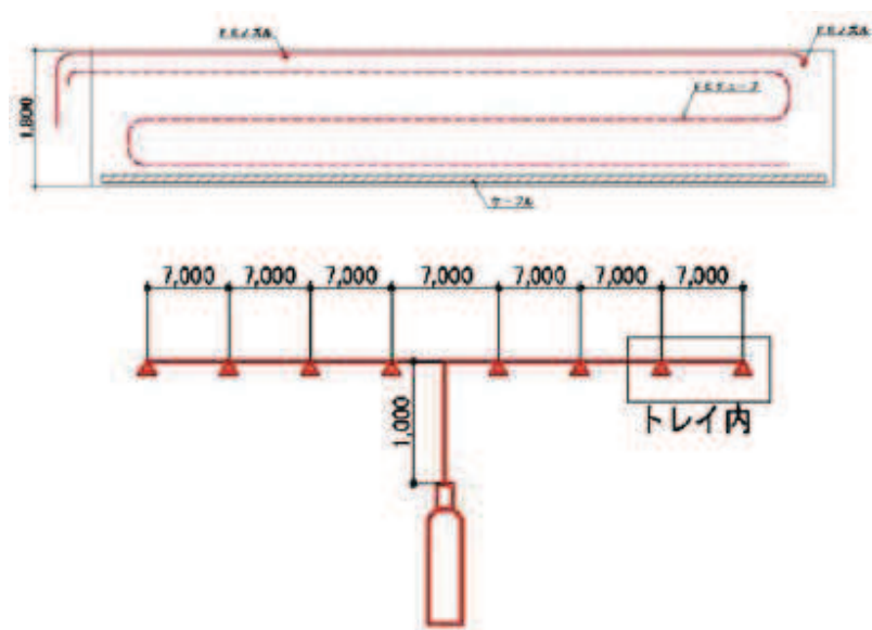
図 4 試験 H1 における検知チューブ等の配置概要
