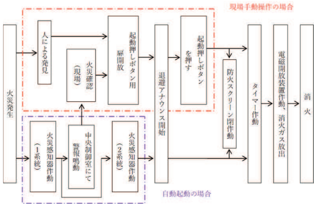
図 14 火災時の信号の流れ（モータコントロールセンタ）
