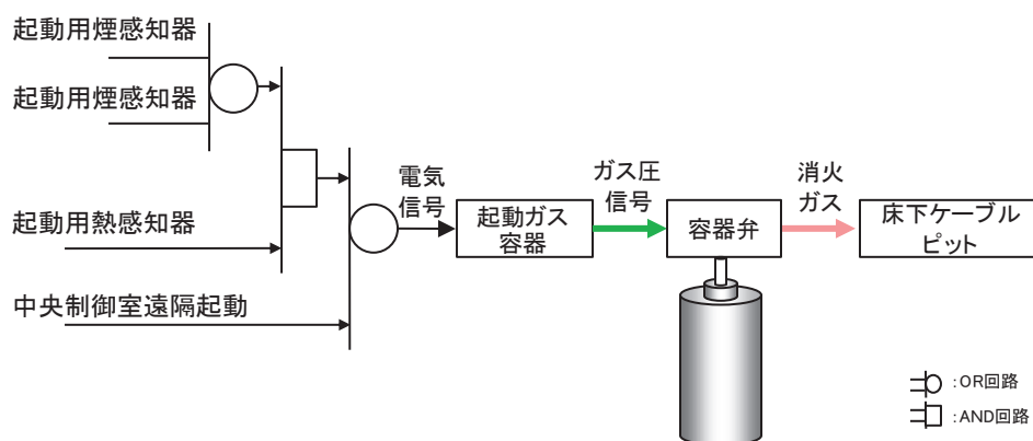
図 17 ハロンガス消火設備（局所）（中央制御室床下ケーブルピット）の系統構成
