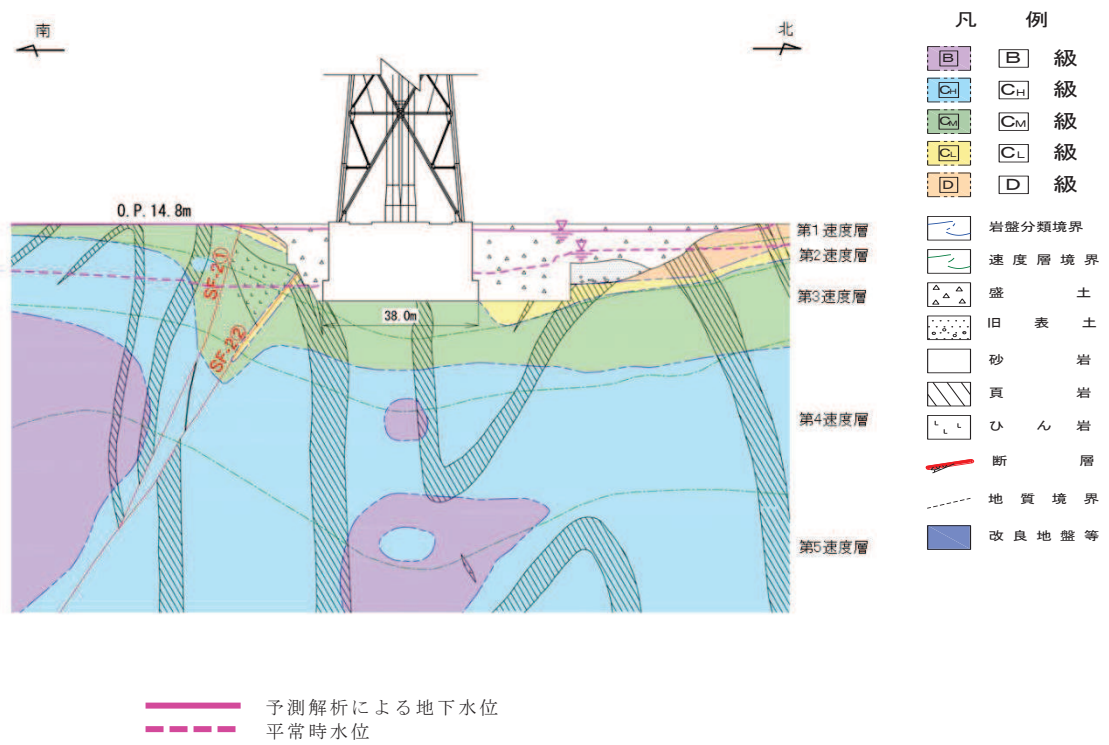
図 3.3-64 排気筒周辺における平常時水位分布(参考)
