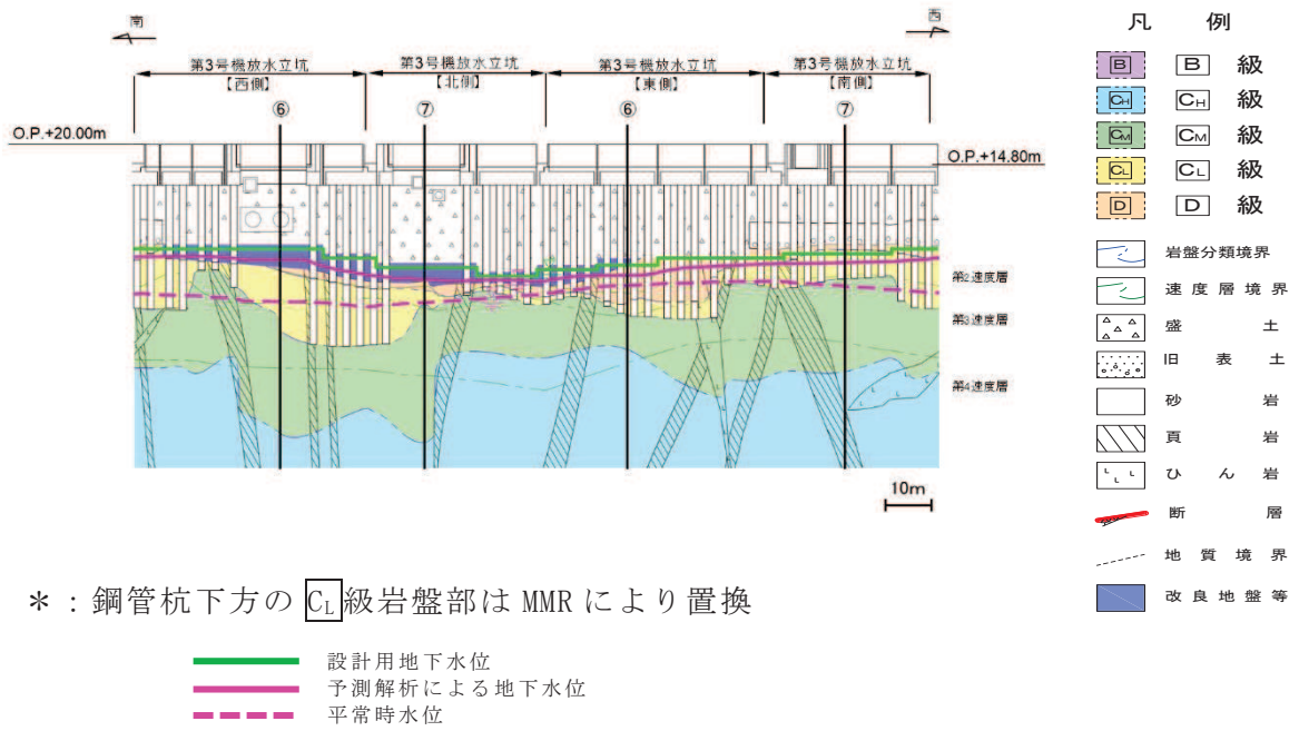
図 3.3-74 (9) 防潮壁における設計用地下水位と平常時水位の比較 (3号機放水立坑) (1/3)
