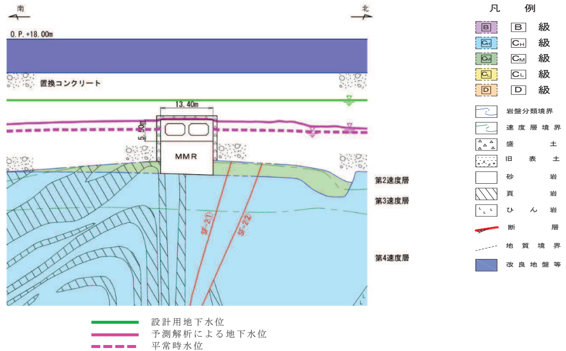
図 3.3-68 (4) 取水路における 設計用地下水位と平常時水位の比較 (横断(標準部③)) (防潮堤を横断する箇所(1))
