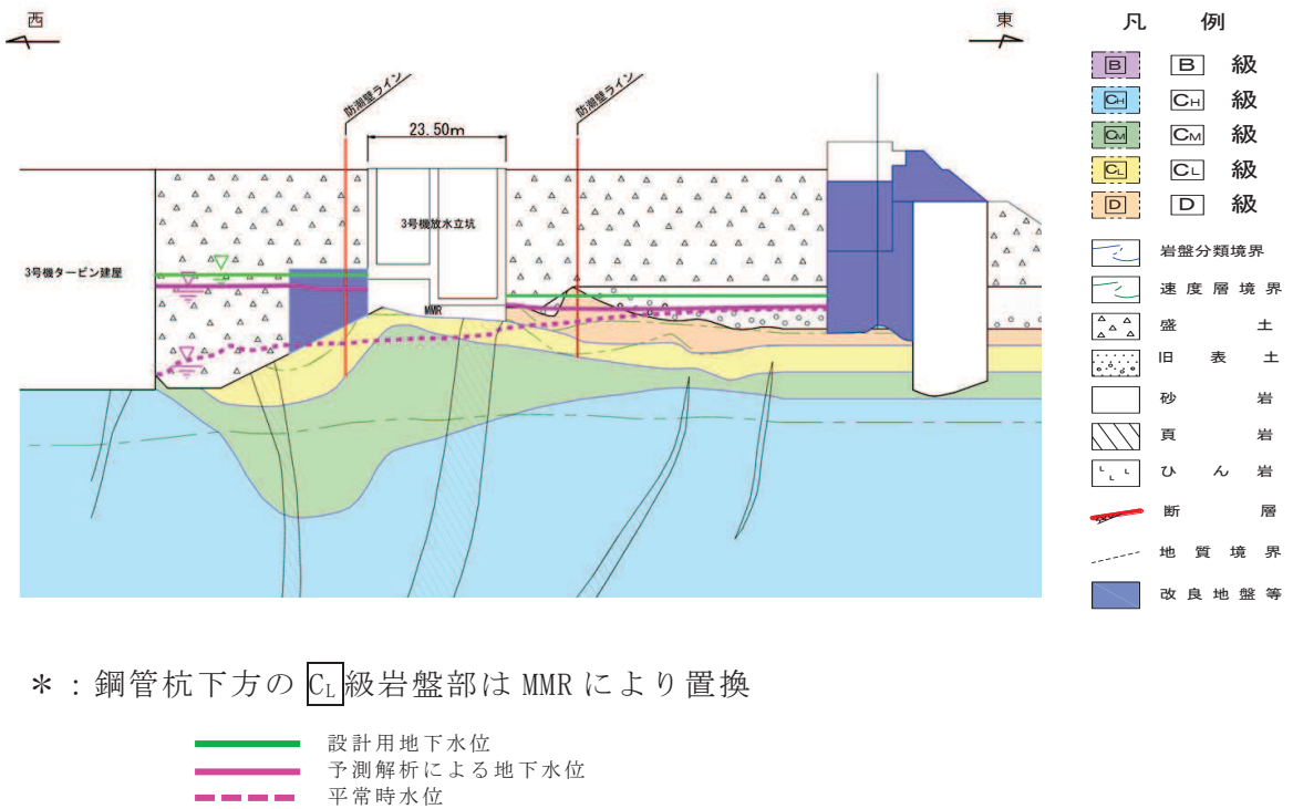
図 3.3-74 (10) 防潮壁における設計用地下水位と平常時水位の比較 (3号機放水立坑) (3号機放水立坑横断方向の地下水位分布(東西)⑤-⑤) (2/3)
