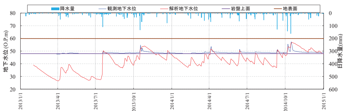
図 3.3-20 (8) 解析水位と観測水位の経時変化 (観測井⑭) (期間 2)
