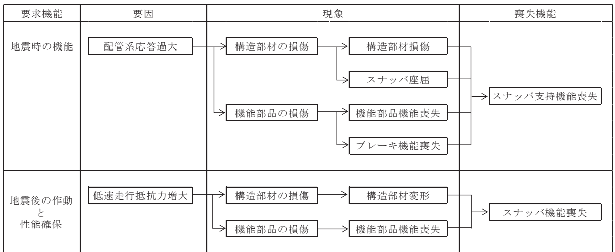
図 4-4 メカニカルスナップ異常要因モード
