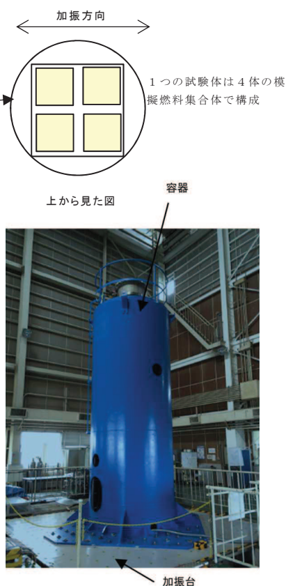
図 4-3 試験装置外観
