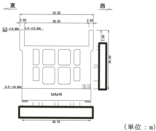
図 3-3-26 海水ポンプ室縦断図 (A-A)
