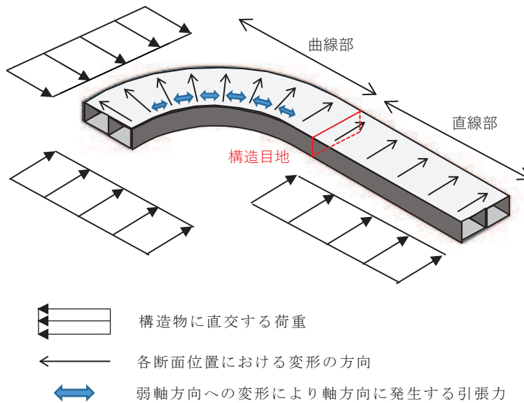
図3-3-17 取水路 (標準部) における変形
