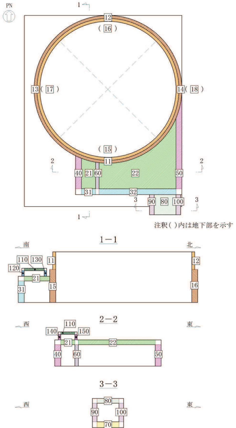
図 3-3-45 復水貯蔵タンク基礎（しゃへい壁，バルブ室及び連絡ダクト）評価位置図
