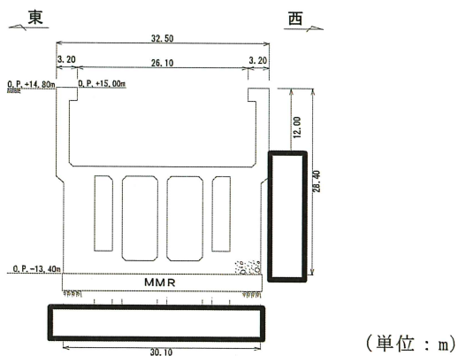
図 3-3-27 海水ポンプ室断面図 (B-B)
