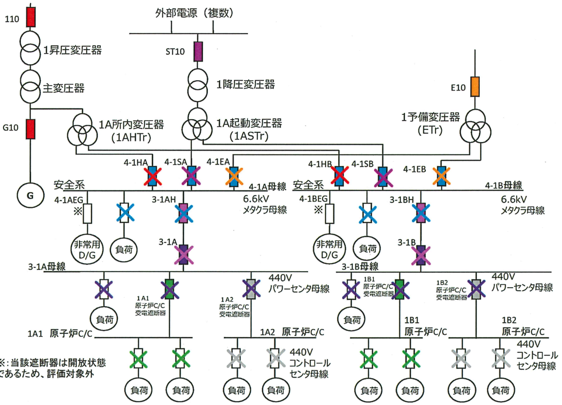
第2-1図 アーク放電発生箇所とアーク放電を遮断するための対策 (外部電源又は主発電機からの給電時)
