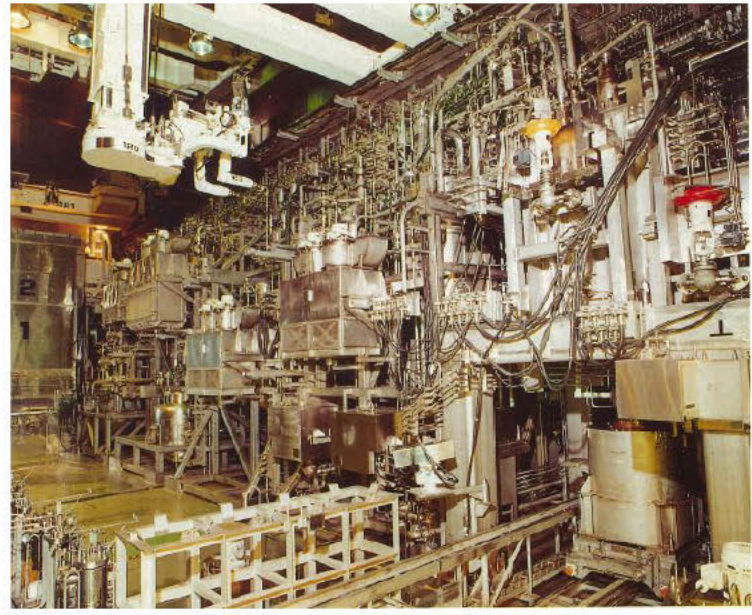
固化セル内
