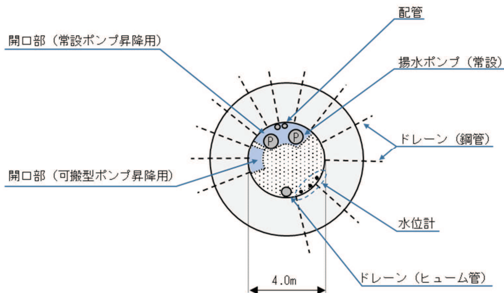
図 5-1 揚水井戸内の揚水ポンプ配置例
