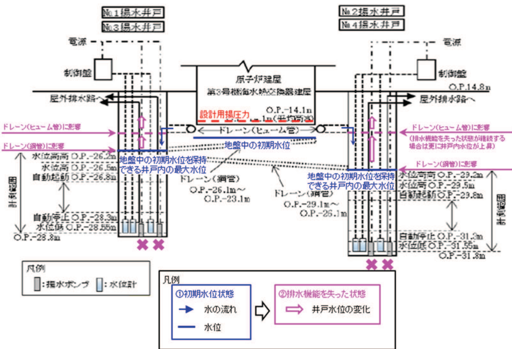
図 3-7 揚水井戸内の水の挙動（概念図）
