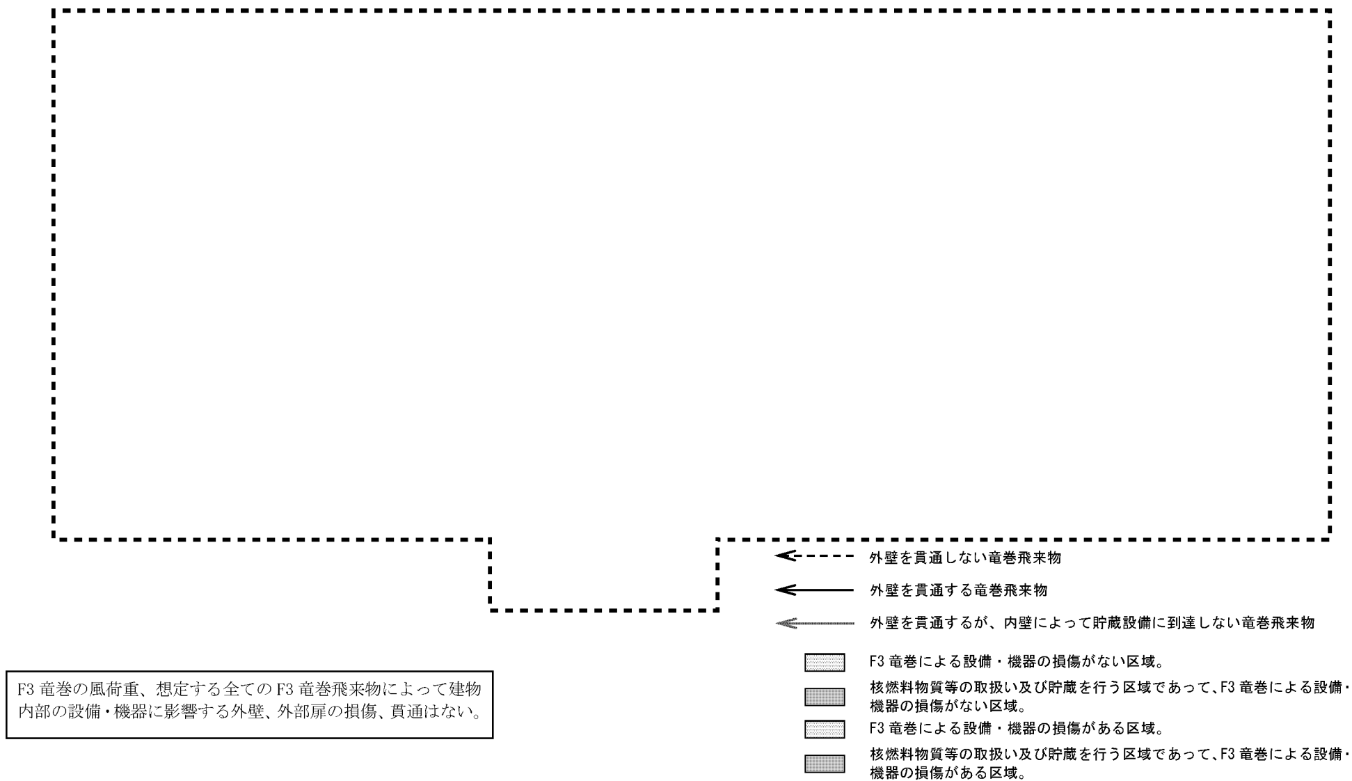
図1 F3 竜巻における第2加工棟1階の損傷状況
