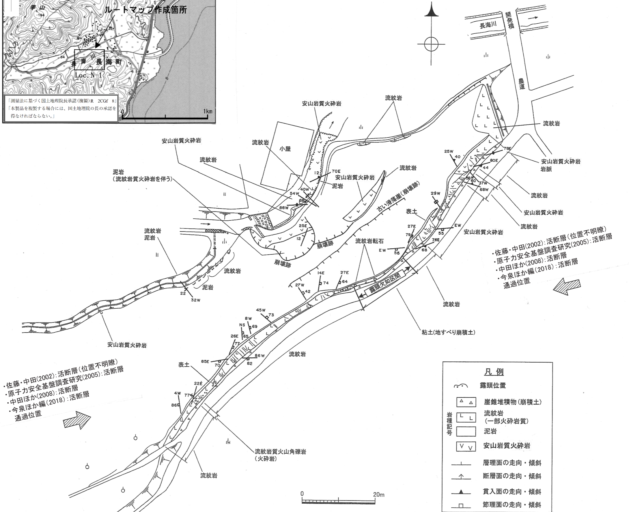
第 3.3-42 図 ルートマップ (長海町地点: Loc. N-1)
