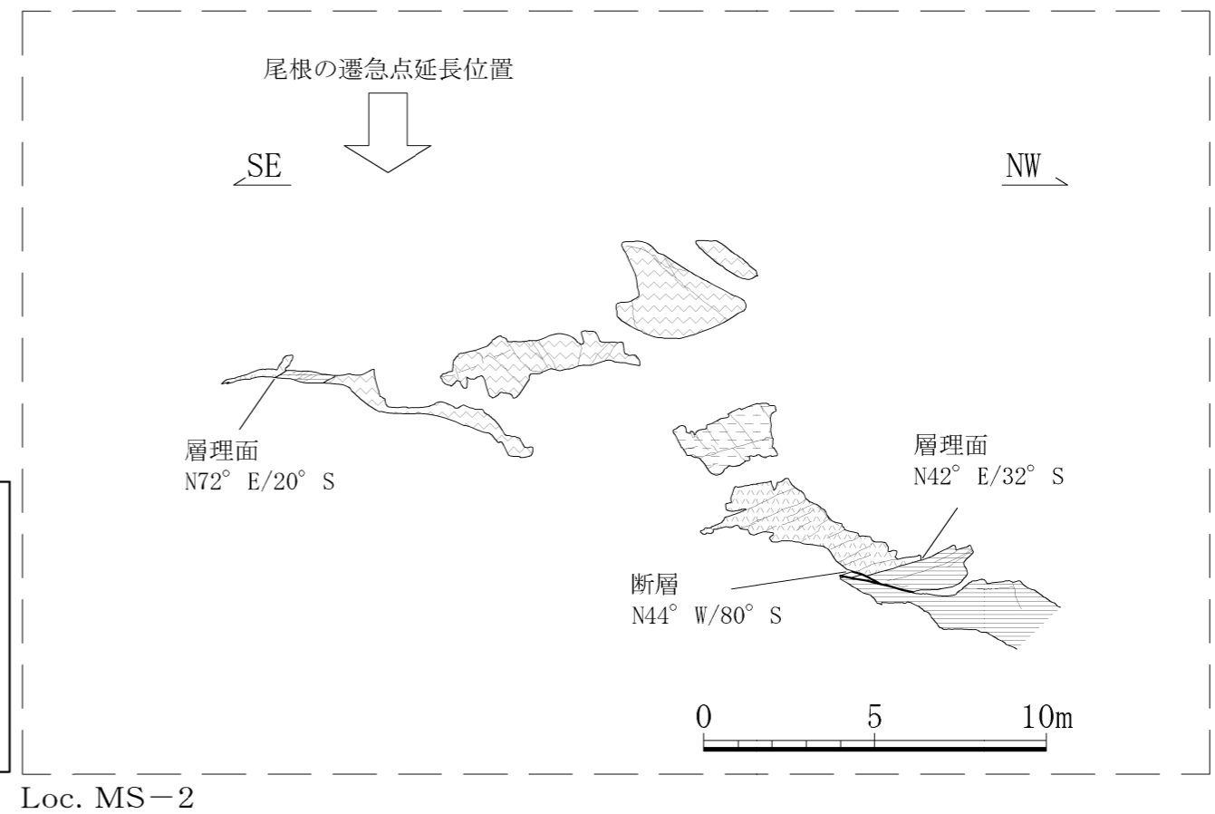
第3.3-34図 露頭スケッチ (女島西方: Loc. MS-2)
