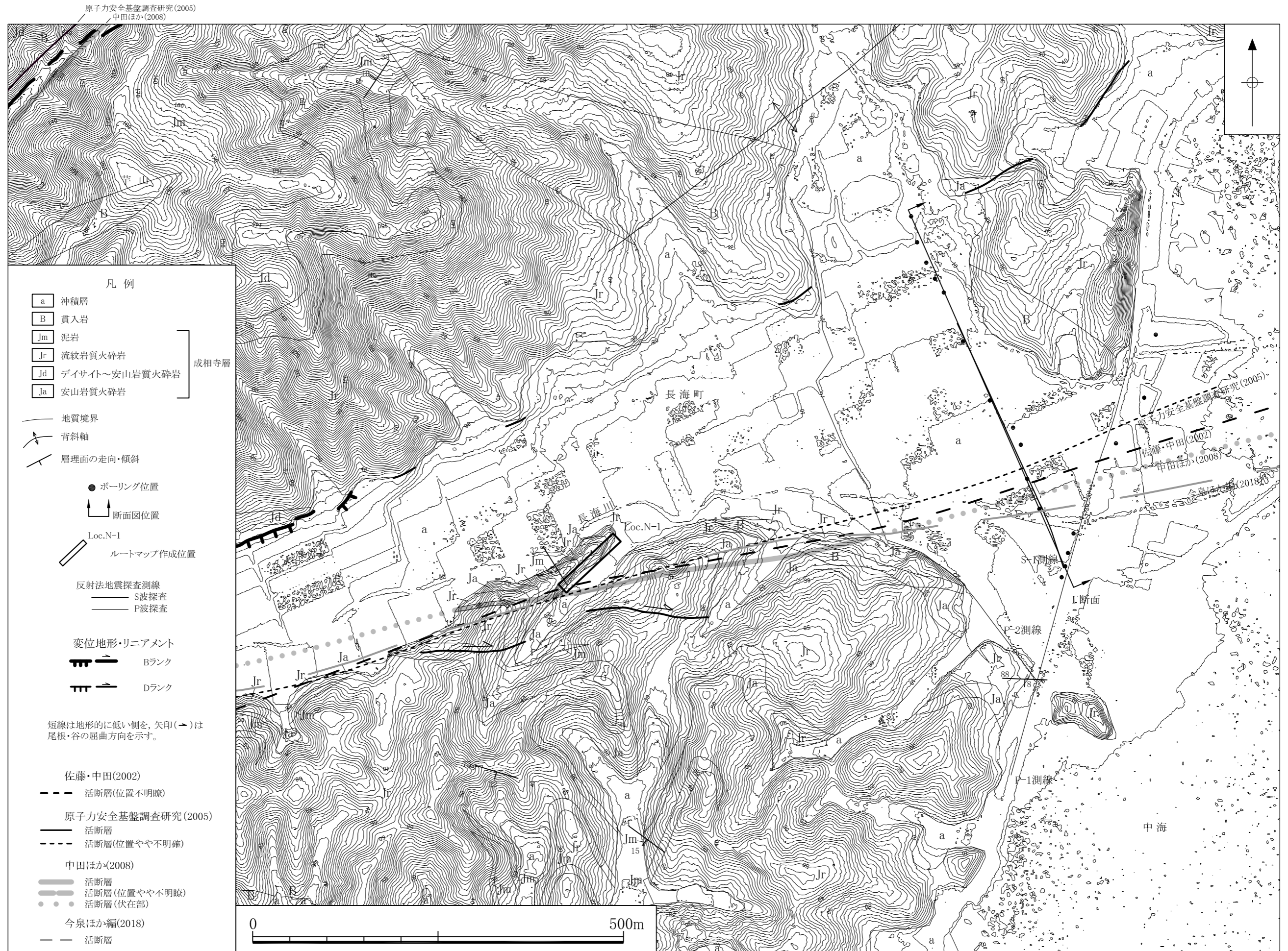
第3.3-41図 長海町地区詳細地質図
