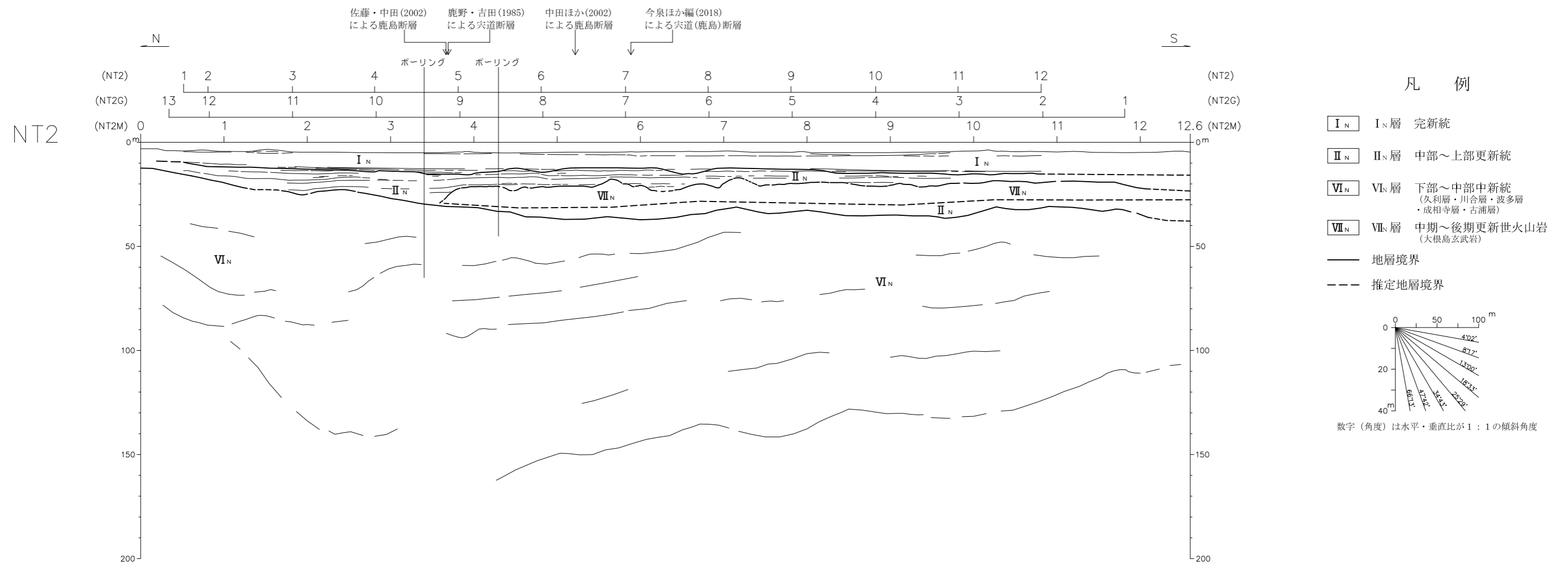
第3.3-45図 中海北部海域の地質断面図
