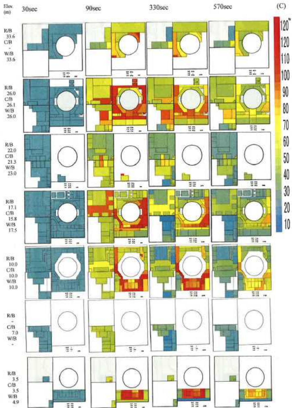
図 4.3-3 区画の可視化の作成例 (例)
