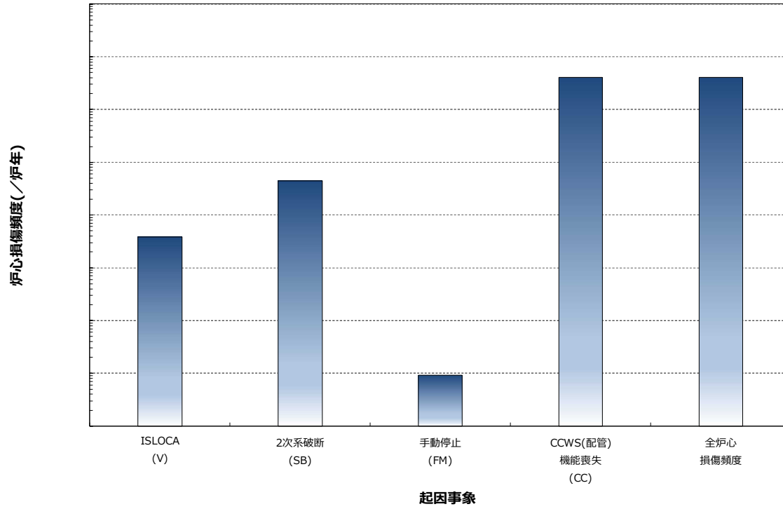
図 4.4-1 起因事象別炉心損傷頻度の割合(例)
