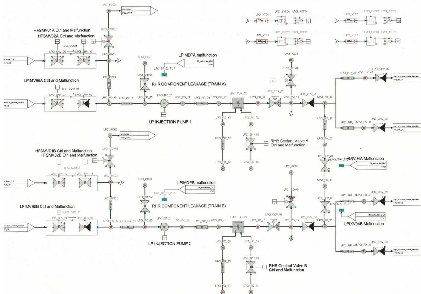
図 4.2-1 余熱除去系 (RHR 系) のモデル図 (例)
