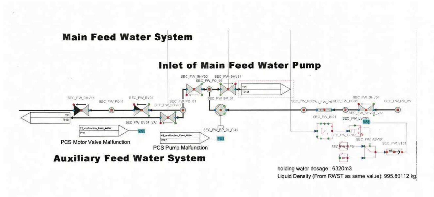
図 4.2-2 主給水系のモデル図 (例)
