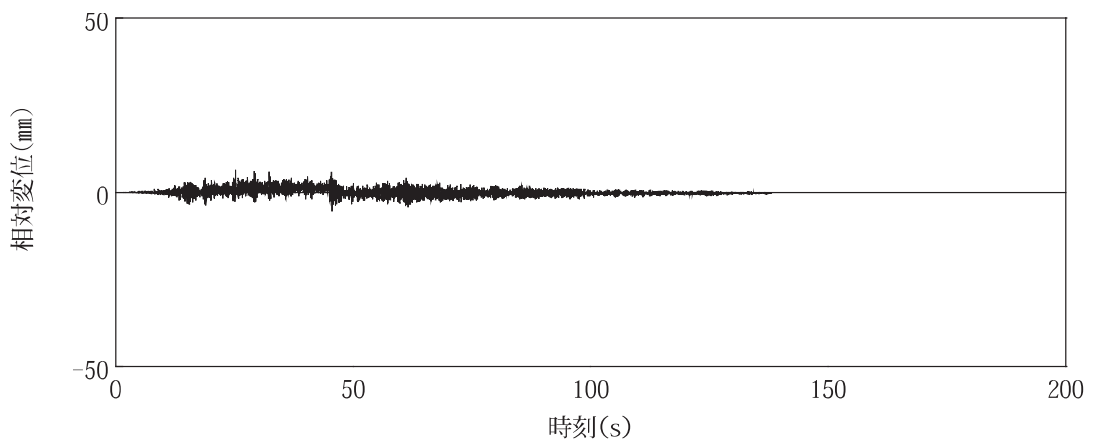
図 4-2 (9) 時刻歴相対変位波形
