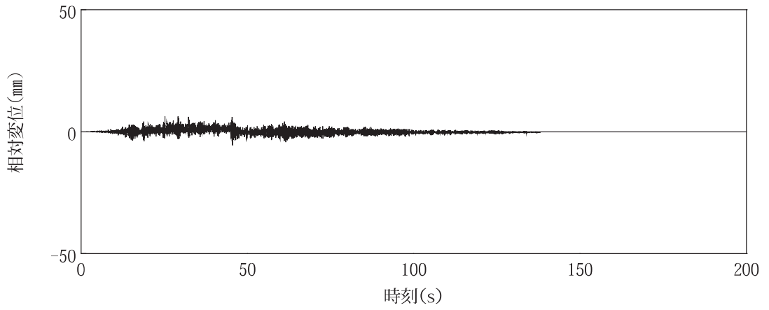
図 4-2 (7) 時刻歴相対変位波形
