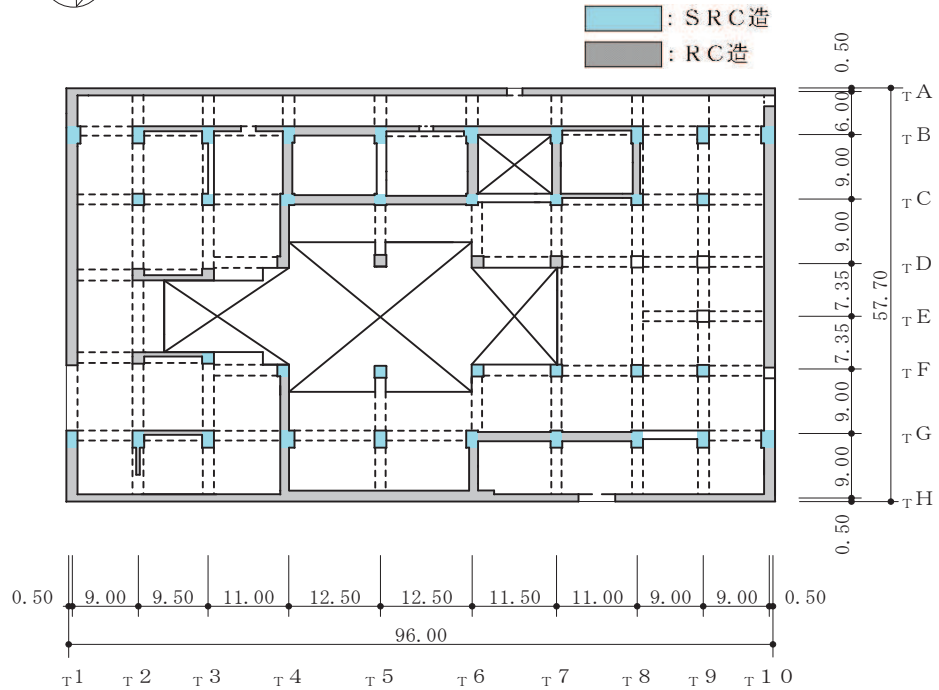
図 2-2(3) タービン建屋の概略平面図 (O.P. 15.0m)
