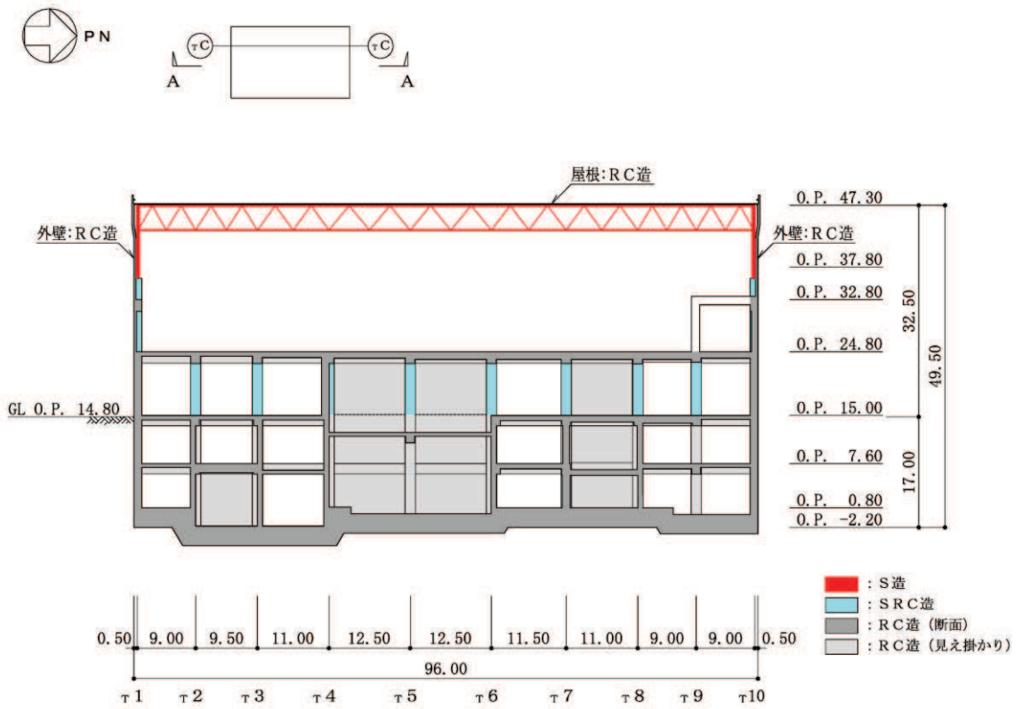
図 2-3(1) タービン建屋の概略断面図 (A-A 断面, NS 方向)
