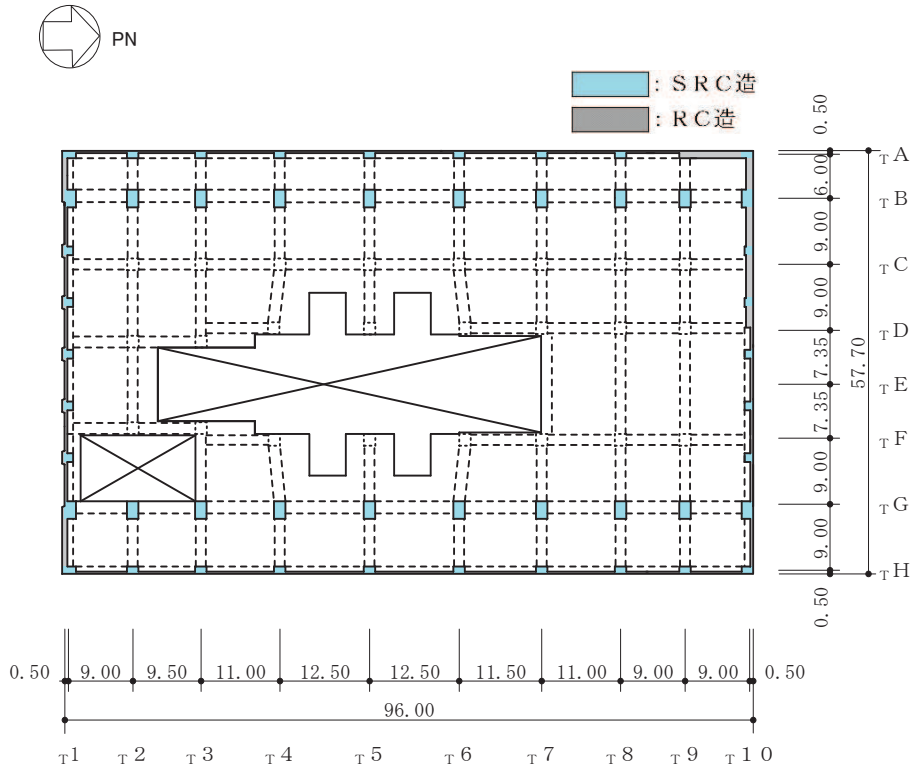
図 2-2(4) タービン建屋の概略平面図 (O.P. 24.8m)
