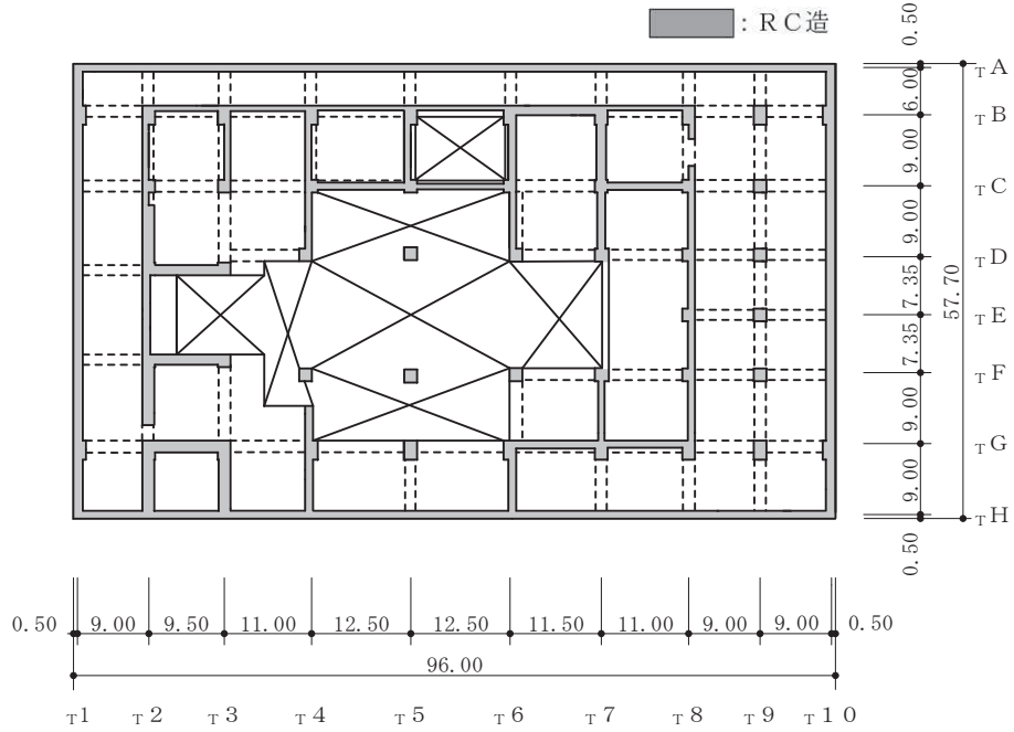
図 2-2(2) タービン建屋の概略平面図 (O.P. 7.6m)
