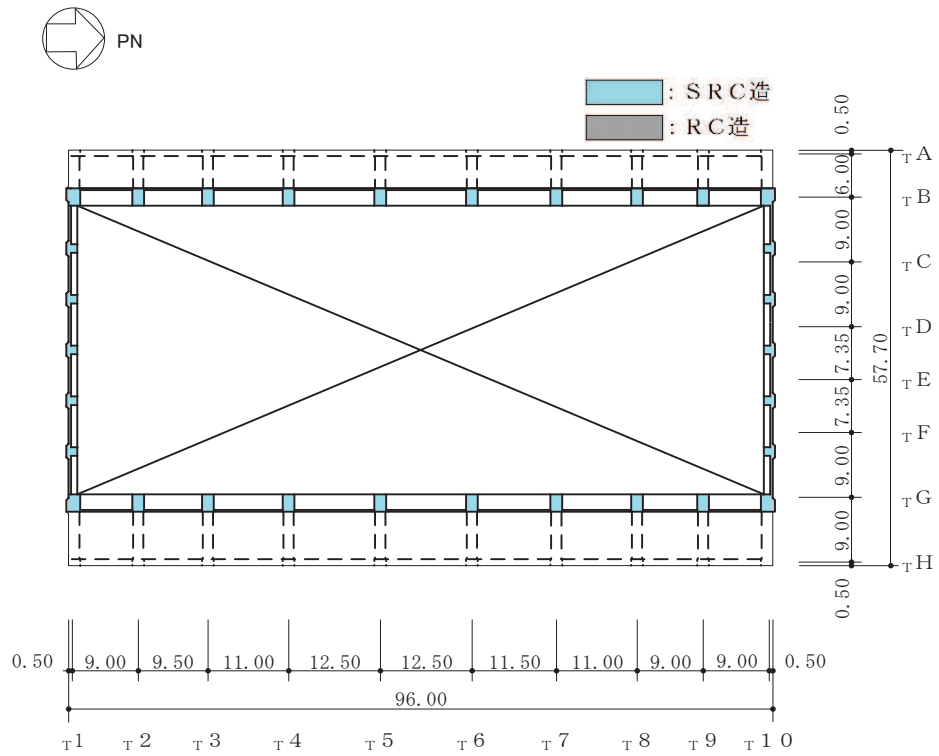
図 2-2(5) タービン建屋の概略平面図 (O.P. 32.8m)
