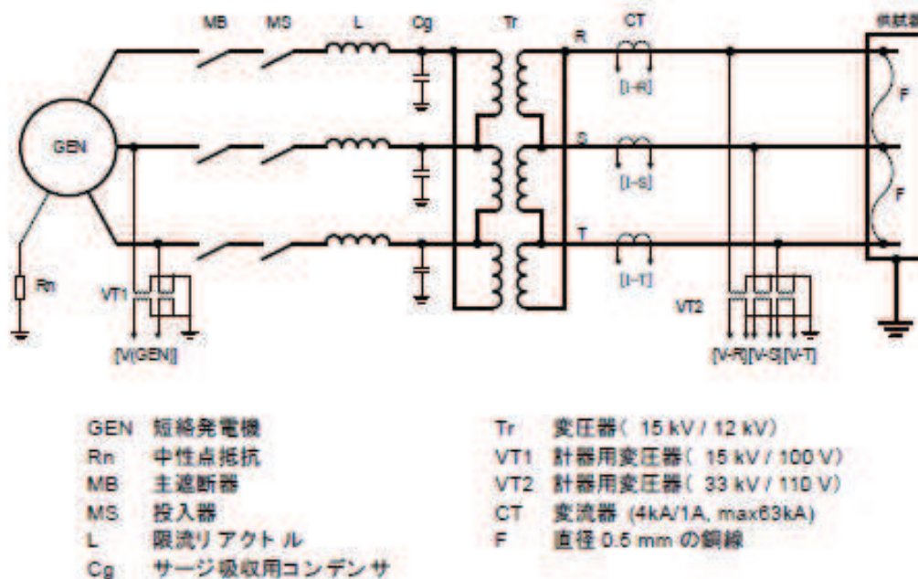
図 4.3.1 M/C 試験回路
