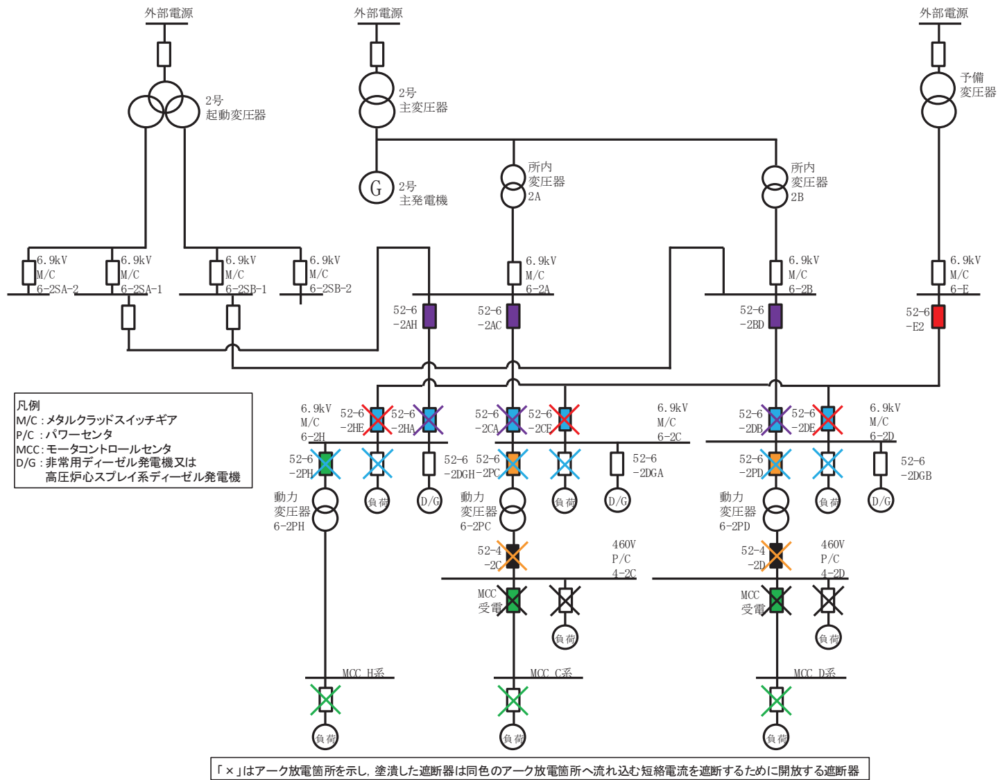
図 3. 3 HEAF 対策が必要な電気盤系統図 (1/2) (非常用ディーゼル発電機又は高圧炉心スプレイ系ディーゼル発電機からの給電時以外)
