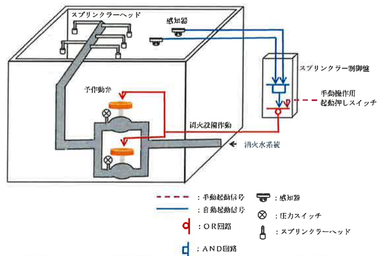
第5-1図 スプリンクラーの概要
