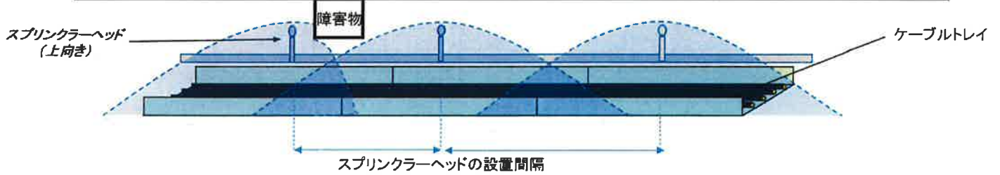
障害物がある場合のスプリンクラーヘッド配置例
