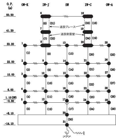
図 4-14(2) 曲げスケルトンカーブ上の最大応答値 (基準地震動 S s , NS 方向) (2/6)
