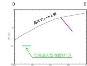
断層配置図(断面)
