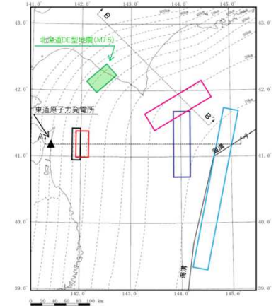
断層配置図(平面)
