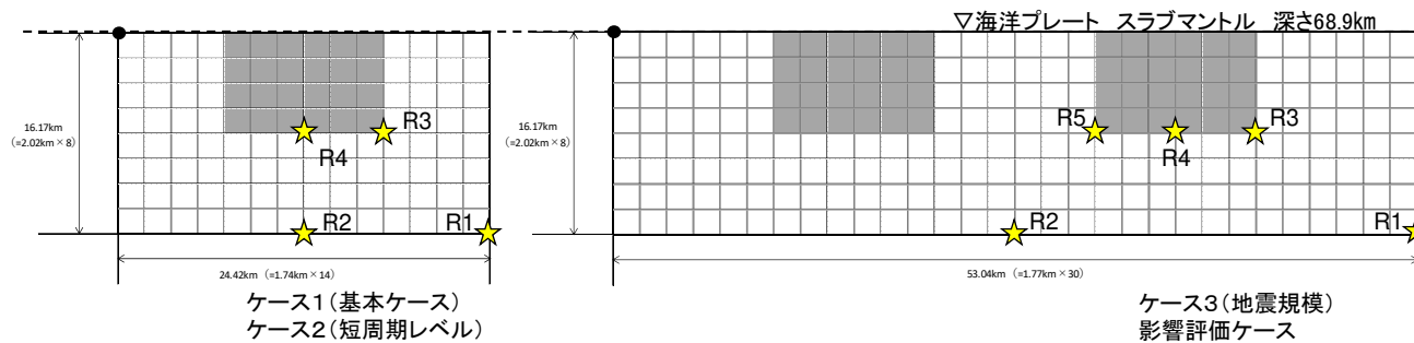
敷地下方DC型地震 展開図
