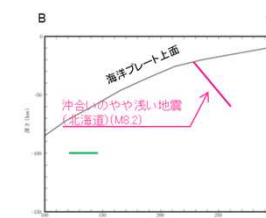
断層配置図(断面)
