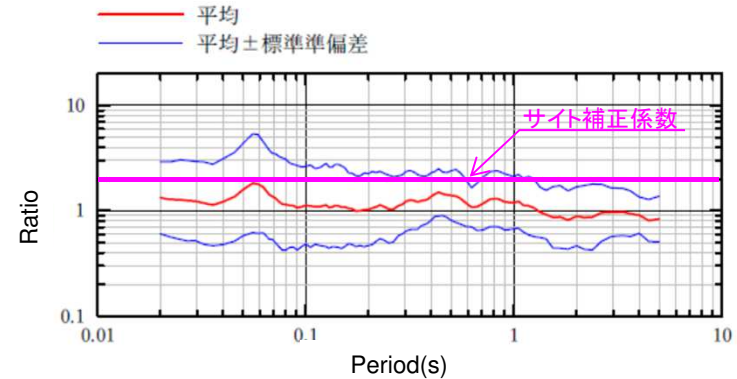
鉛直成分
