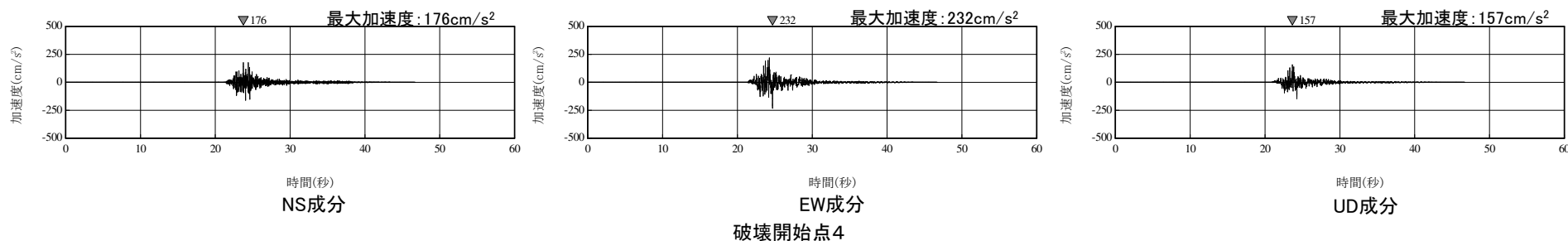
敷地下方DC型地震のうちケース1(基本ケース)の加速度波形(PN基準)
