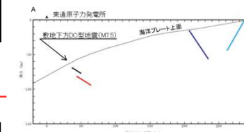
断層配置図(断面)
