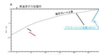
断層配置図(断面)
