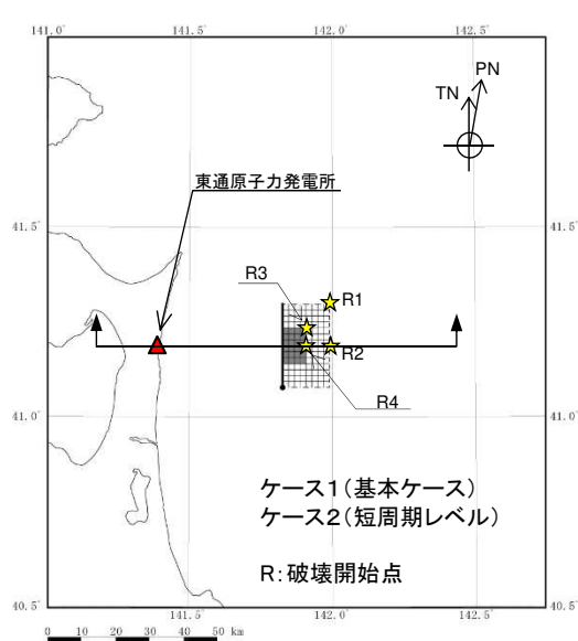
断層配置図
