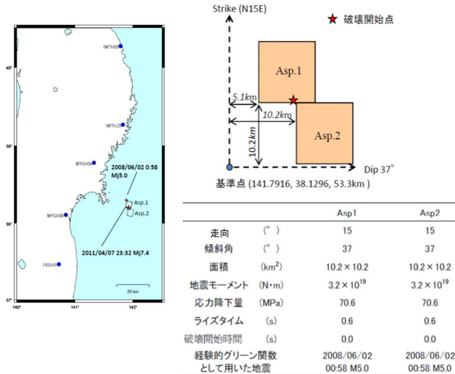
原田・釜江(2011)の4.7地震の震源モデル
