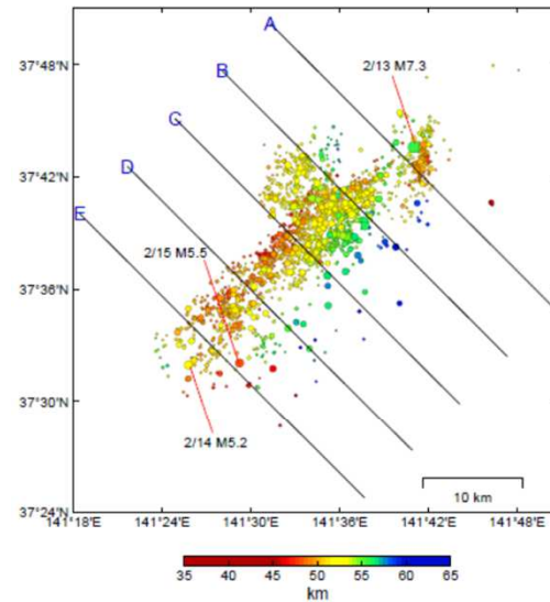
震央分布
