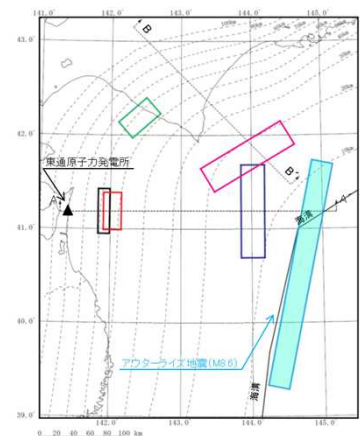
断層配置図(平面)
