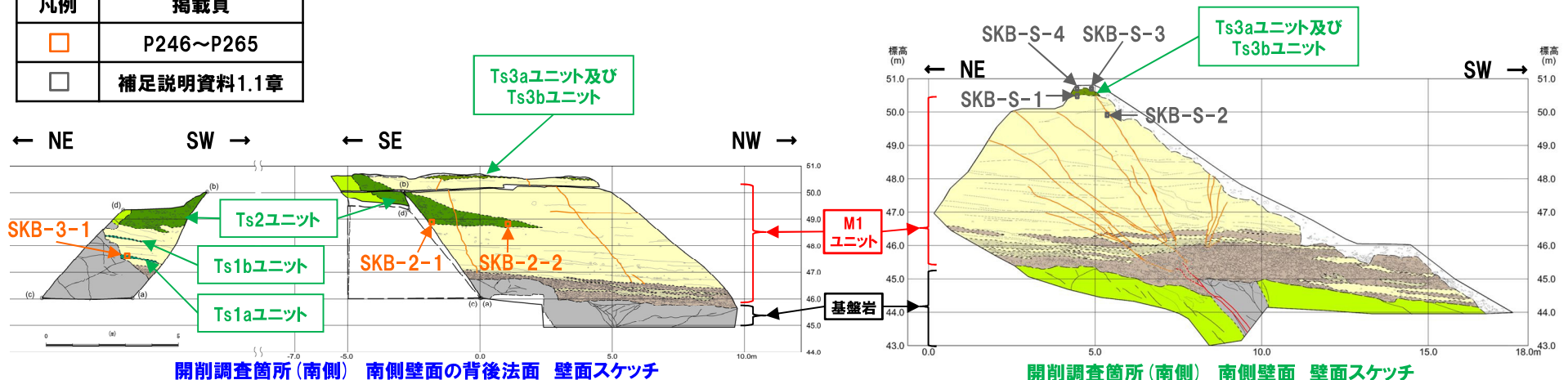
開削調査箇所(南側) 南側壁面の背後法面 壁面スケッチ
