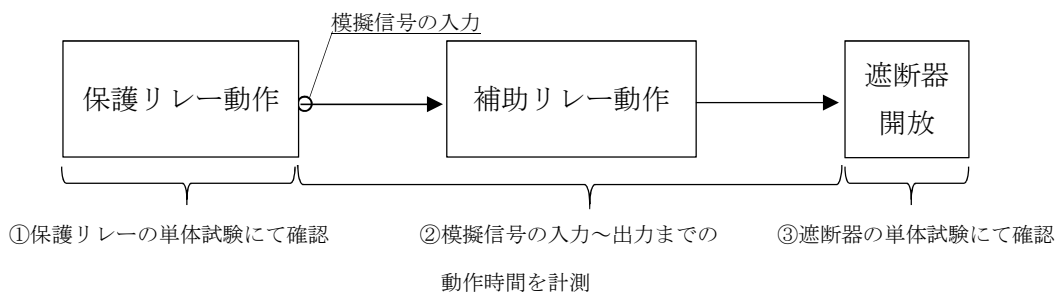
図 4-1 パターン1（M/C に接続される遮断器（D/G 受電遮断器以外）での HEAF 時）
