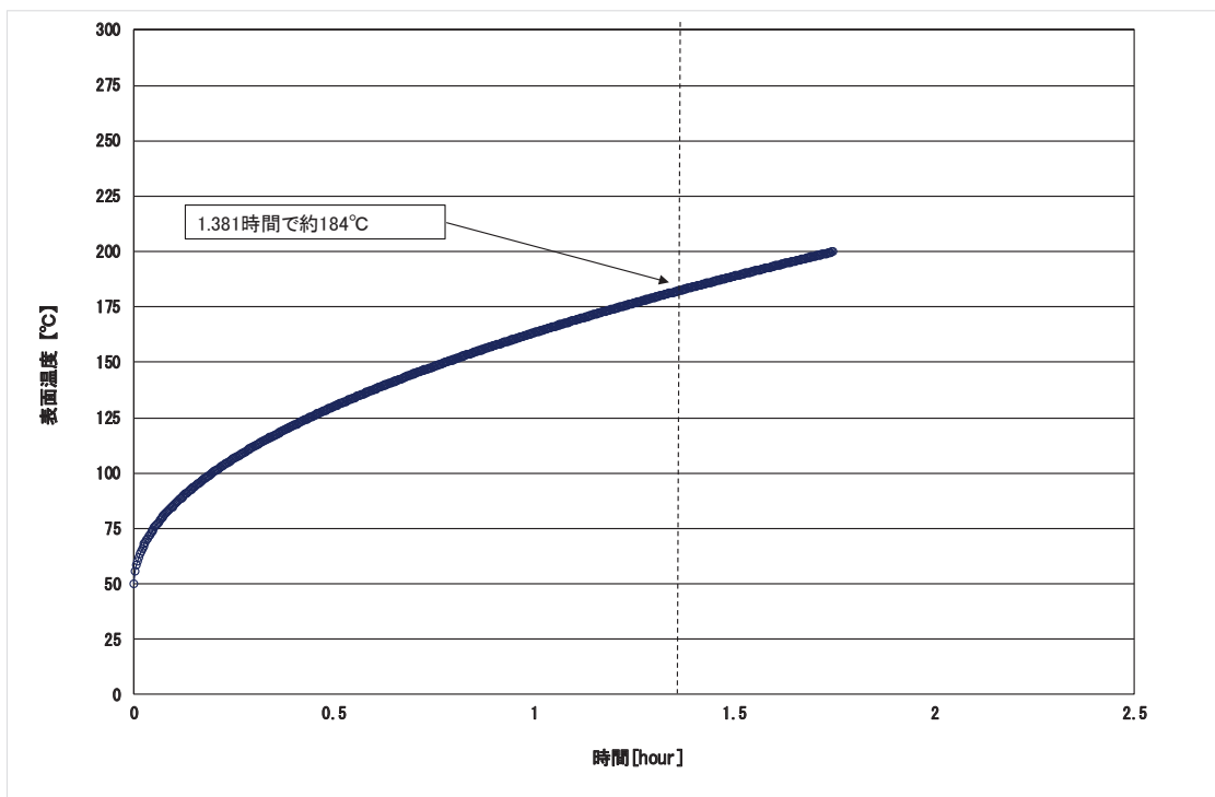
図 2.3-6 外壁温度推移（自衛隊機又は米軍機（その他の大型固定翼機，小型固定翼機及び回転翼機））
