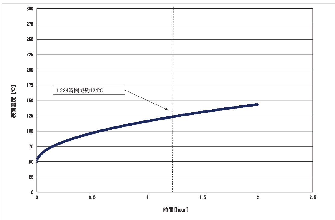
図 2.3-7 外壁温度推移（自衛隊機又は米軍機（基地—訓練空域間往復時））
