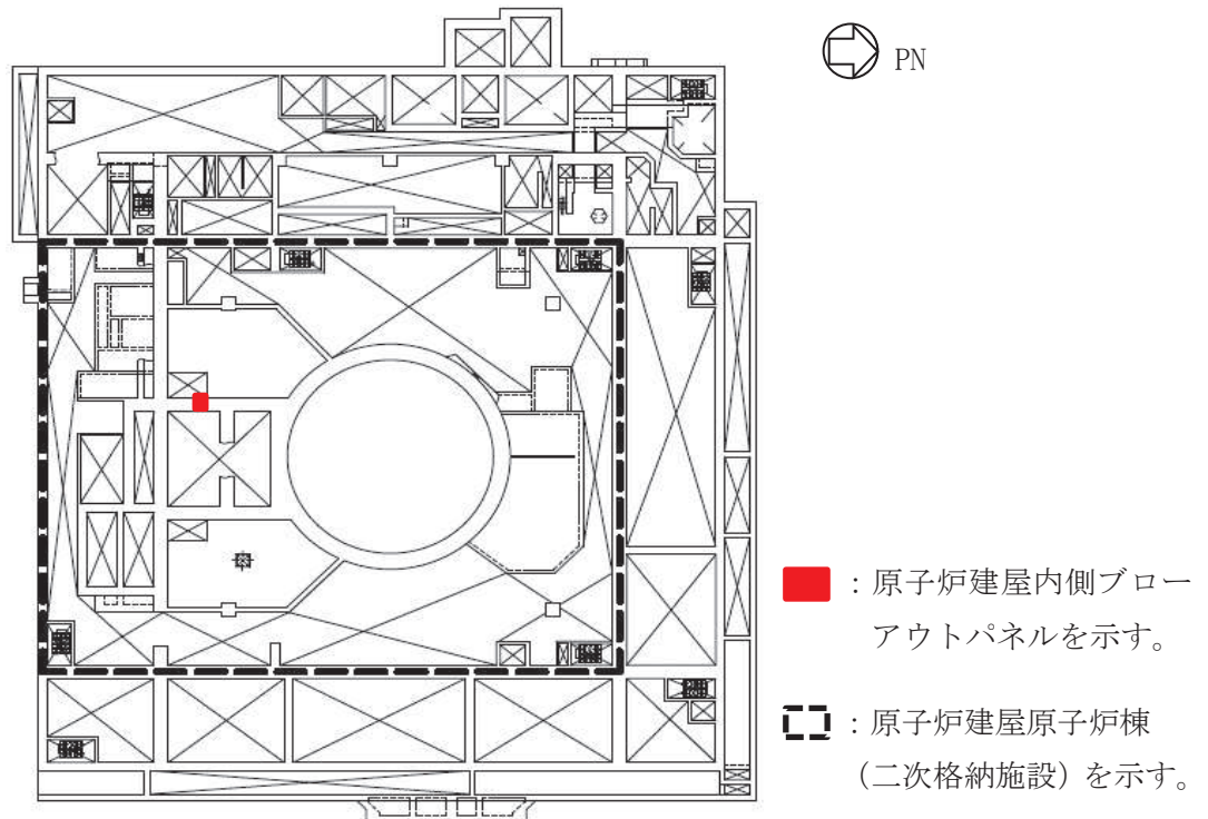
原子炉建屋原子炉棟中地下 1 階 概略平面図
