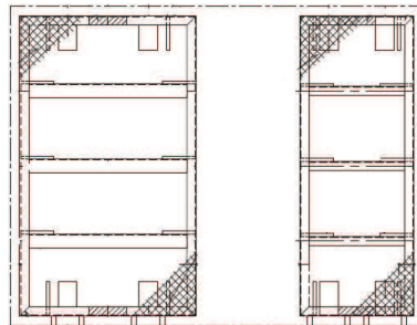
正面図
