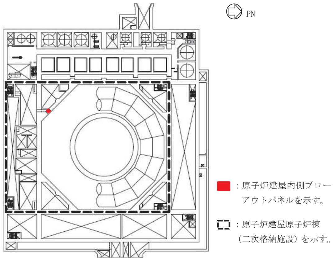
原子炉建屋原子炉棟中地下3階 概略平面図
