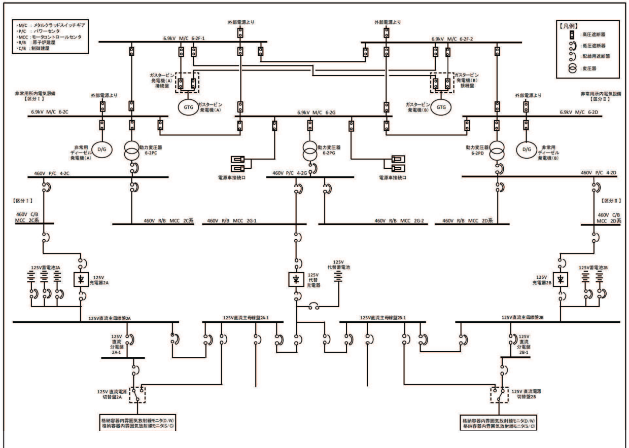
【格納容器内雰囲気放射線モニタの電源構成概略図】
