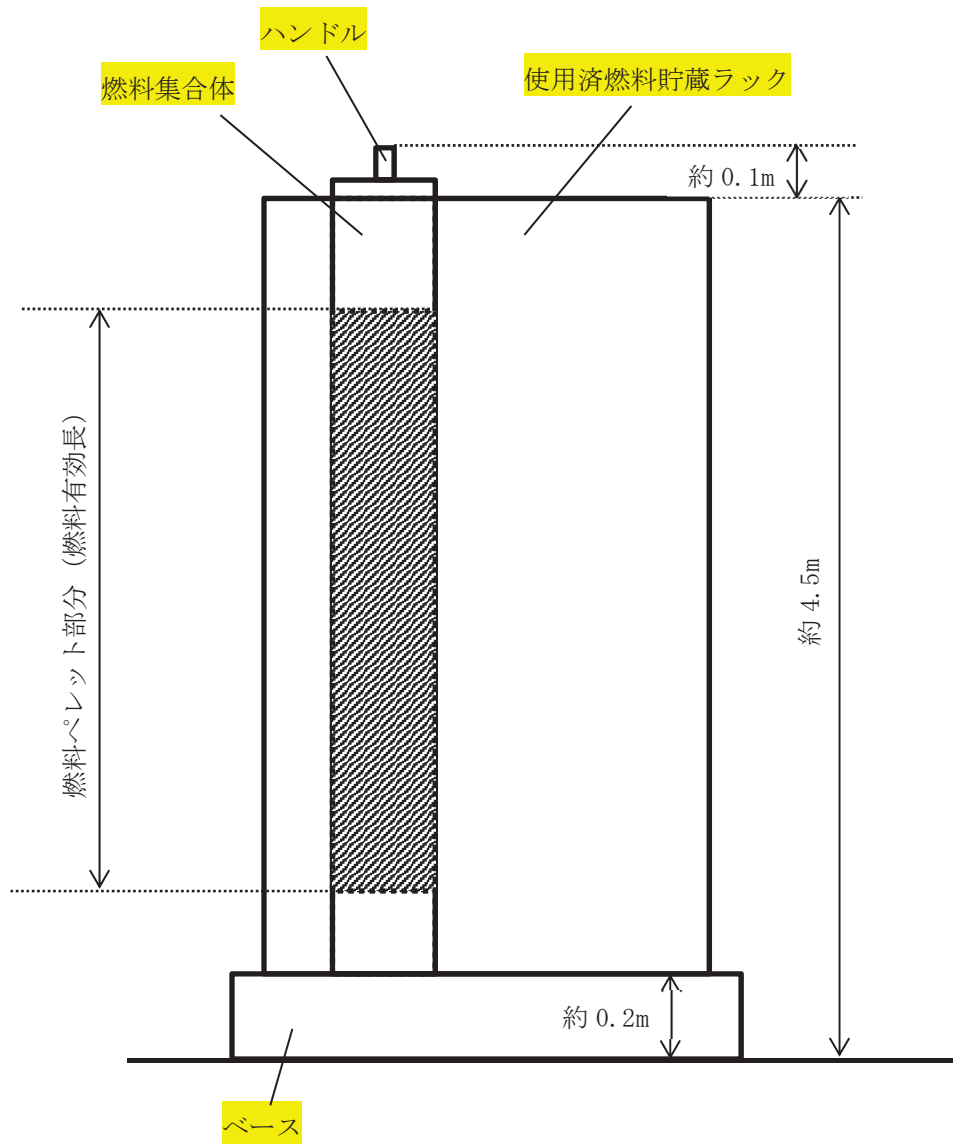
図 5-3 燃料集合体とラックの関係図
