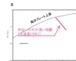
断層配置図(断面)
