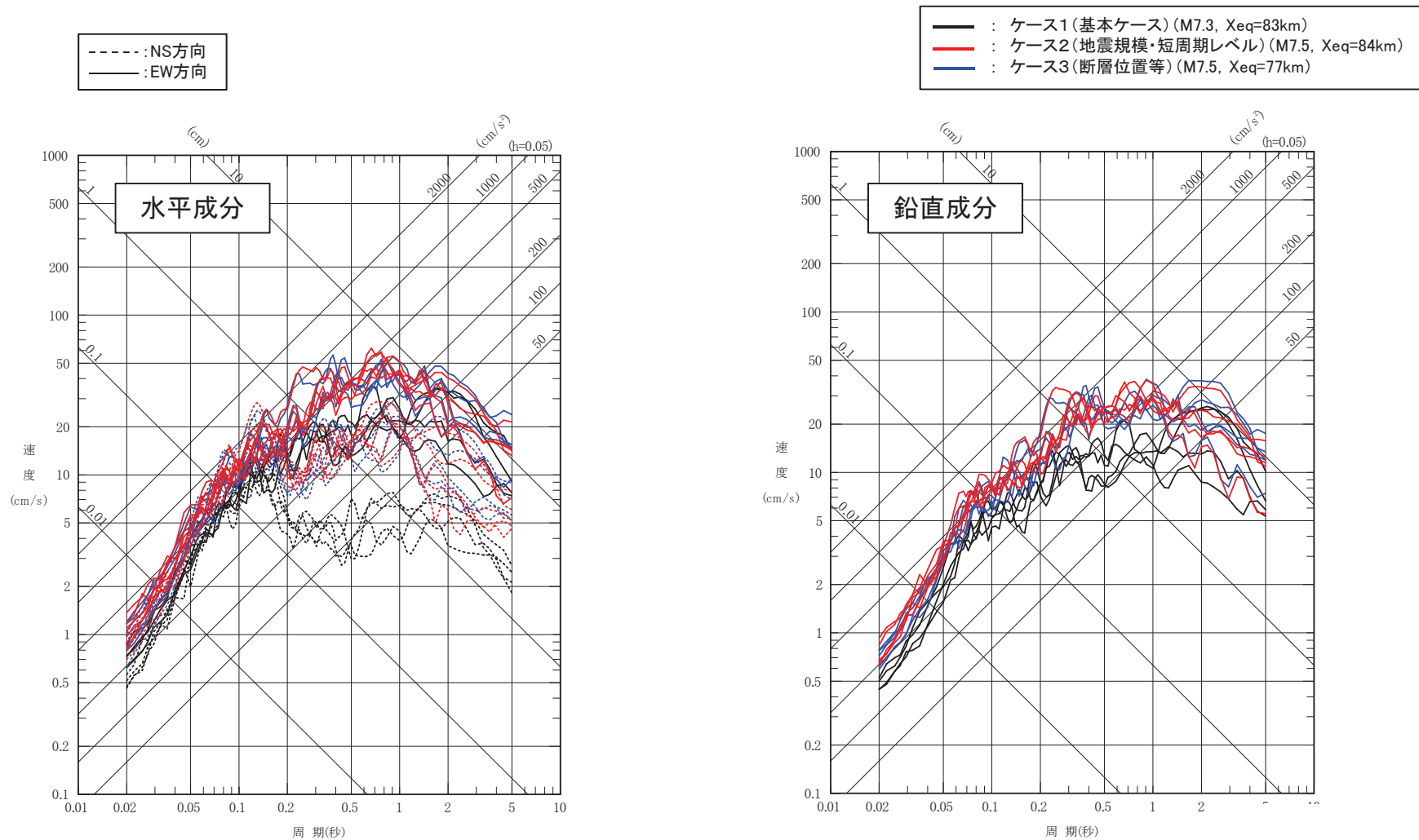
敷地下方DC型地震の断層モデル手法を用いた地震動評価(PN基準)
