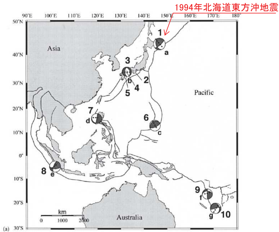
規模の大きな浅い海洋プレート内地震の震源メカニズム 〔Seno and Yoshida(2004)一部加筆〕
