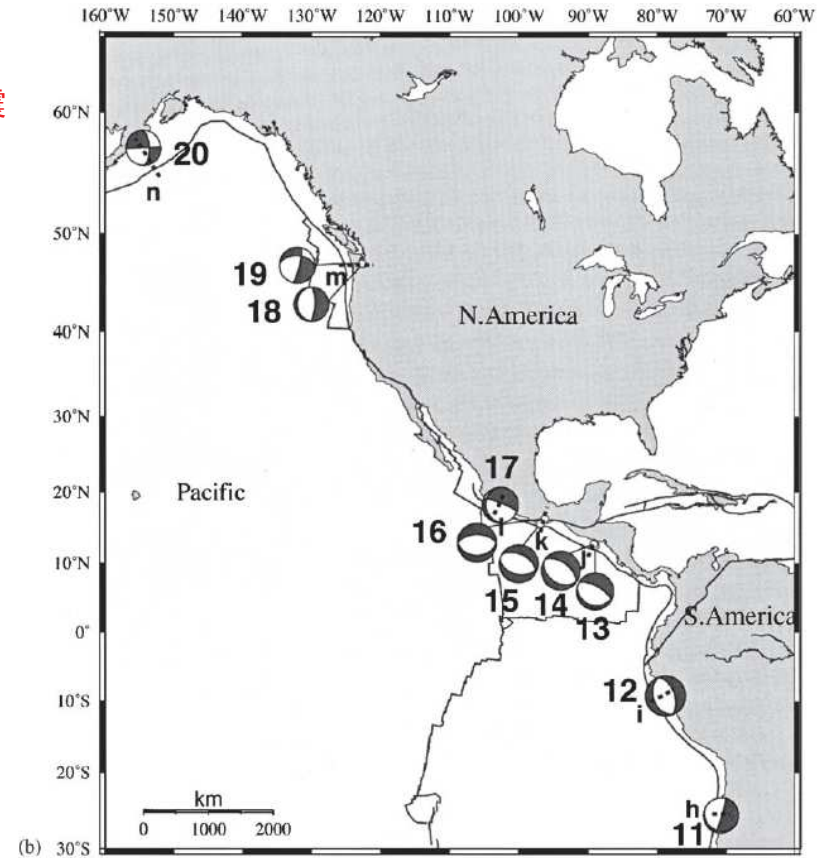
規模の大きな浅い海洋プレート内地震の震源メカニズム 〔Seno and Yoshida(2004)一部加筆〕
