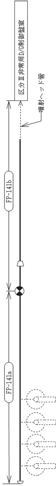
区分Ⅲ非常用D/G制御室消火系 ハロン130L貯蔵容器
