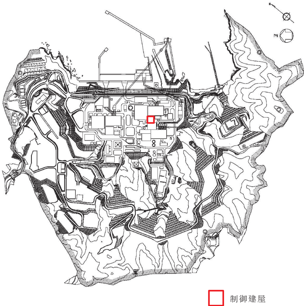
図 2-1 中央制御室待避所遮蔽を含む制御建屋の設置位置
