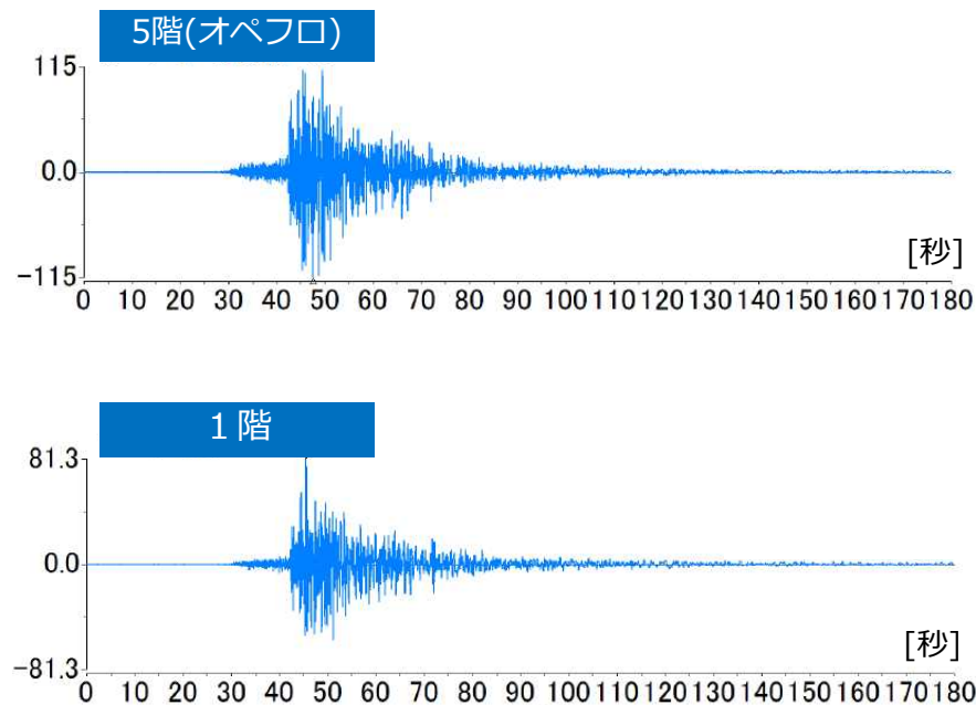
3号機地震計 2021年3月20日の観測記録 (NS方向)
