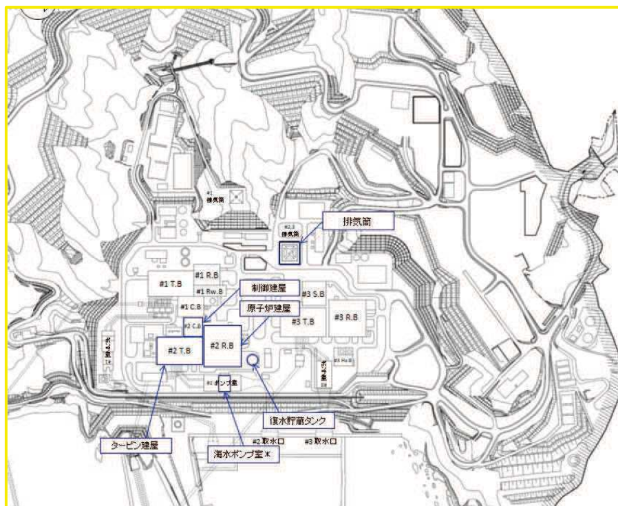
(敷地全体図)
