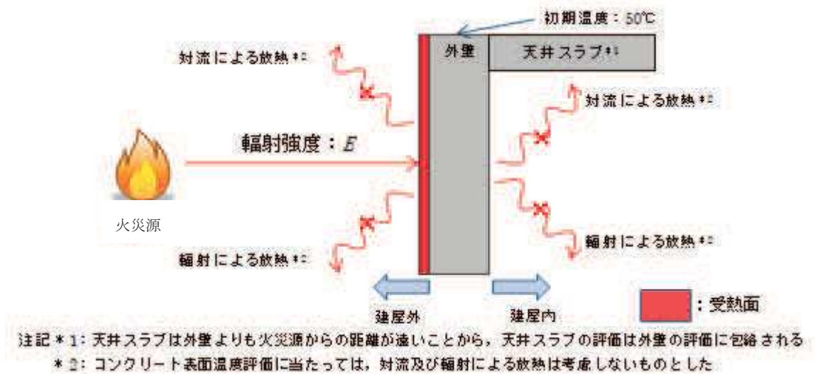
図 2.3-2 建屋外壁の評価概念図
