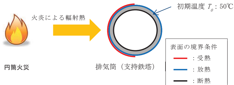
図 2.3-9 排気筒の評価概念図
