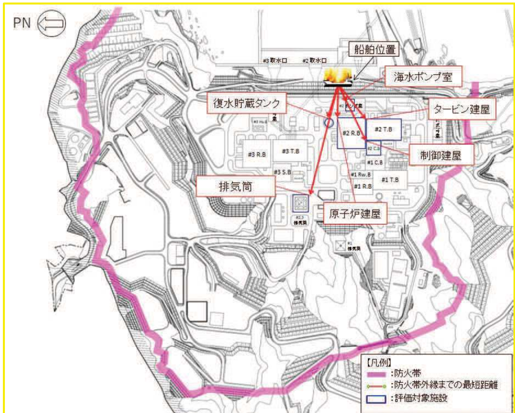
(敷地全体図)
