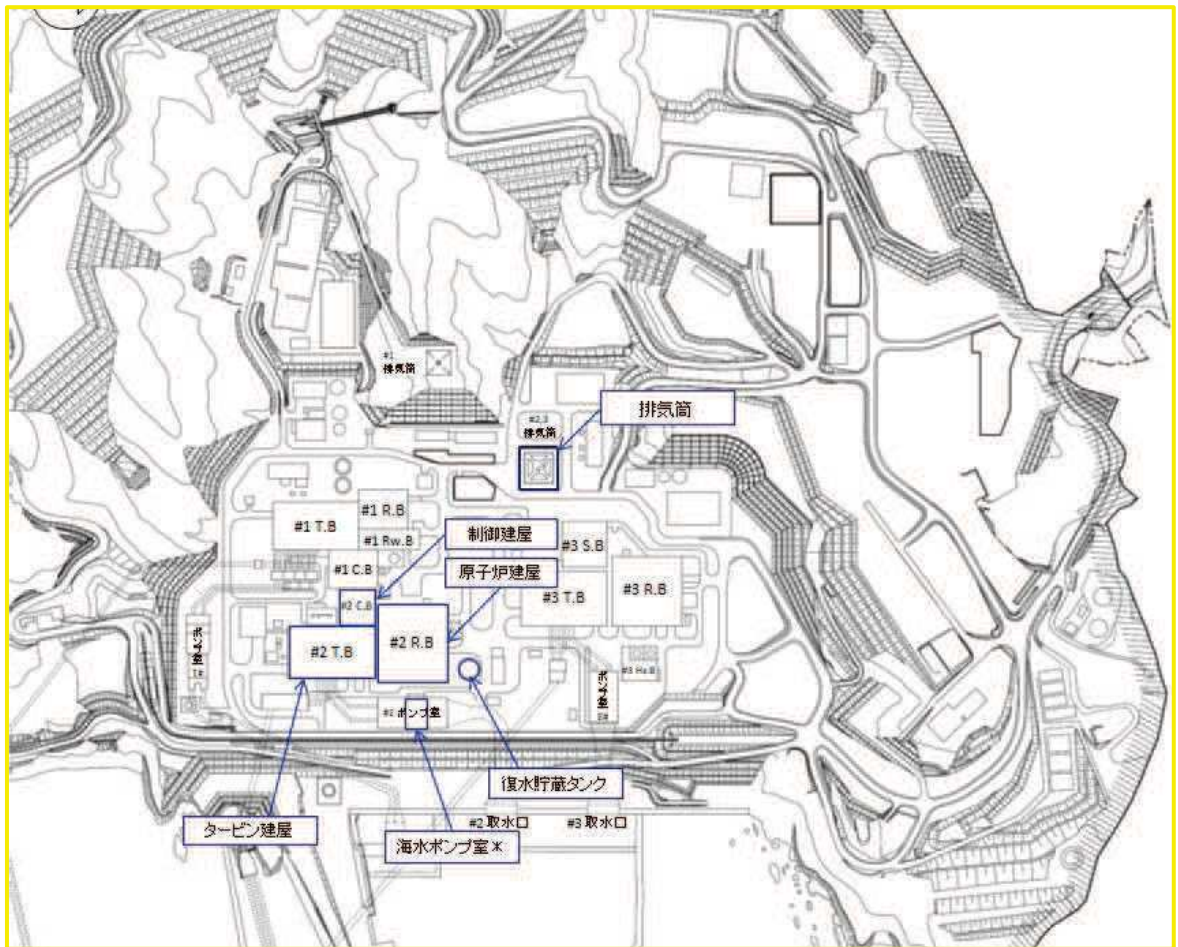
(敷地全体図)
