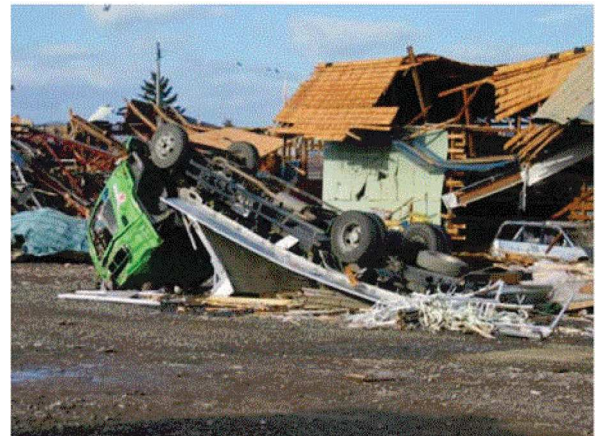
図37 竜巻による被災後の4tトラックの様子 (26)(30)
