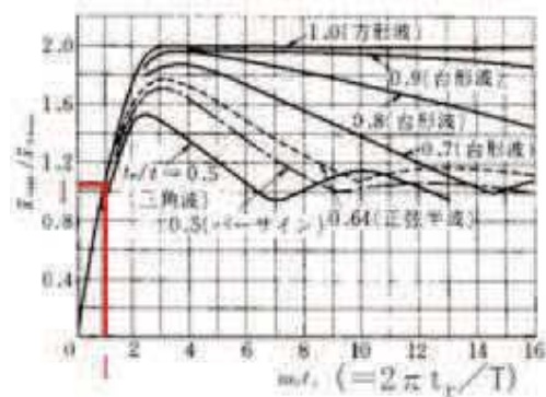
図 1.5-2 衝突時間と応答加速度の関係 (機械工学便覧(基礎編α2 機械力学))
