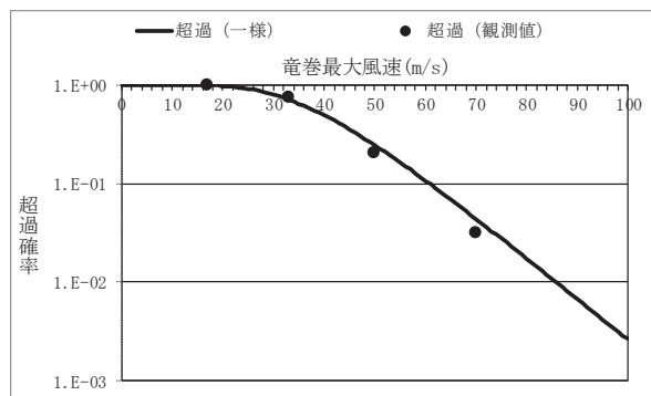
図 1.9-27 竜巻最大風速の超過確率分布
