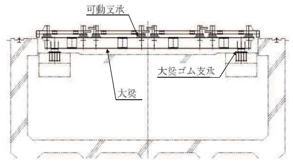
(B-B 矢視)
