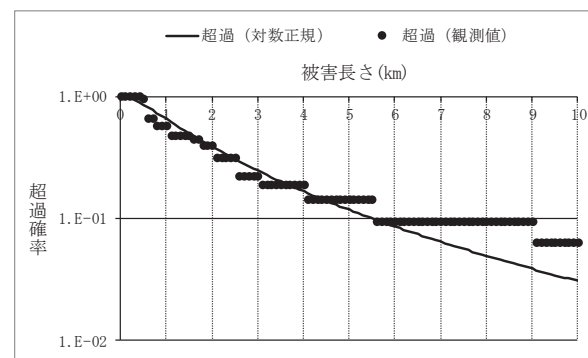
図 1.9-31 被害長さの超過確率分布
