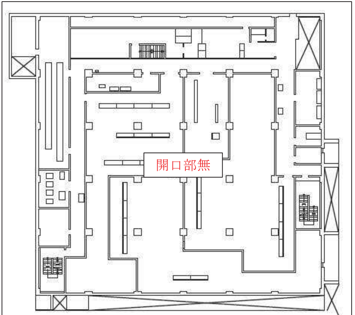
図 1.3-11 制御建屋 0.P. 19.50m における開口部
