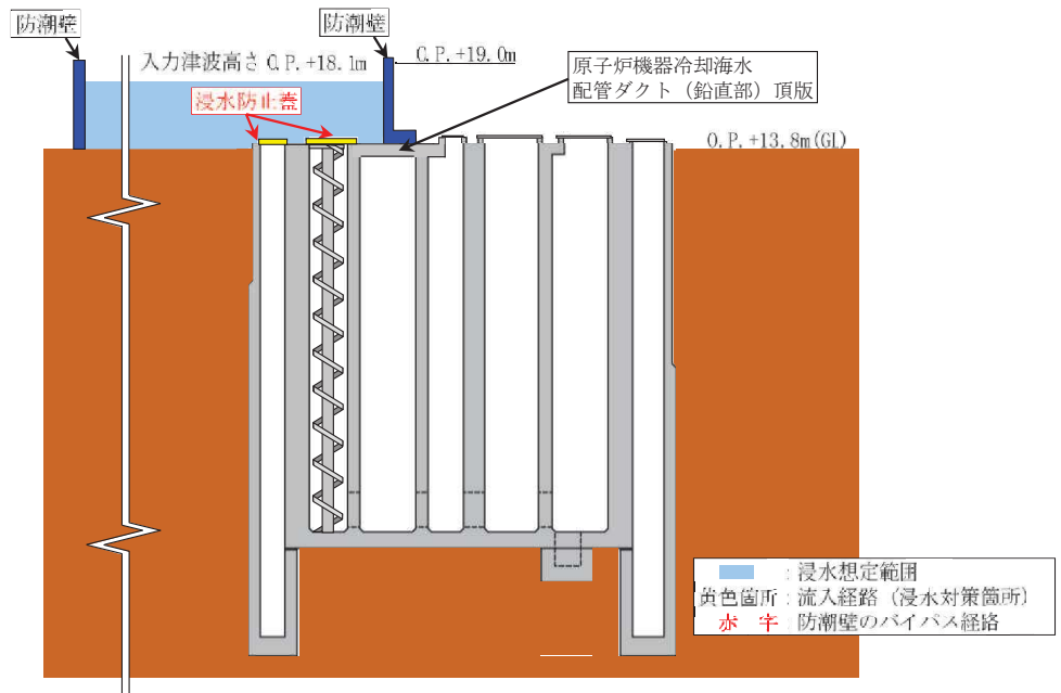
第2号機海水ポンプ室 (B-B断面図)
