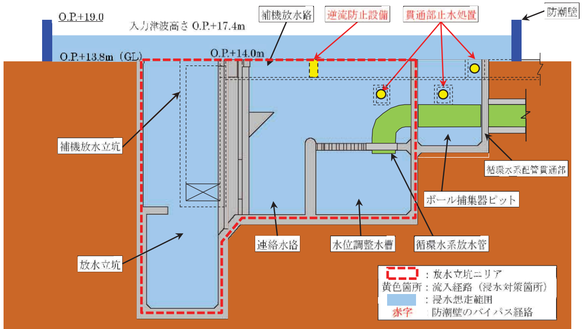
図 2.1-1 強度評価の対象施設の配置 (12/18)
