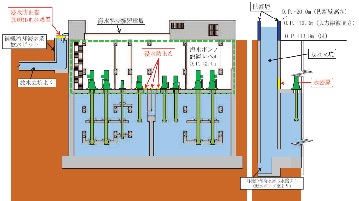
第3号機海水熱交換器建屋 (A-A, B-B 断面図)
