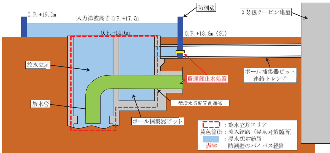
第3号機放水立坑（A-A 断面図）
