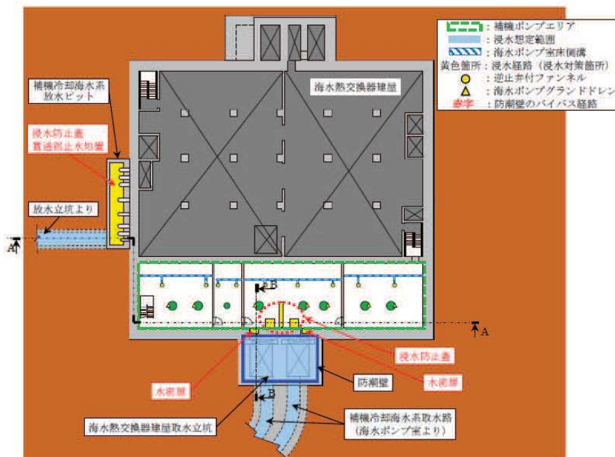
第 3 号機海水熱交換器建屋 (平面図)
