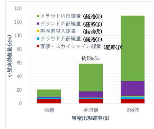
敷地境界における実効線量の評価結果 (高浜 3、4 号機の評価例：格納容器健全)
