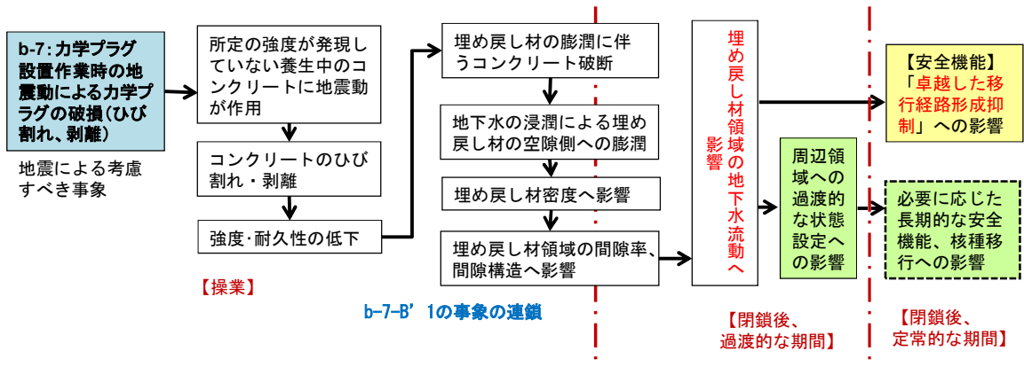
図 3.2-66 操業段階における力学プラグ設置作業時の地震動による力学プラグの破損による埋め戻し材の特性や安全機能への影響(b-7-B'1)
