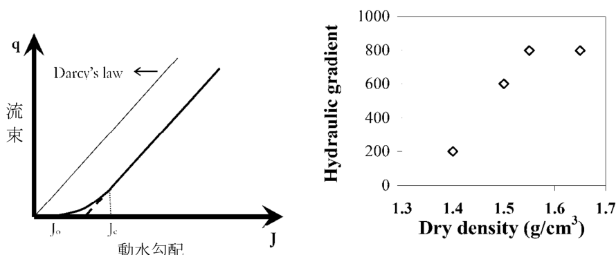
図 4.3-15 Dixon et al. (33) による非線形流動モデルの概念（左）及び FEBEX ベントナイトを対象とした測定可能な流動開始の動水勾配についての試験結果（右） (32)
