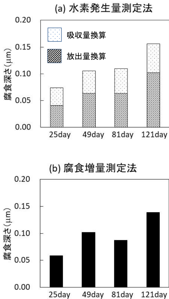
図 2.3-5 (a) 水素発生量測定法と、(b) 腐食増量測定法による 180℃の脱酸素条件でのジルカロイ試料の腐食深さ (腐食量) と時間の関係
