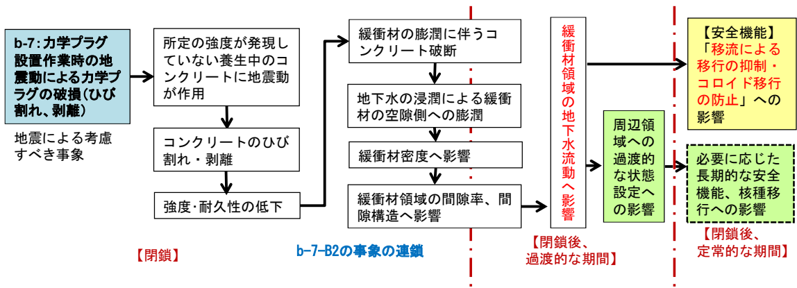
図 3.2-67 閉鎖段階における力学プラグ設置作業時の地震動による力学プラグの破損による緩衝材の特性や安全機能への影響(b-7-B2)
