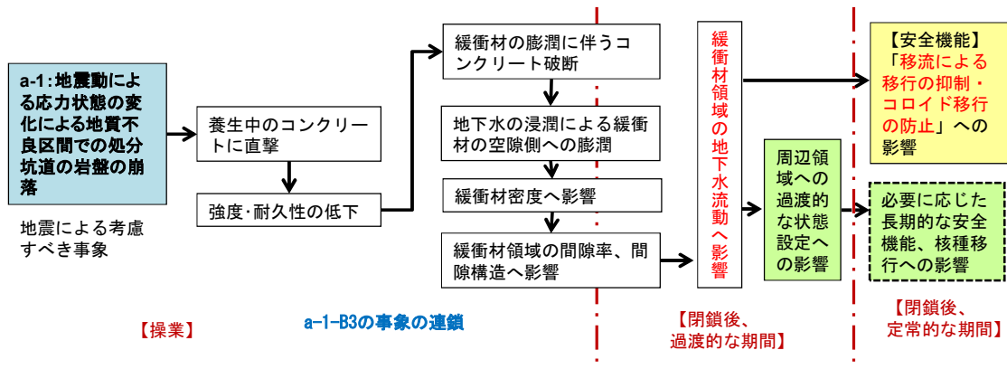
図 3.2-19 作業段階における地質不良区間での処分坑道の岩盤崩落による緩衝材の特性や安全機能への影響(a-1-B3)
