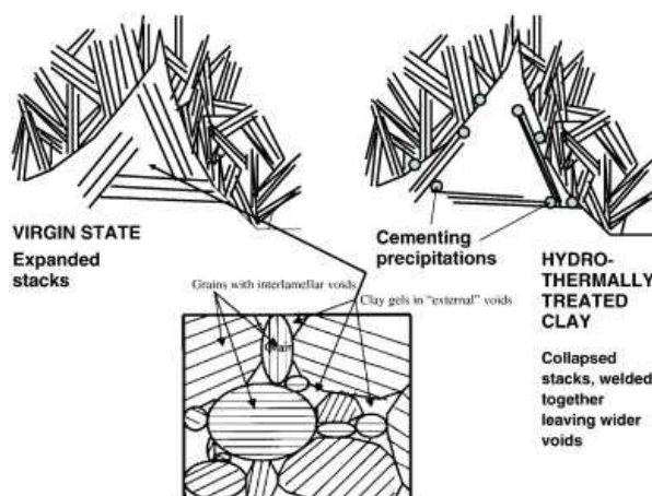
図 4.3-9 加熱による空隙の拡大に伴う透水係数の増大とケイ酸塩鉱物の沈殿に伴う剛性の増大を引き起こすと考えられるメカニズム
