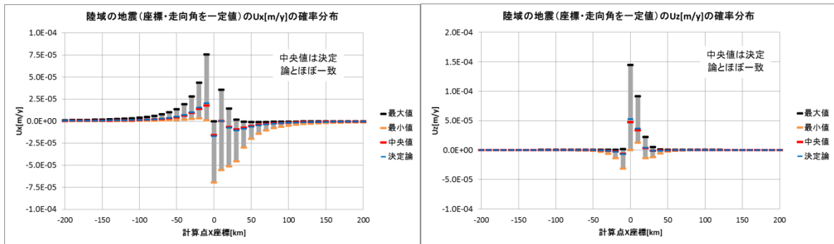
図 1.3-18 陸域の地震による変位速度の確率分布（起点座標と走向角は一定値）
