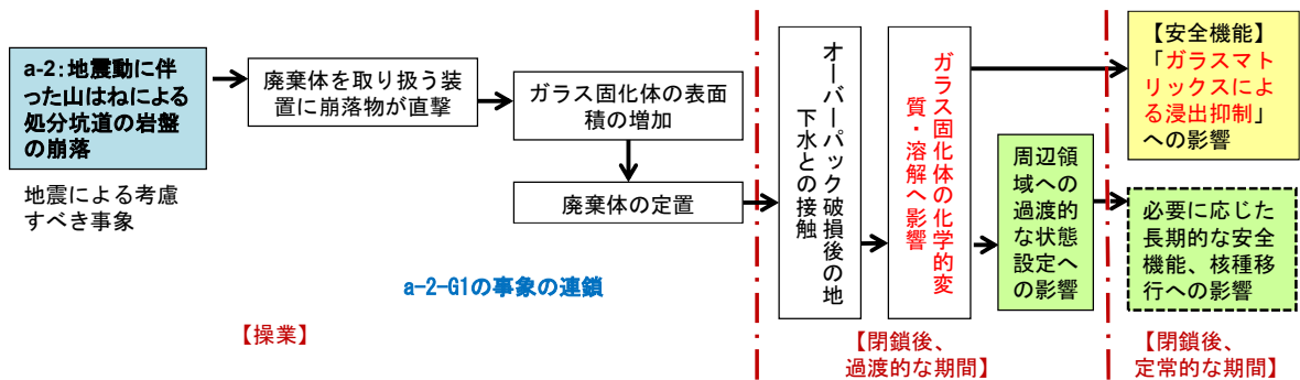
図 3.2-29 建設段階における山はねによる処分坑道の岩盤崩落によるガラス固化体の特性や安全機能への影響(a-2-G1)
