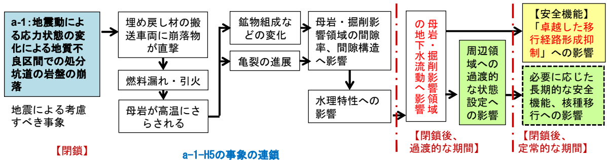
図 3.2-23 閉鎖段階における地質不良区間での処分坑道の岩盤崩落による母岩の特性や安全機能への影響(a-1-H5)
